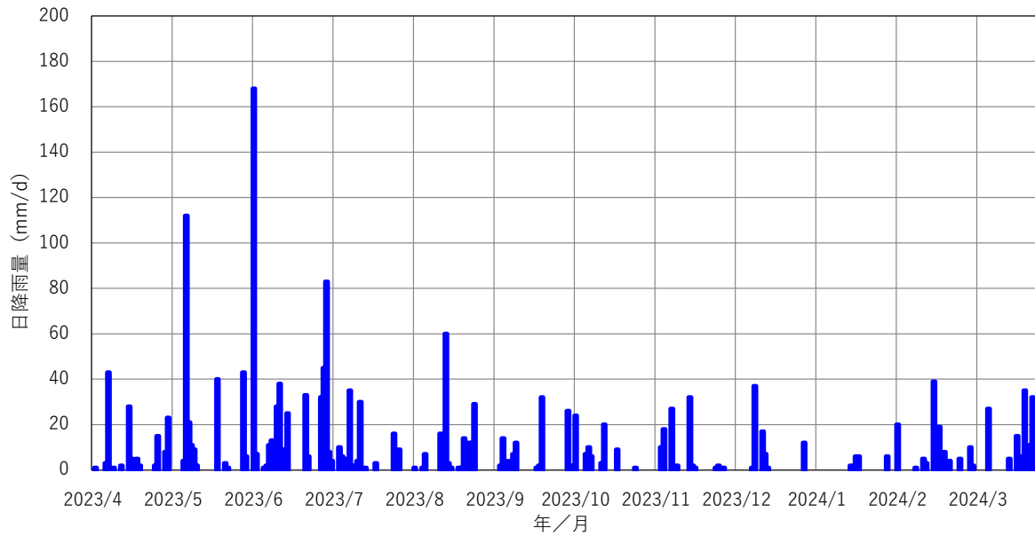
付録1-2 2023年度 日降雨量変動図 (国土交通省・日吉観測所における雨量観測記録 4) より)
