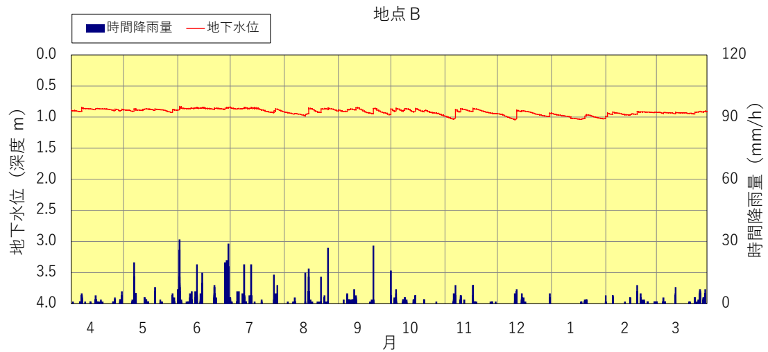
図3.1.2-3 地下水位変動図 地点B (2023年度)
