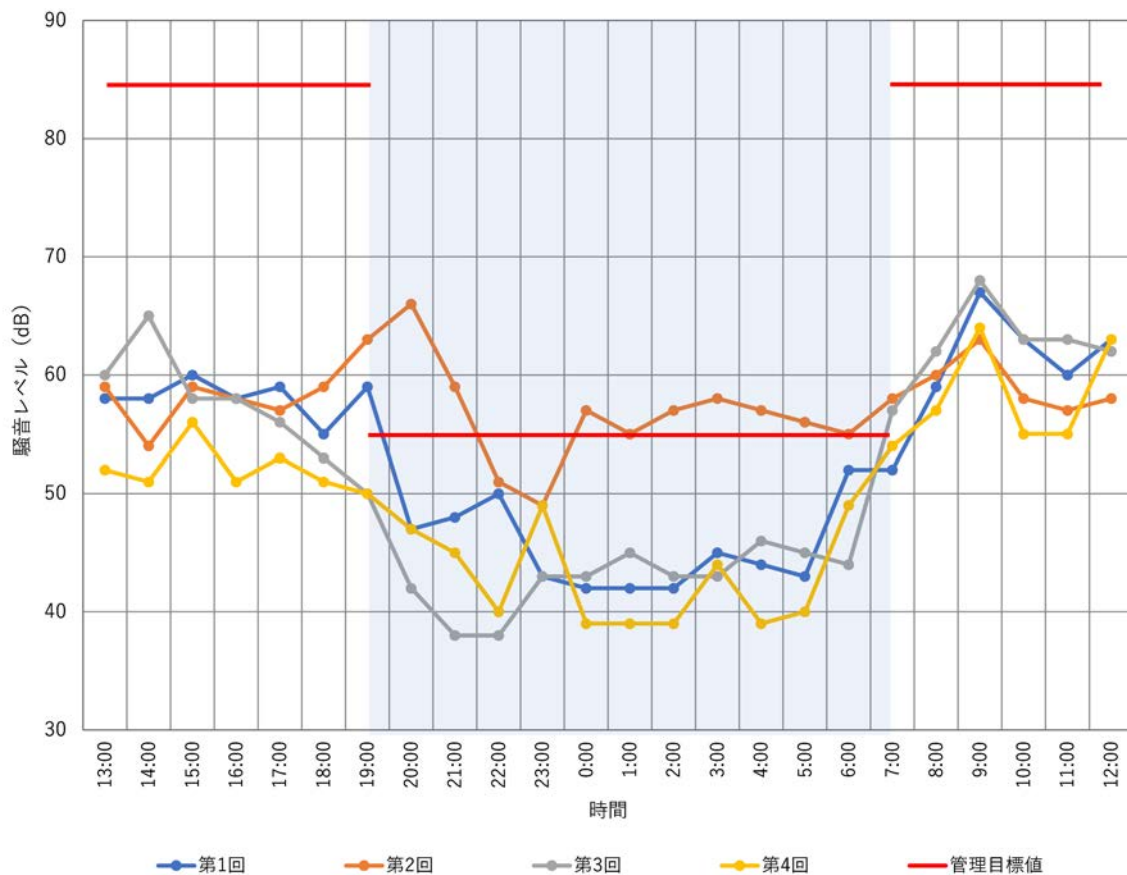
図3.4.2-1 騒音の90%レンジの上端値 (L A5 ) (2023年度)
