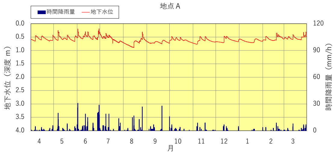
図3.1.2-1 地下水位変動図 地点A (2023年度)
