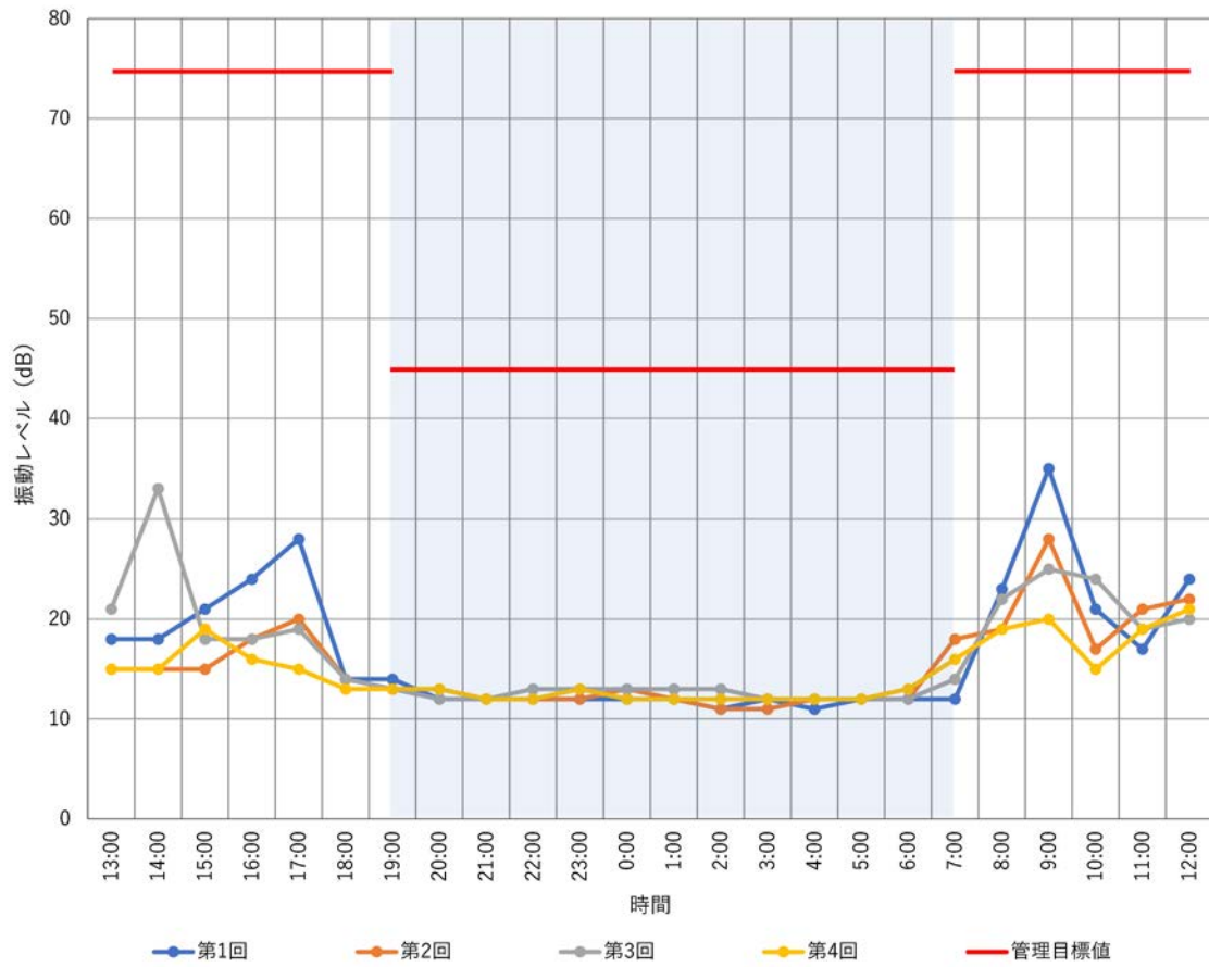
図3.4.2-2 振動の80%レンジの上端値 (L 10 ) (2023年度)
