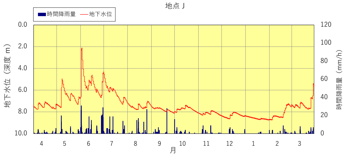
図3.1.2-17 地下水位変動図 地点J (2023年度)
