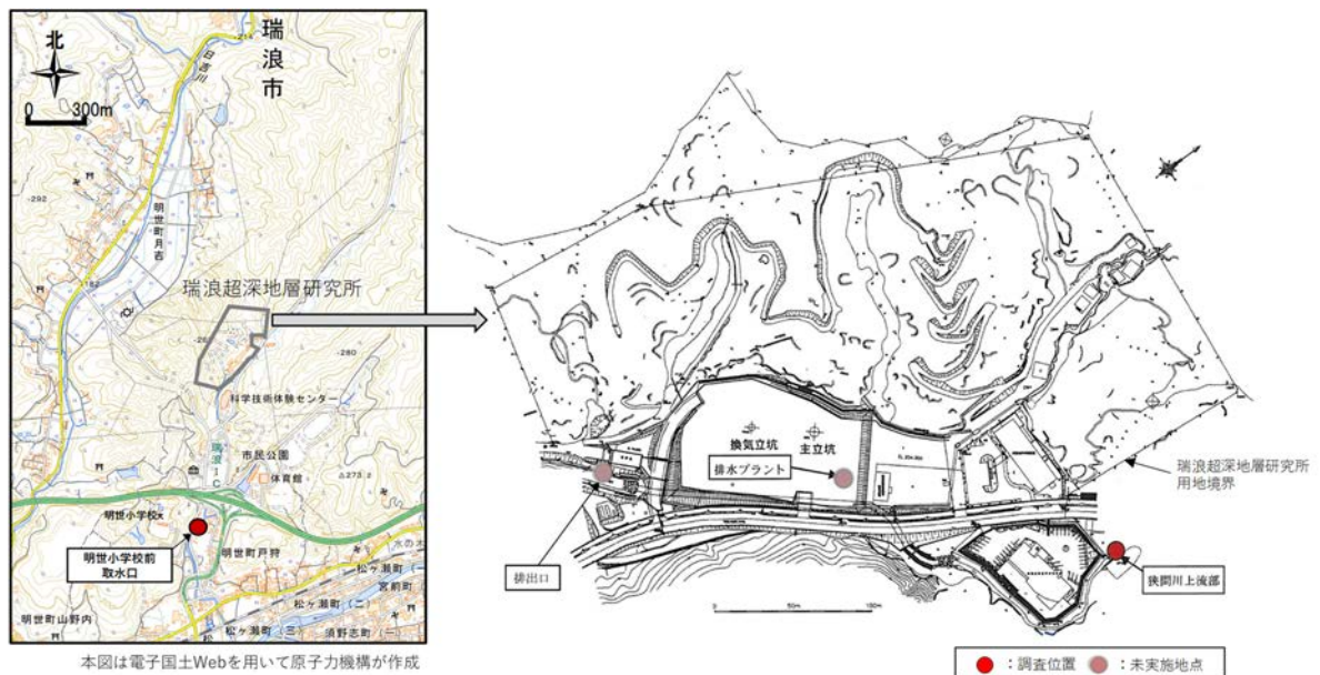
図3.3.1-3 試料採取地点図（塩化物イオン測定）
