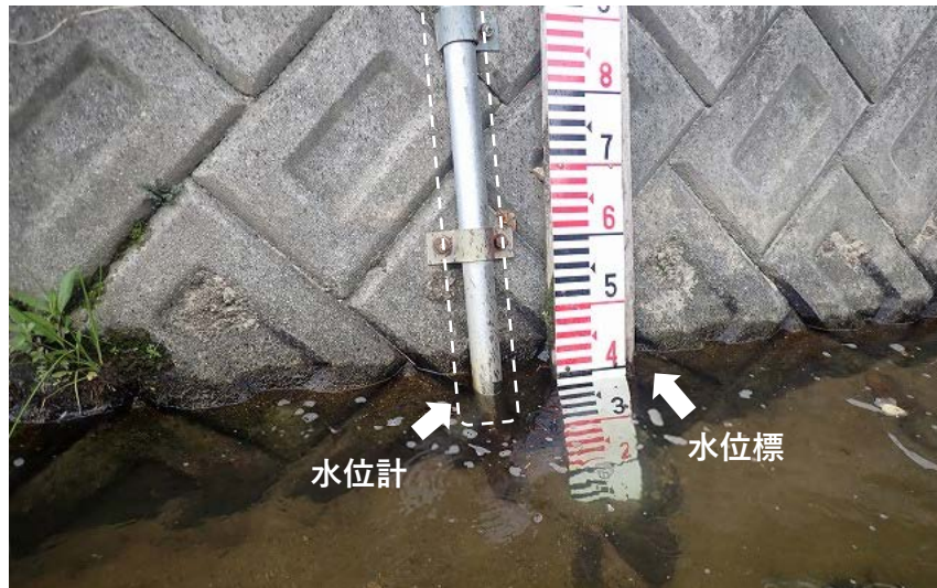
図3.2.1-3 上流地点の水位標・水位計設置状況
