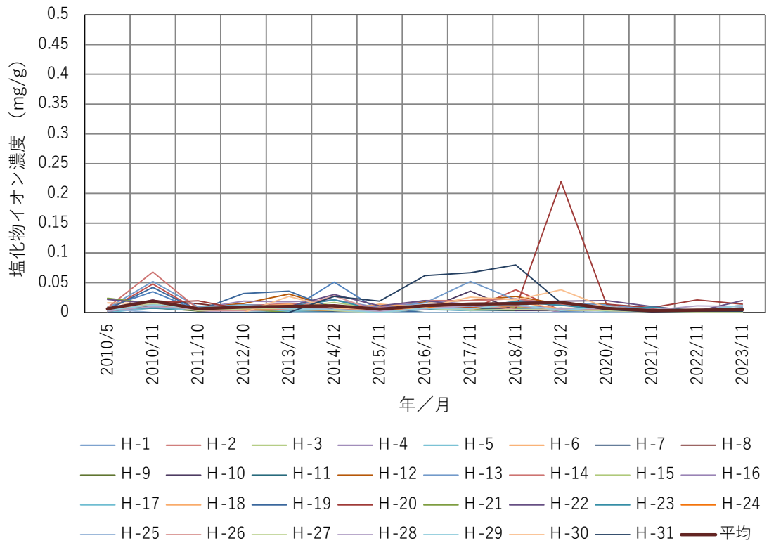
図3.5.2-1 灰の塩化物イオン濃度の経年変動（2023年まで）
