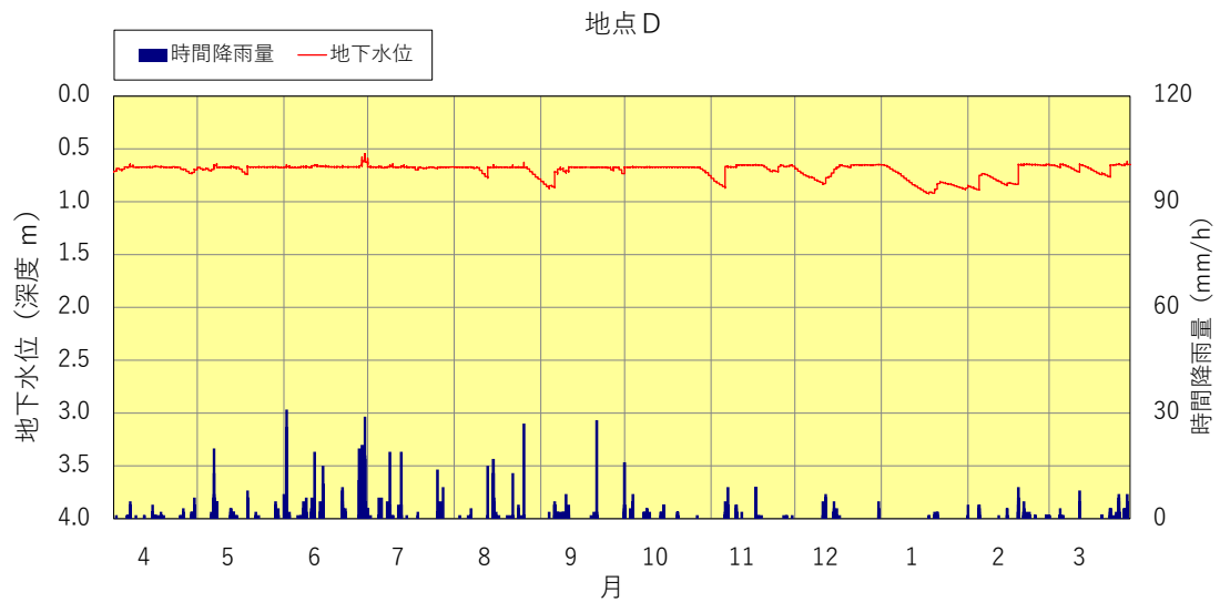
図3.1.2-7 地下水位変動図 地点D (2023年度)
