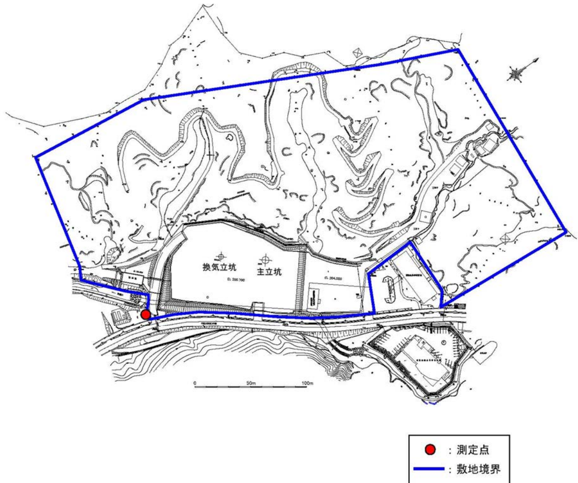
図3.4.1-1 騒音・振動調査における測定地点
