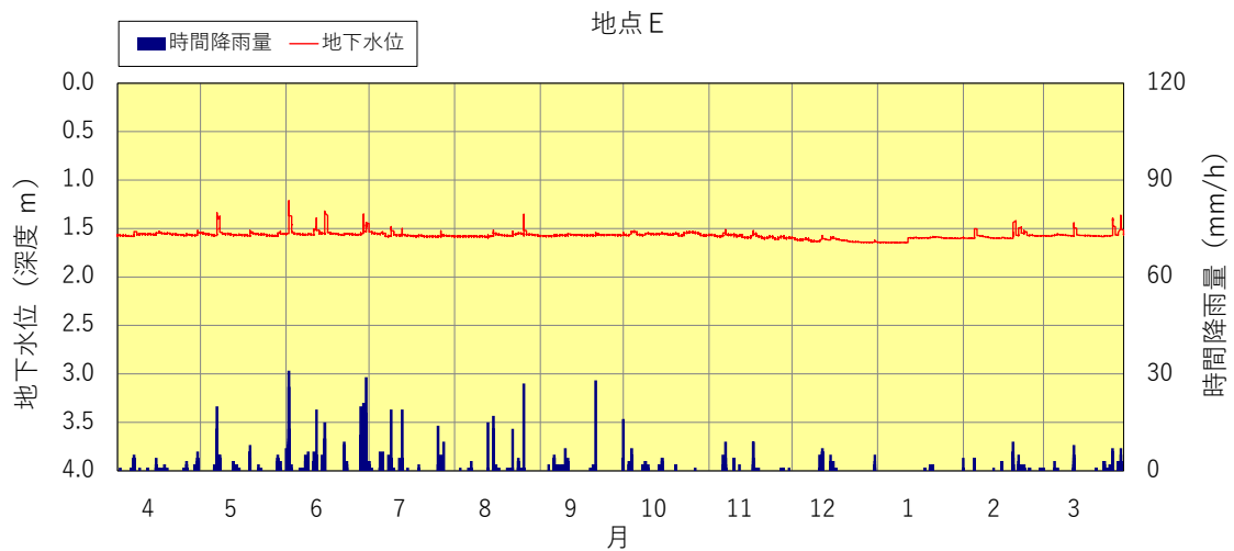
図3.1.2-9 地下水位変動図 地点E (2023年度)
