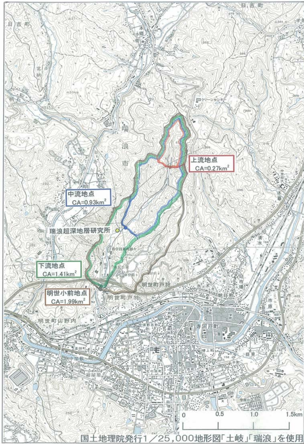
図3.2.1-2 各河川流量測定地点の流域図
