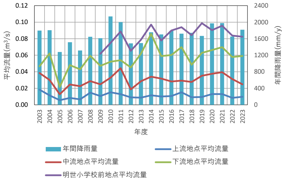
図3.2.2-1 各河川流量測定地点における年間平均流量の変動
