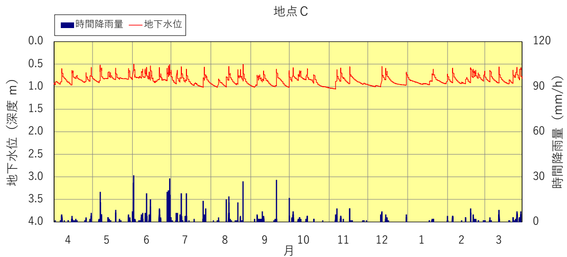
図3.1.2-5 地下水位変動図 地点C (2023年度)
