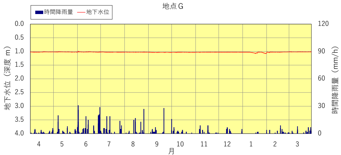
図3.1.2-13 地下水位変動図 地点G (2023年度)
