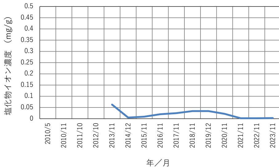
図3.5.2-3 河床の塩化物イオン濃度の経年変動（2023年まで）
