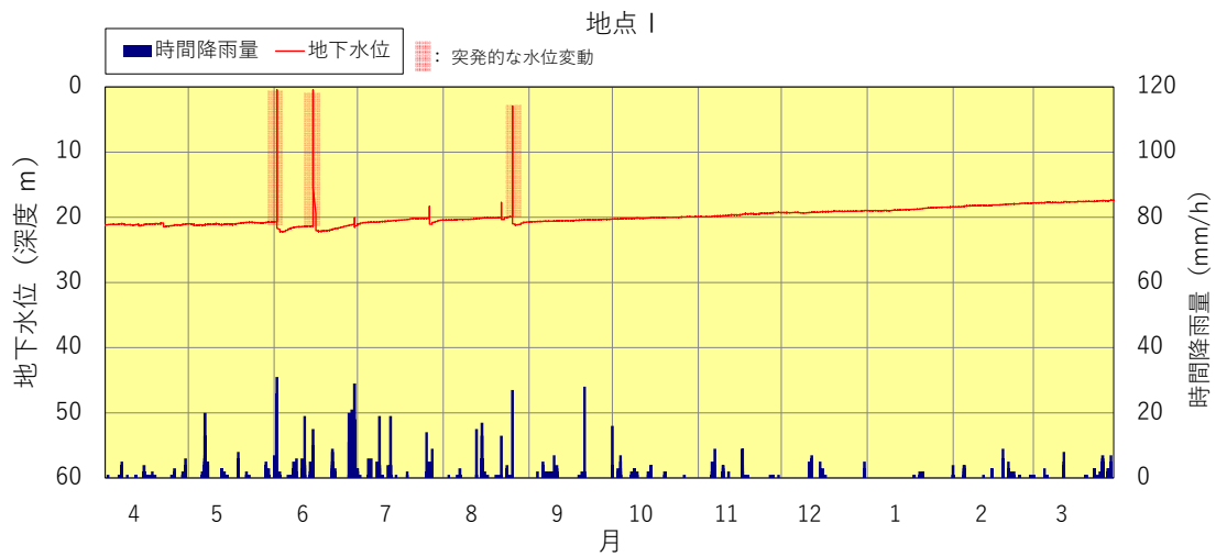
図3.1.2-15 地下水位変動図 地点I (2023年度)
