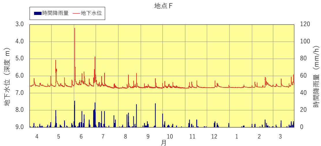
図3.1.2-11 地下水位変動図 地点F (2023年度)
