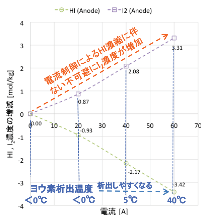
電流制御における陽極溶液の濃度変化(出口)
