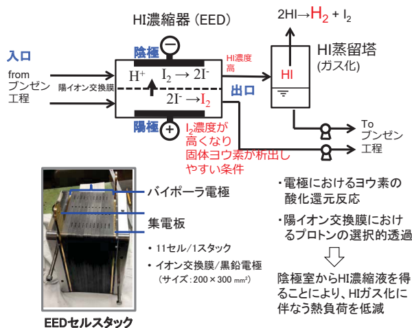
EEDセルスタック
