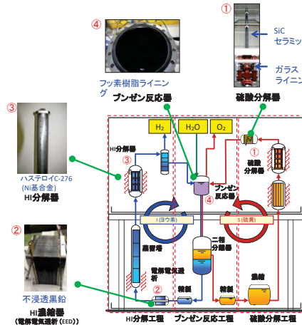
連続水素製造試験装置 3階建鉄骨構造 塩ビ板囲い (幅18.5m×奥行5.0m×高さ8.1m)
