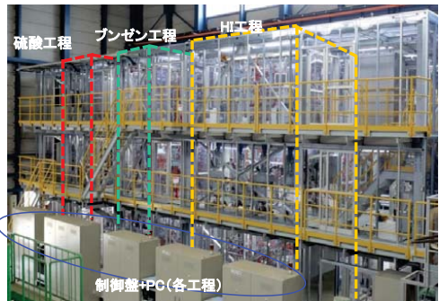
連続水素製造試験装置 3階建鉄骨構造 塩ビ板囲い (幅18.5m×奥行5.0m×高さ8.1m)
