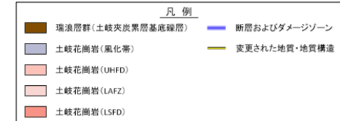
図 4.4.3-2 Stage300 地質構造モデルの更新結果の比較 (水平断面図)
