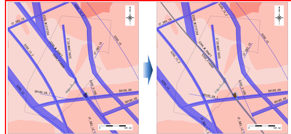
Substage200地質構造モデルの深度200m水平断面図
