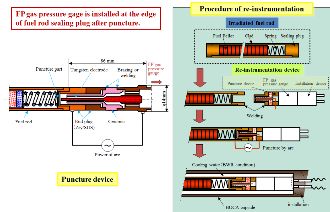
図 9 照射済燃料への熱電対及び FP ガス圧力計の再計装技術
