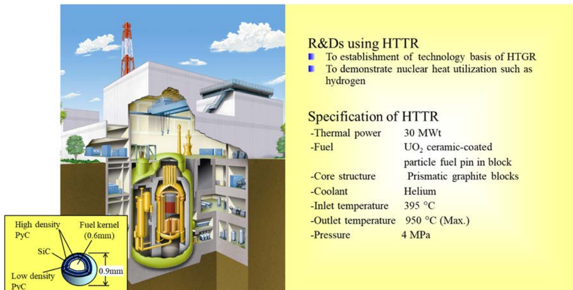
図 6 HTTR の概要 3)
