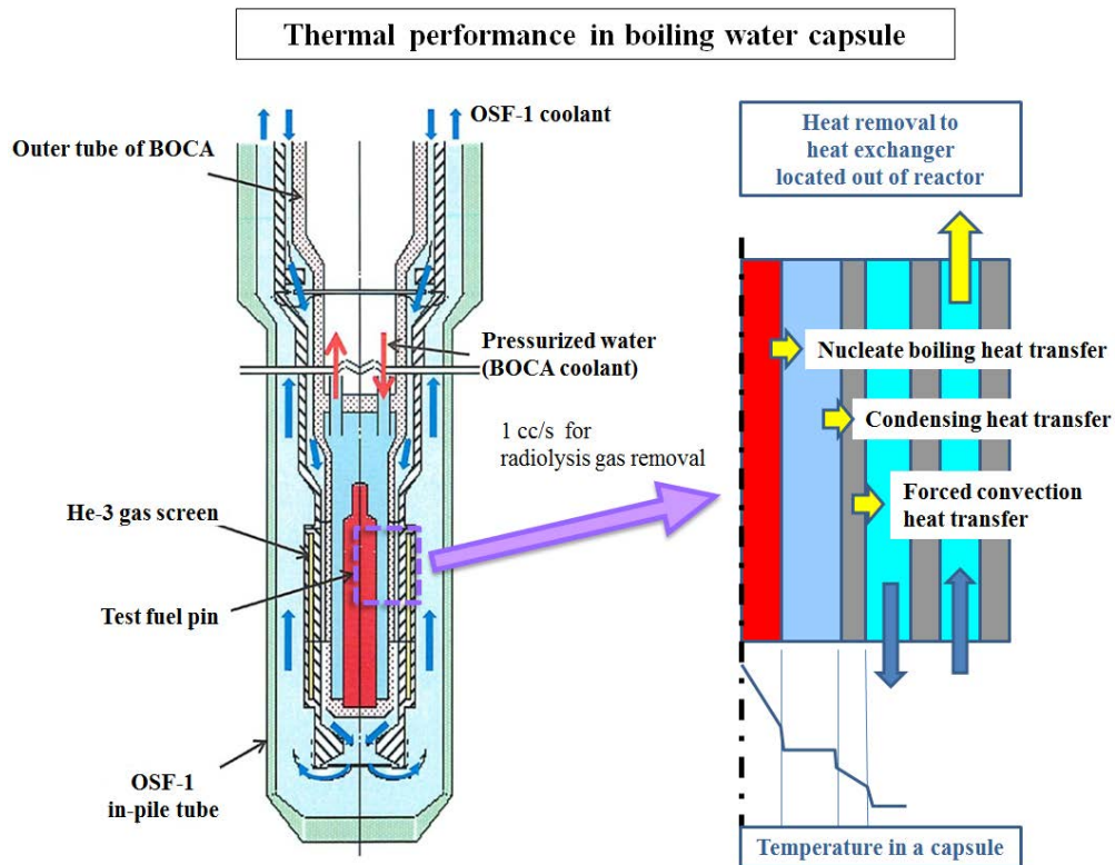
図 10 沸騰水キャプセルの熱移動
