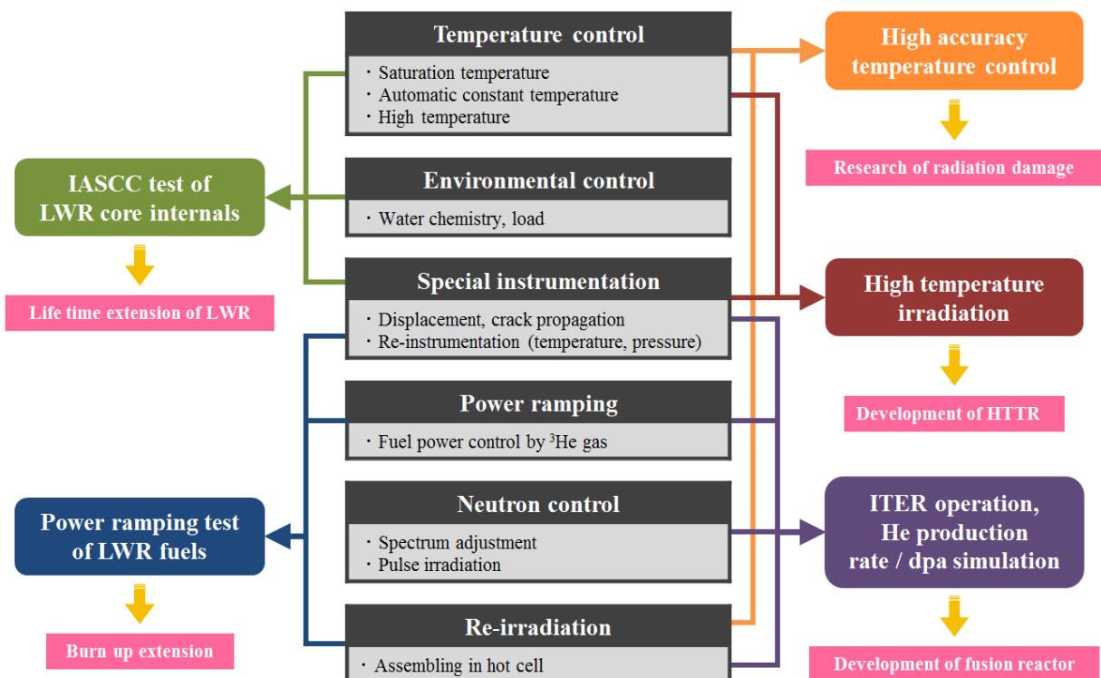
図 8 JMTR の照射技術
