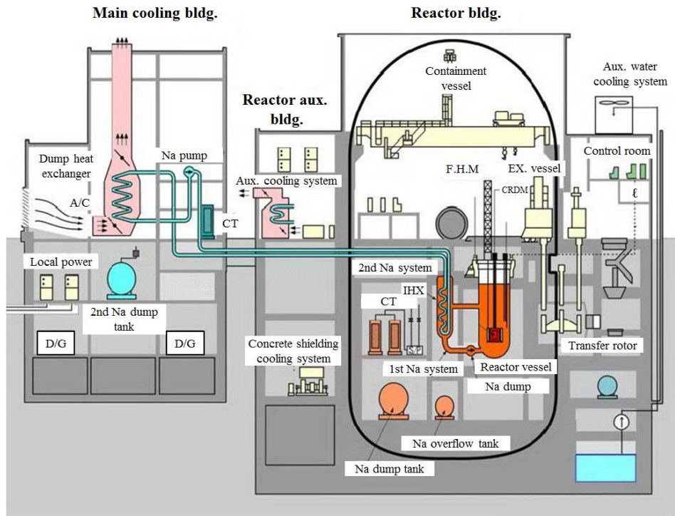
図 5 「常陽」の概要 3)
