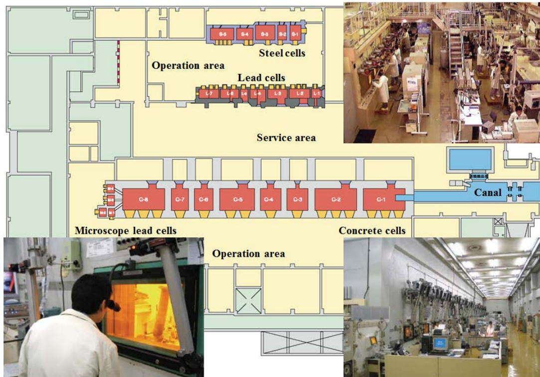
図 7 JMTR HL のホットセルの概要 2)
