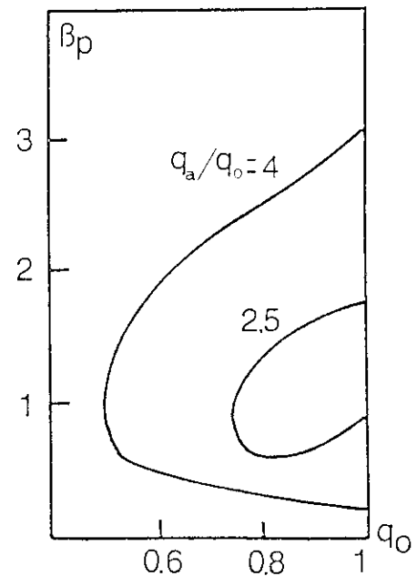
図 6.6 q_a/q_0 = 2.5 および 4.0 の場合の m=1 内部キックモードの (q_0, \beta_p) 平面における安定図。各々の臨界安定曲線の内部でモードは不安定。
