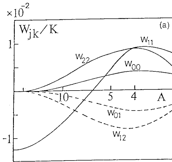
図 6.9(a) 各フーリエ成分のポテンシャル・エネルギーへの寄与 W_{m,m'} のアスペクト比依存性。 nq_0 と k(=n/R_0) を固定した場合 (横軸は 1/A 日盛) 1/A \rightarrow 0 とともに W_{0,0} , W_{2,2} は正の側からゼロに W_{1,2} , W_{0,1} は負の側からゼロに近づき、 W_{1,1} は負の有限値に近づき、したがって m=1 内部キック・モードは不安定。平衡は円形断面で \beta_p = 1.0 , q_a/q_0 = 2.5 。
