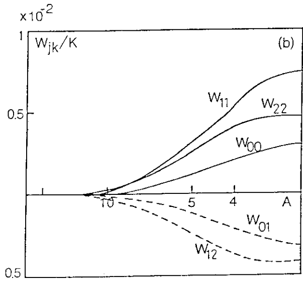
図 6.9(b) q_0 と n を固定した場合の W_{m,m'} のアスペクト比依存性。 W_{1,1} は正の側からゼロに近づき、 m=1 内部キック・モードは臨界安定。
