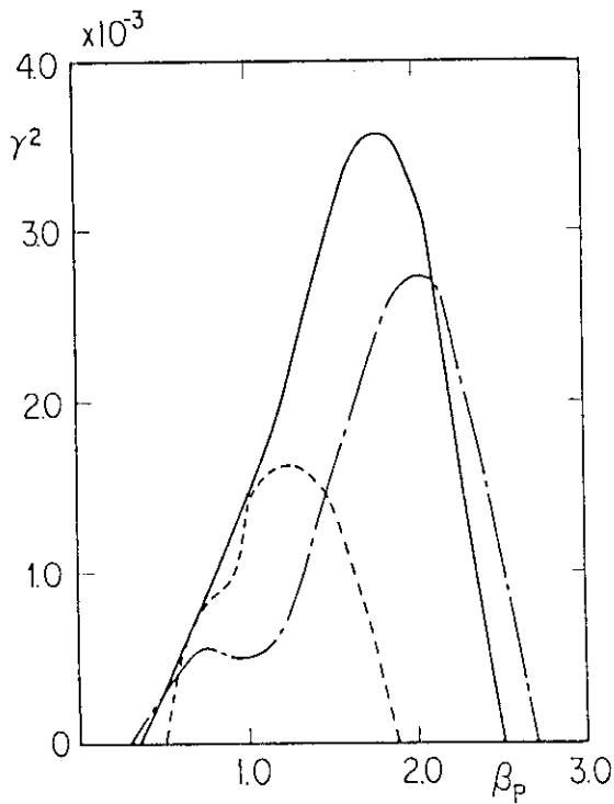
図 6.5 q_a/q_0 = 4.0 の場合の成長率の自乗 \gamma^2 の \beta_p 依存性 (破線 : q_0 = 0.6 , 実線 : q_0 = 0.8 , 一点鎖線 : q_0 = 0.9 )。
