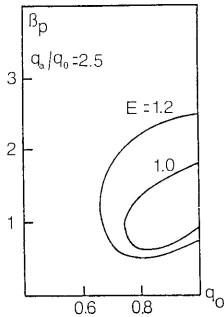
図 6.8 楕円断面平衡 ( E=1.2, q_a/q_0=2.5 ) および円形断面平衡 ( E=1.0, q_a/q_0=2.5 ) の場合の m=1 内部キック・モードの安定図。
