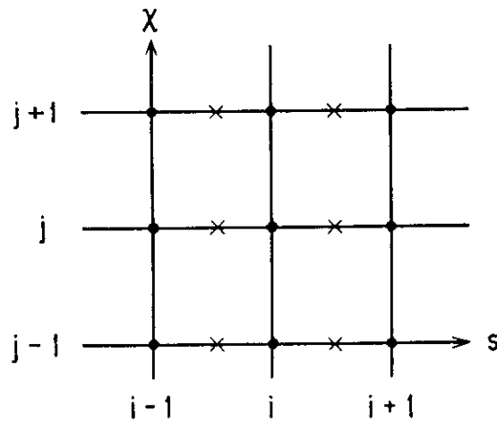
図 4.2 ERATO コードに使われる (s, X) 座標と節点 (• X, × V および Y)
