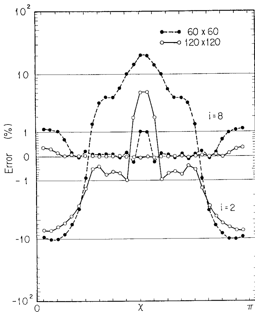
図 5.5 線積分 (5.2-2) から求めた \beta_x(\psi_i, \chi) ( i=2, 8 ) の相対誤差。格子点数は N_R \times N_z = 60 \times 60 (●印) および N_R \times N_z = 120 \times 120 (○印) である。相対誤差は \sinh^{-1} 目盛である。
