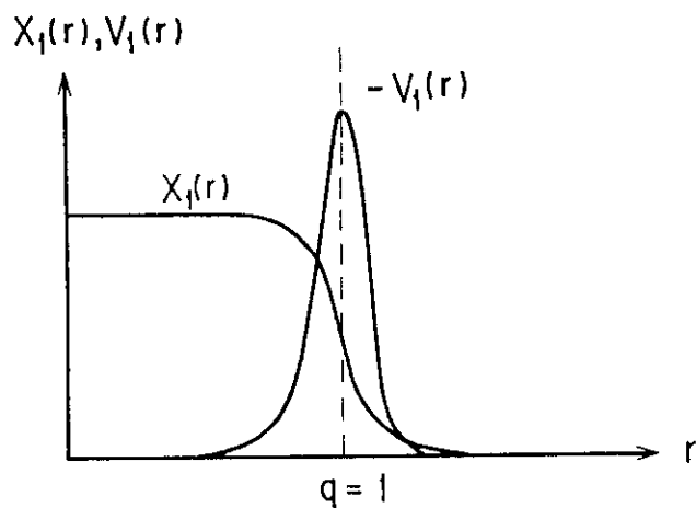
図 6.2 m=1 内部キック・モードの固有関数の概略図。(X- \xi \cdot \Delta r, V=r (\xi \cdot \Delta \chi - \xi \cdot \Delta \psi / q) )
