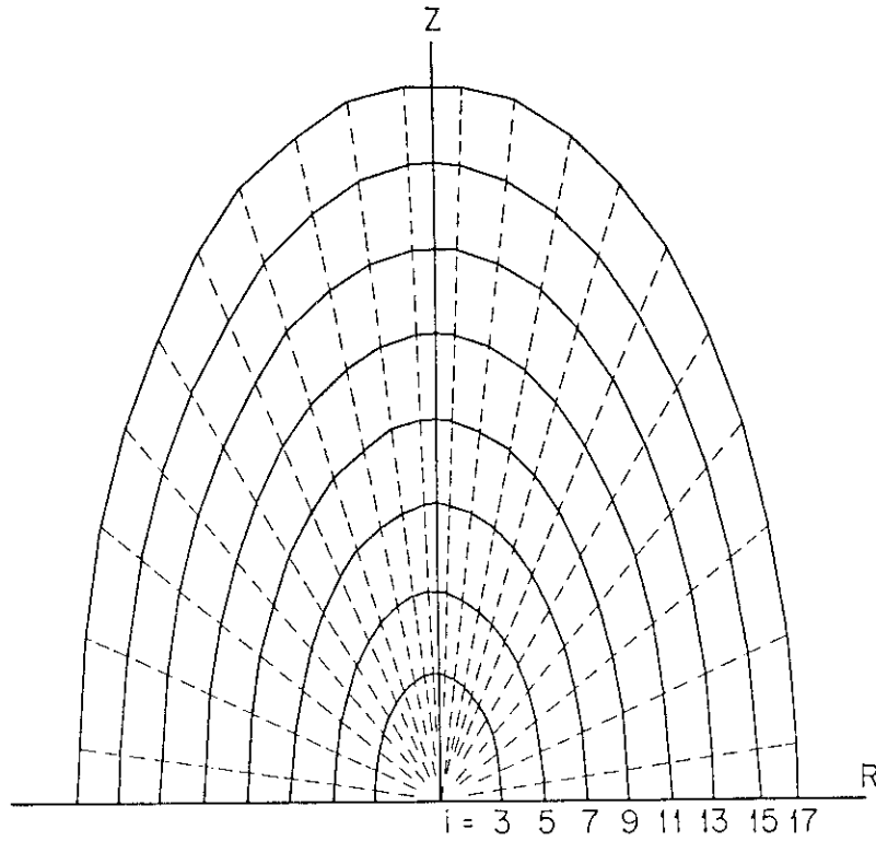
図 5.1 \psi(R, Z) = 2\pi(R^2 + Z^2/4)^2 に対する等 \psi 線 (実線) と等 \lambda 線 (破線)。(R, Z)座標の格子点数 N_R \times N_Z は 60 \times 60 であり, 等 \psi 線の値 \psi_i は \psi_i = 2\pi R_i^4 , R_i = (1 - 3J_R)i/40 ( i = 1, 2, \dots, 40 ), J_R = 2/55 である。関数 \psi(R, Z) は 3 次のスプライン関数で補間される。
