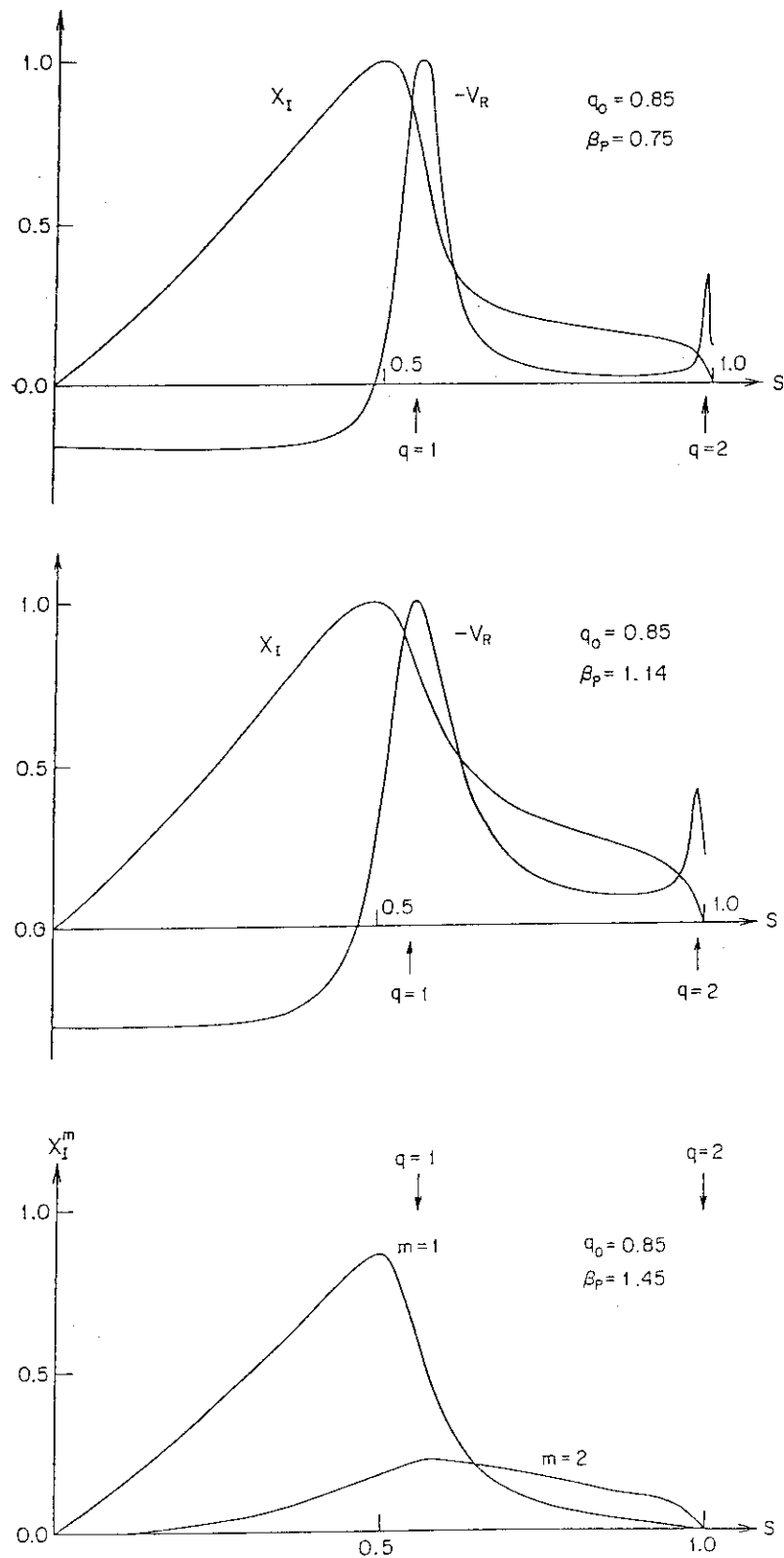
図 6.11 m=1 内部キンク・モードの固有関数 X_I (\sim s \xi^s) と V_R (\sim \xi^x - \xi^y/q) の \chi=0 面における s -依存性 (a) \beta_P=0.75 (b) \beta_P=1.14 (c) \beta_P=1.45 。平衡は円形断面 q_a/q_0=2.5, q_0=0.85 。
