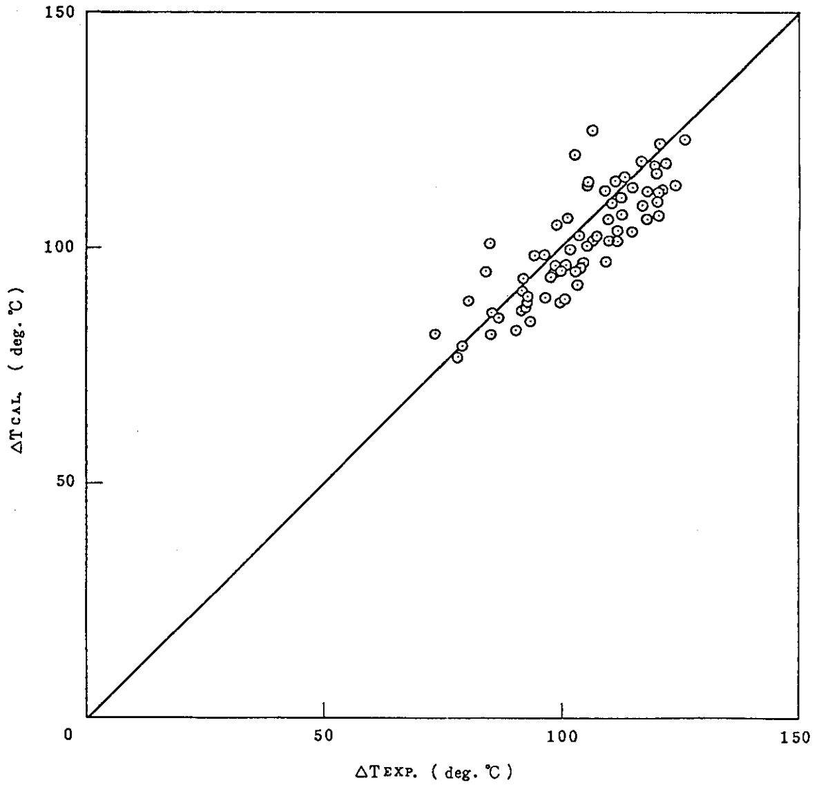
Fig. 5.10 境膜温度差の比較 (最適式)
