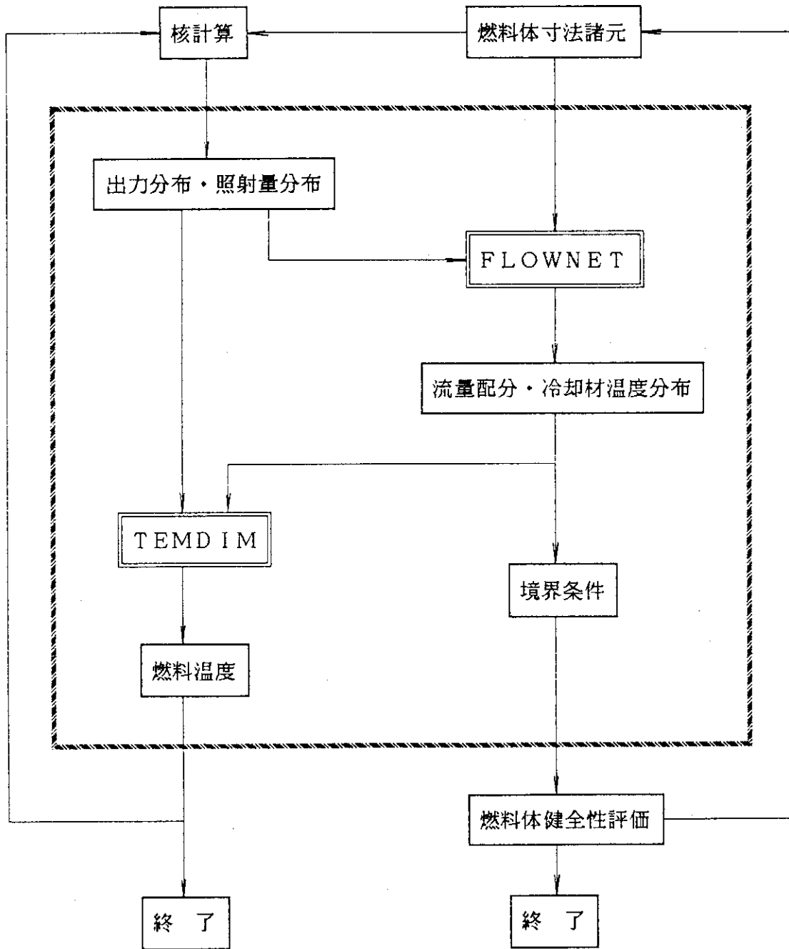
Fig. 1.4 熱流力設計の概要
