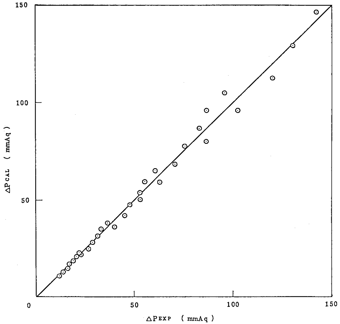
Fig. 5.22 各段毎の圧力損失の比較 (最適式)
