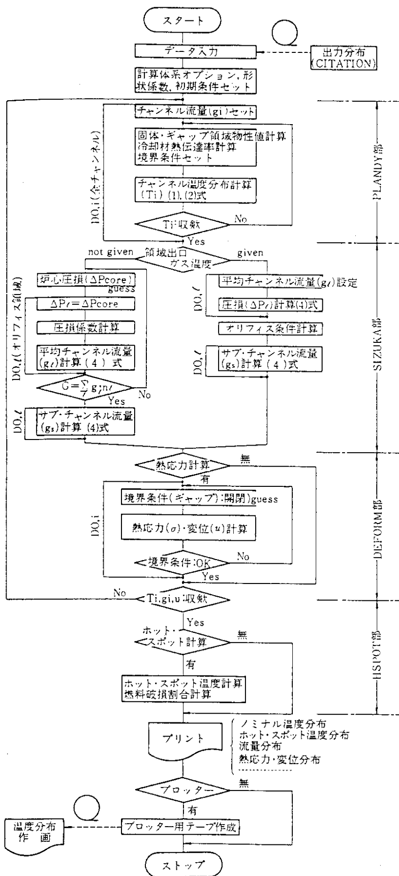
Fig. 2.1 TEMDIMフローチャート
