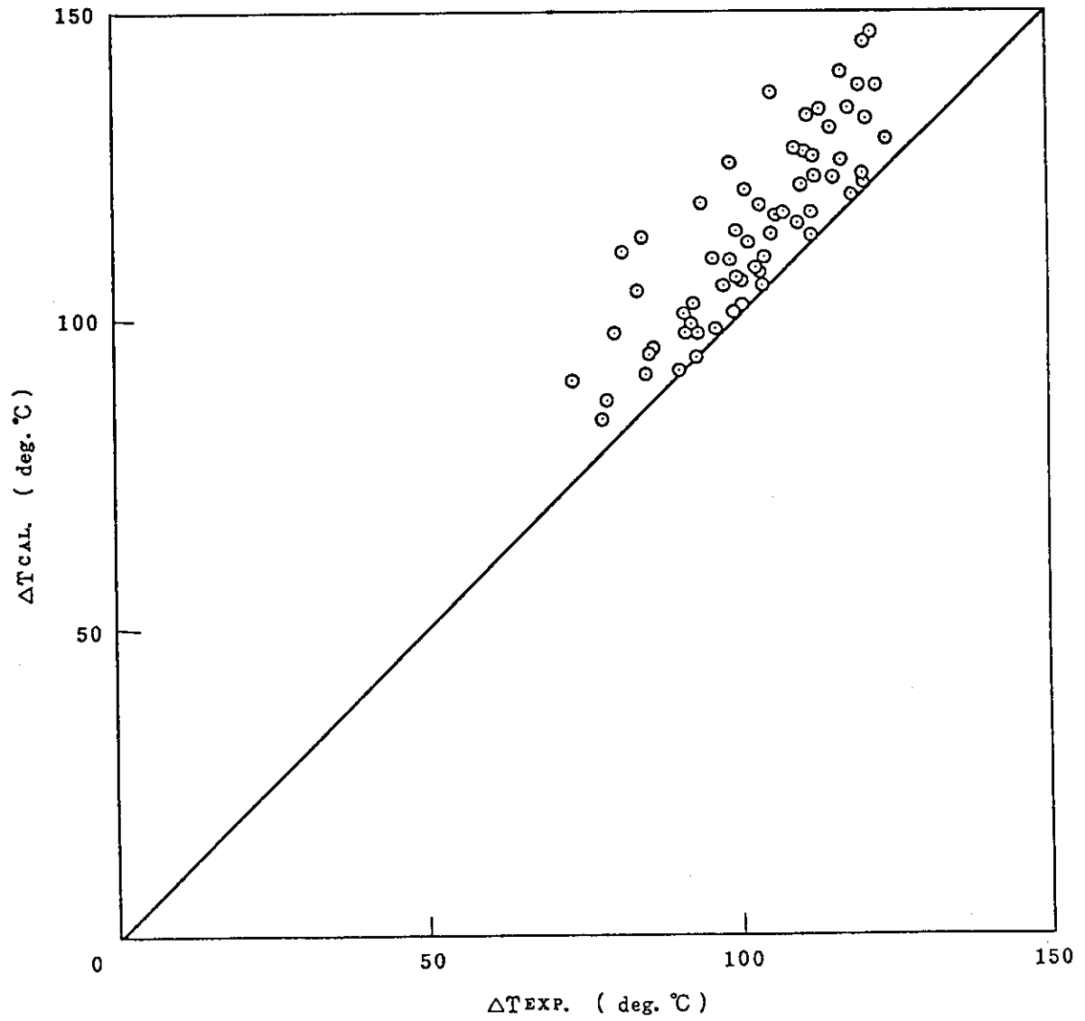
Fig. 5.11 境膜温度差の比較 (設計式)
