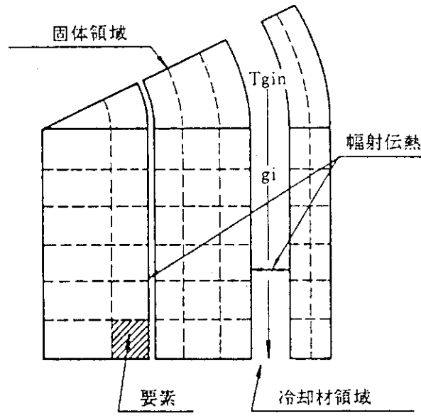
Fig. 2.2 温度分布計算モデル
