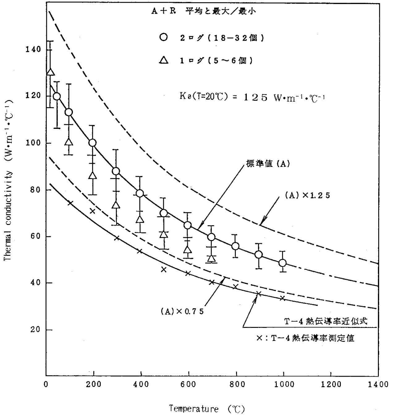
Fig. 4.10 IG-110 黒鉛及びT-4 黒鉛の熱伝導率
