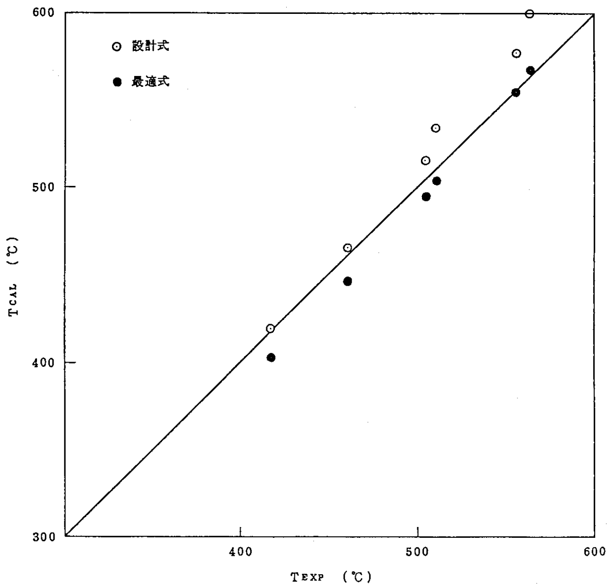
Fig. 5.12 ヒーター中心温度の比較
