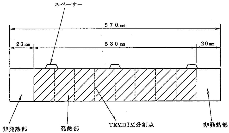
Fig. 4.2 模擬燃料棒軸方向模式図
