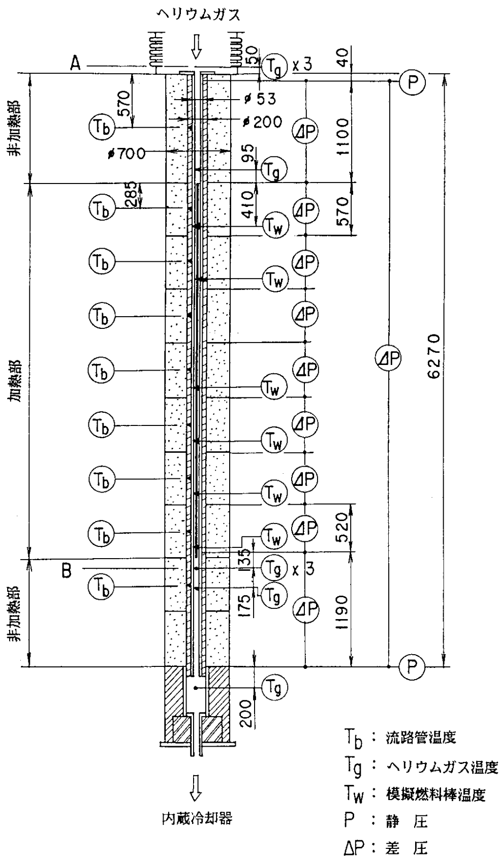
Fig. 3.4 T 1-1 試験装置計測位置
