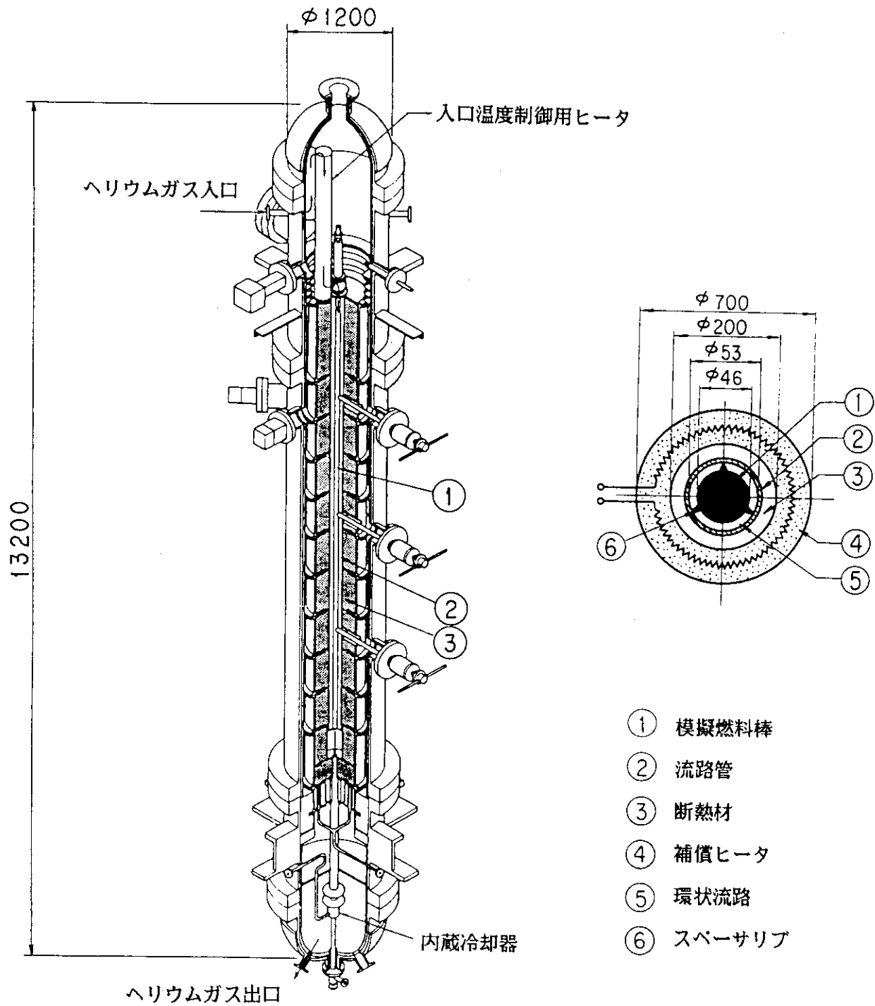
Fig. 3.2 T 1-s 試験装置の概略構造
