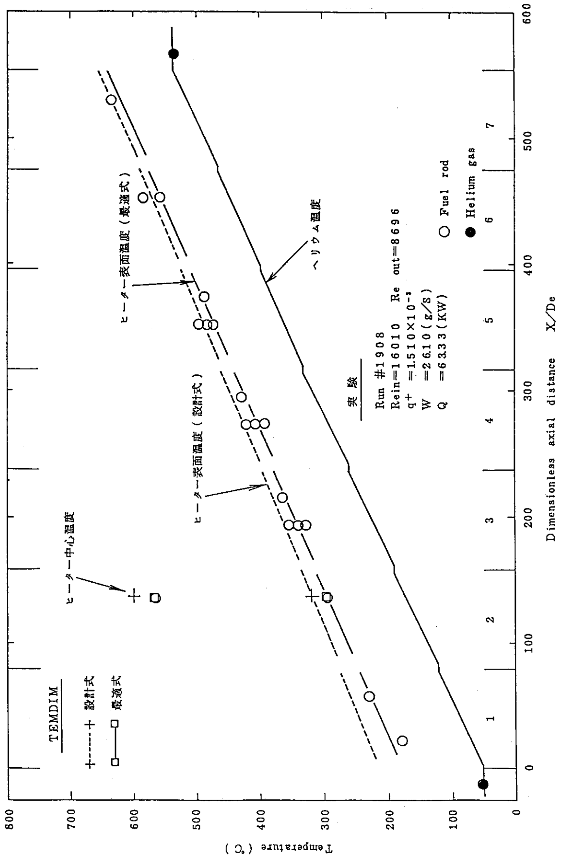
Fig. 5.6 温度分布の比較 (No.1908)
