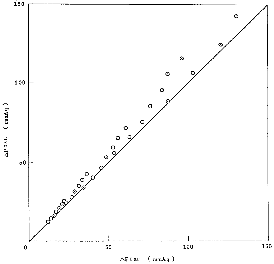
Fig. 5.23 各段毎の圧力損失の比較 (設計式)
