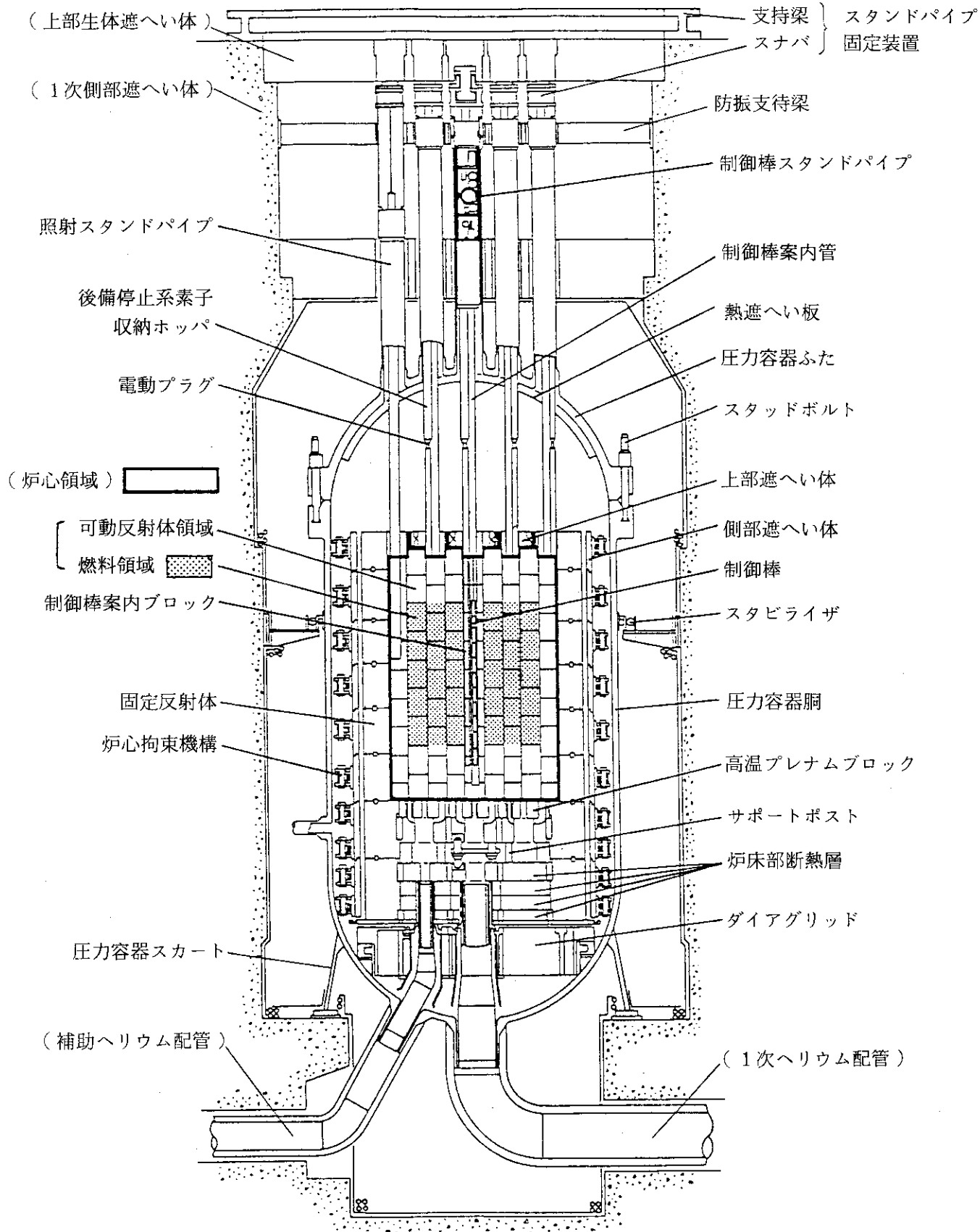
Fig. 1.1 原子炉縦断面図
