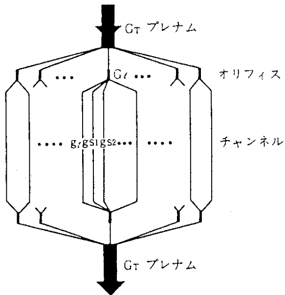
Fig. 2.3 流量配分モデル
