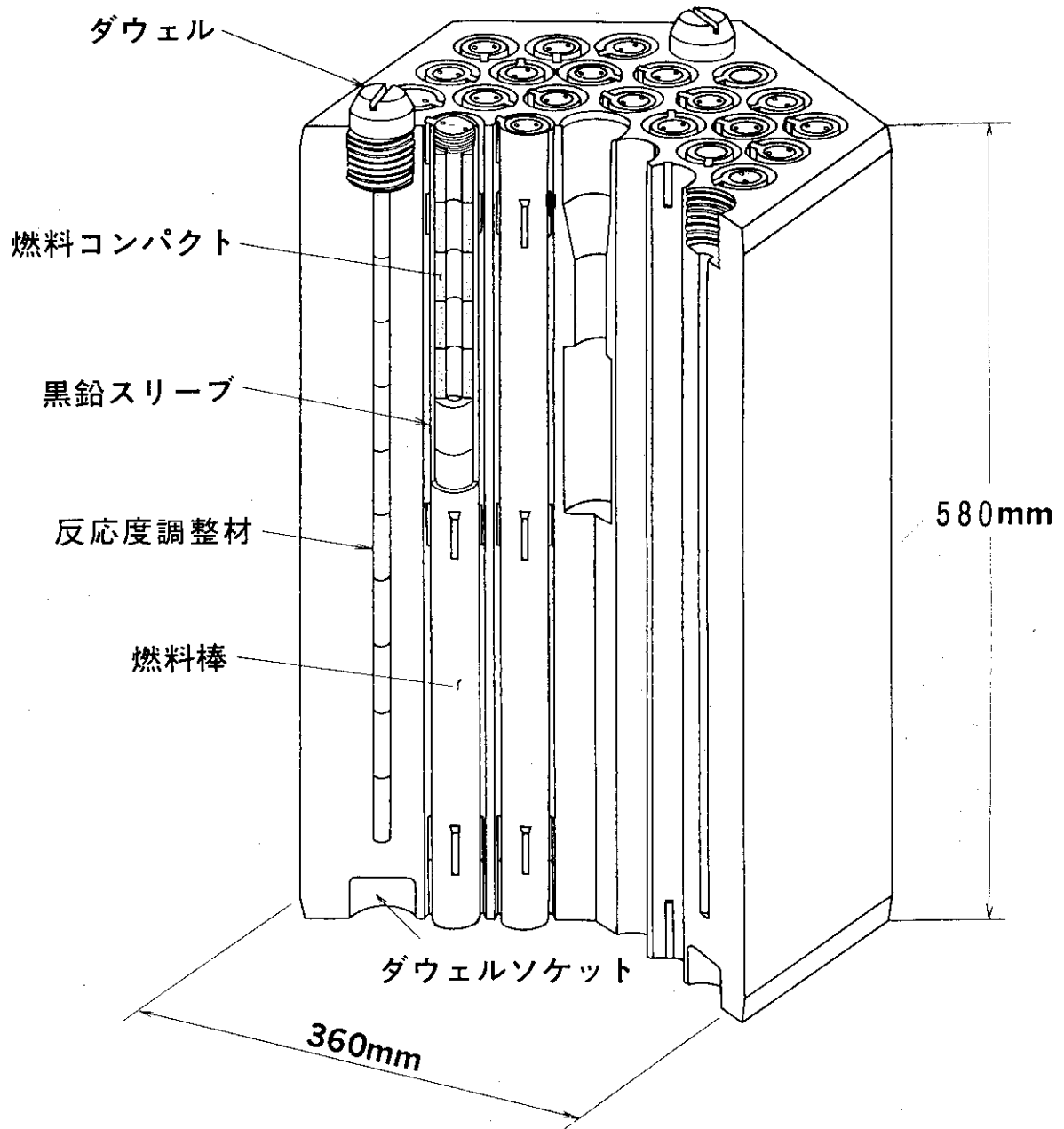
Fig. 1.3 燃料体概略構造図
