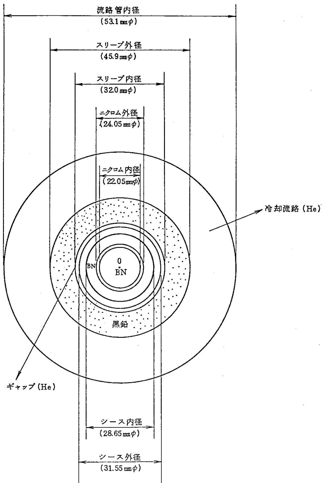
Fig. 4.1 模擬燃料棒断面図
