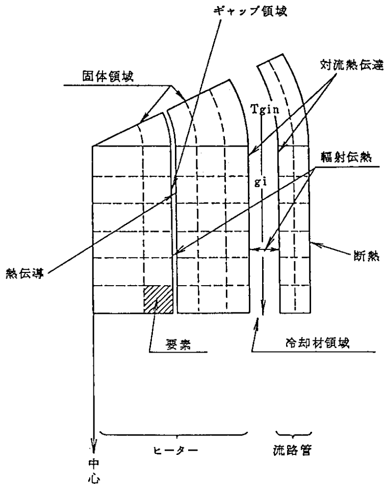
Fig. 4.3 TEMDIM温度分布計算モデル
