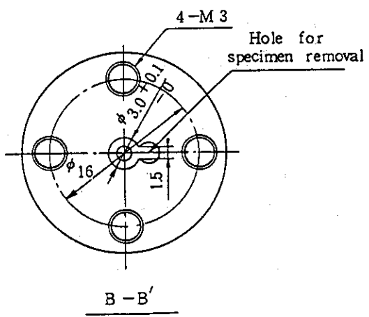
③ Lower die
