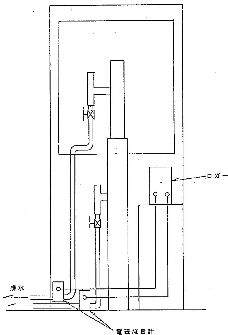
図3-2 湧水量連続観測模式図
