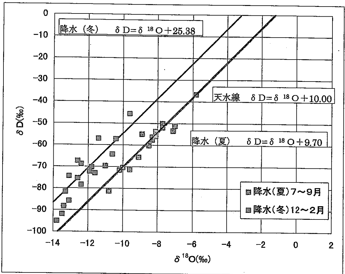
図2-6-3 水素同位体比( \delta D )と酸素同位体比( \delta^{18}O )の関係図 (降水の7~9月(夏)と12月~2月(冬)) (平成3('91)年7月~平成10('98)年2月)
