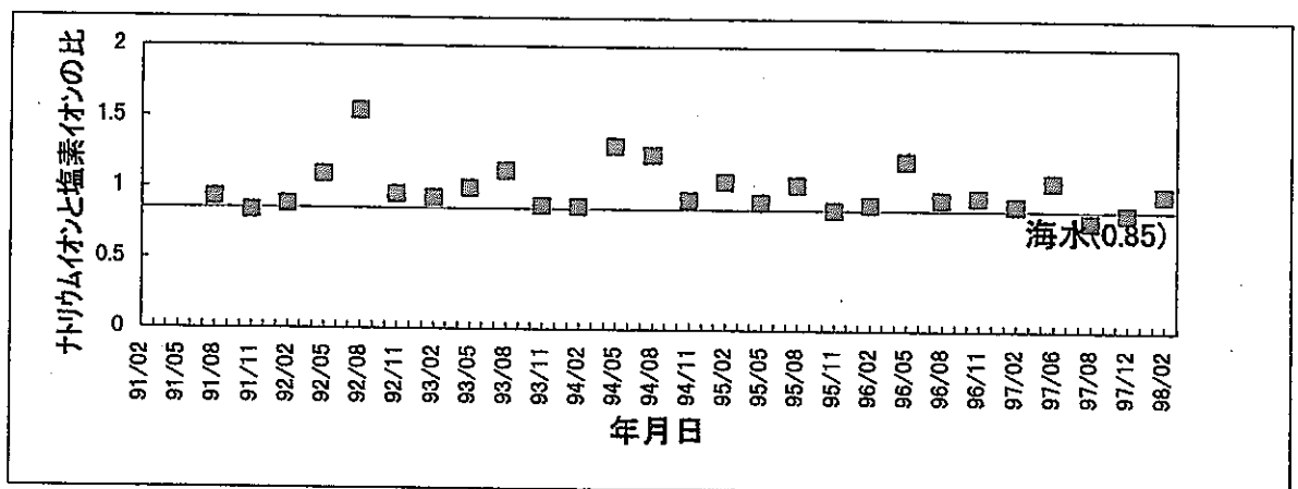
図2-6-4 dパラメータ及び塩素イオン、ナトリウムイオンの経時変化図 (1991年7月から1998年3月までのデータ)
