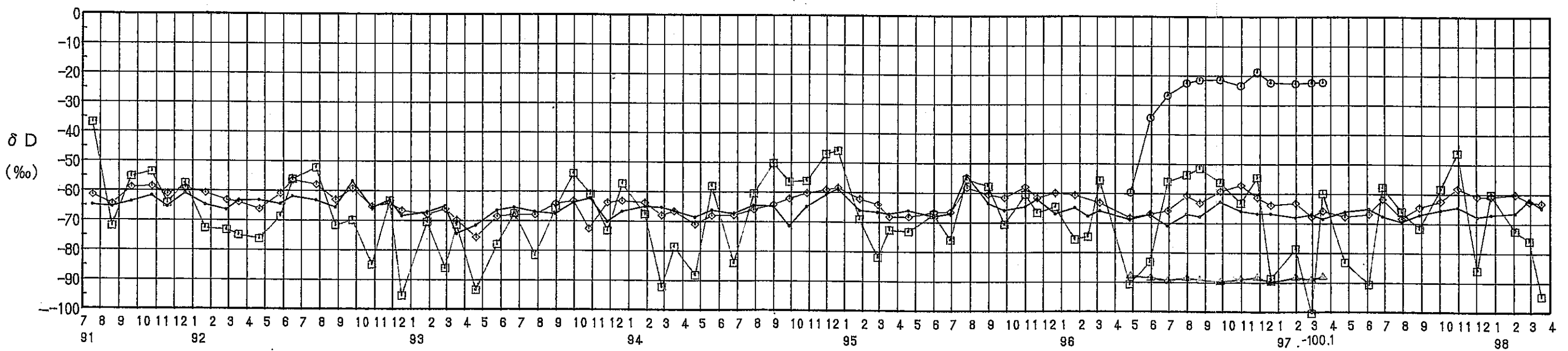
図2-6-1. 酸素同位体比 ( \delta^{18}O ) と 水素同位体比 ( \delta D ) の経時変化図
