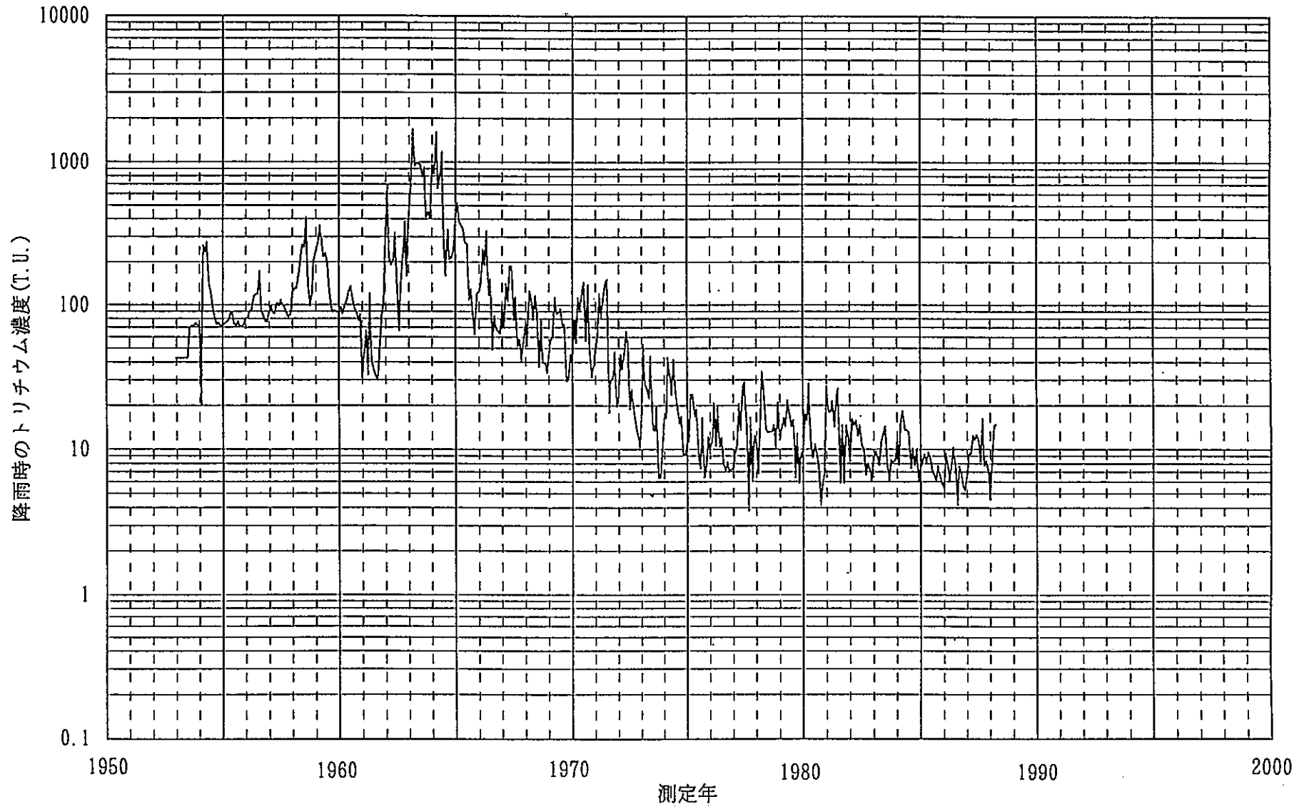
図3-1 降水中のトリチウム濃度 (Sanjo, 1990) (5) から引用
