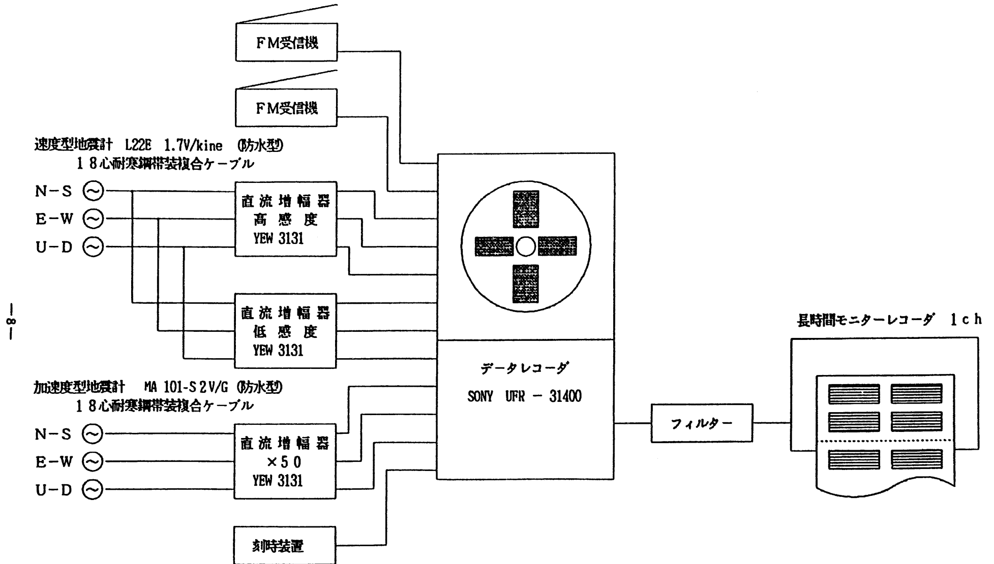
図 3・2 地震観測装置システム図 (本観測)
