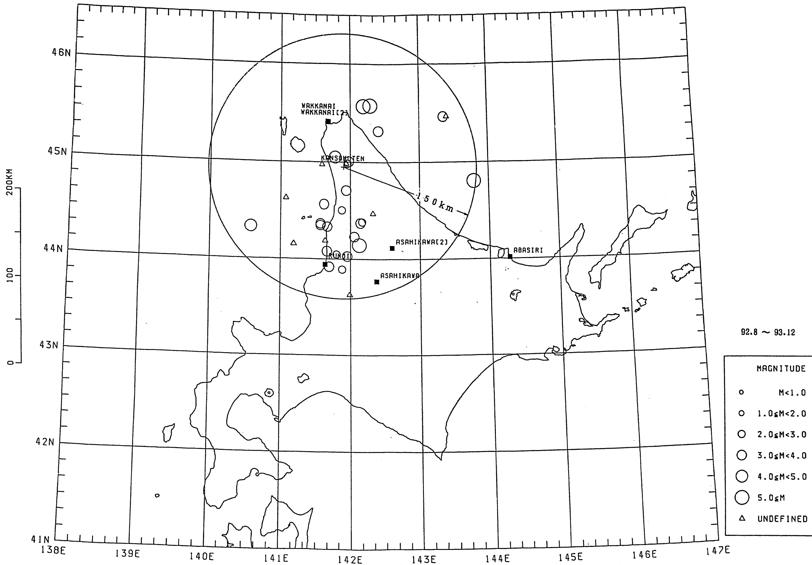
図 4・4・1 気象庁により震源決定がなされかつ観測点で検知した地震の震央 (1992年8月~1993年12月:震央距離 150km以内 N=32)
