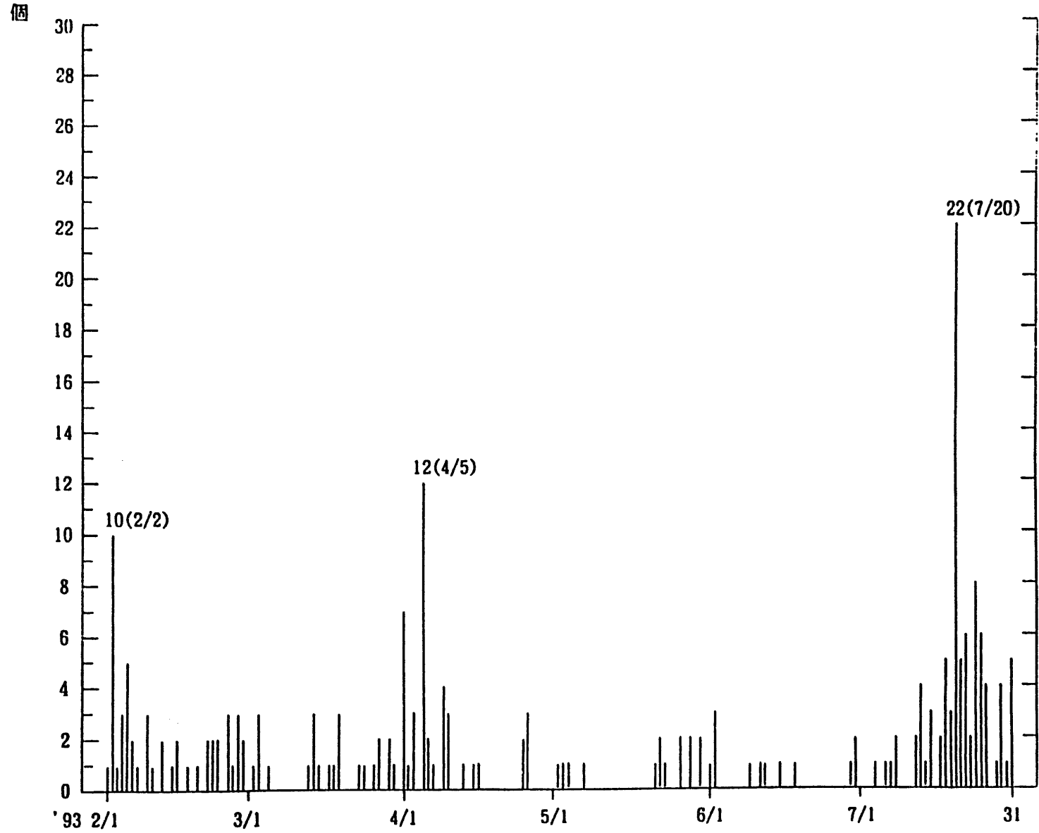
図 4・3・2 地震発生頻度 (動燃事業団1点地震観測記録の内、S-Pタイムが10秒未満の地震について)
