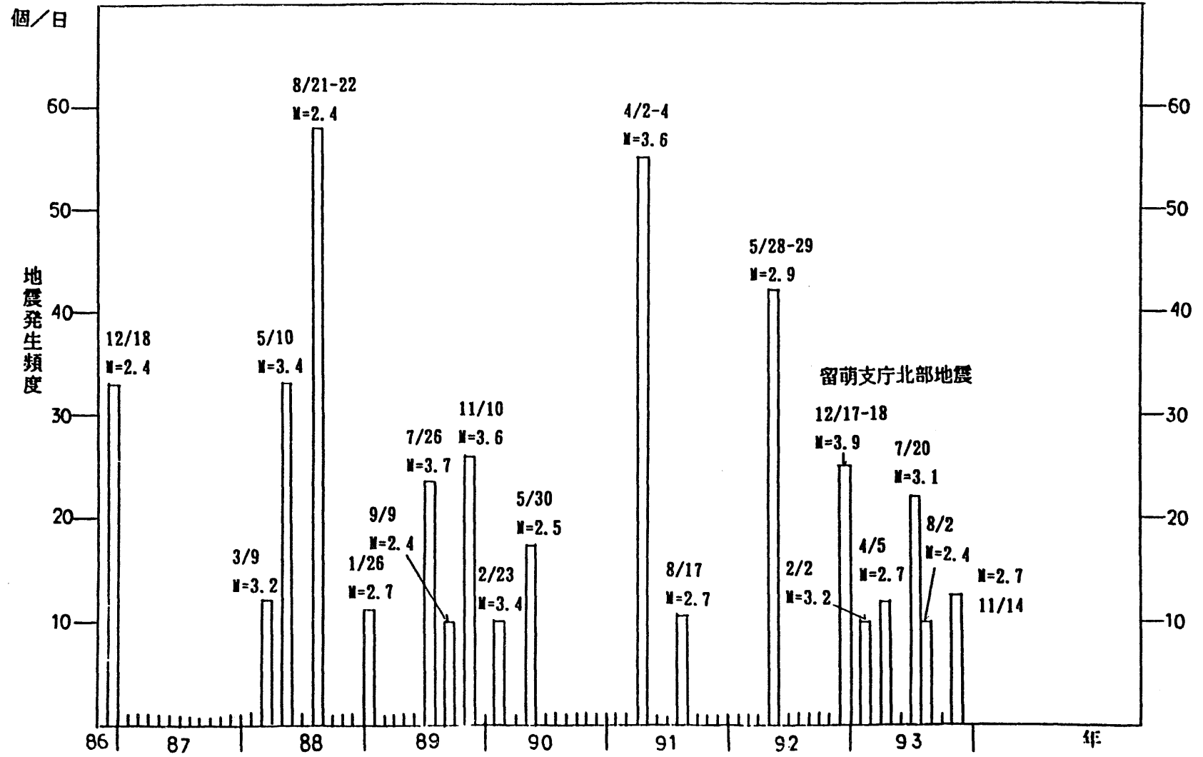
図 4・3・4 やや活発な地震活動歴と最大地震のM
