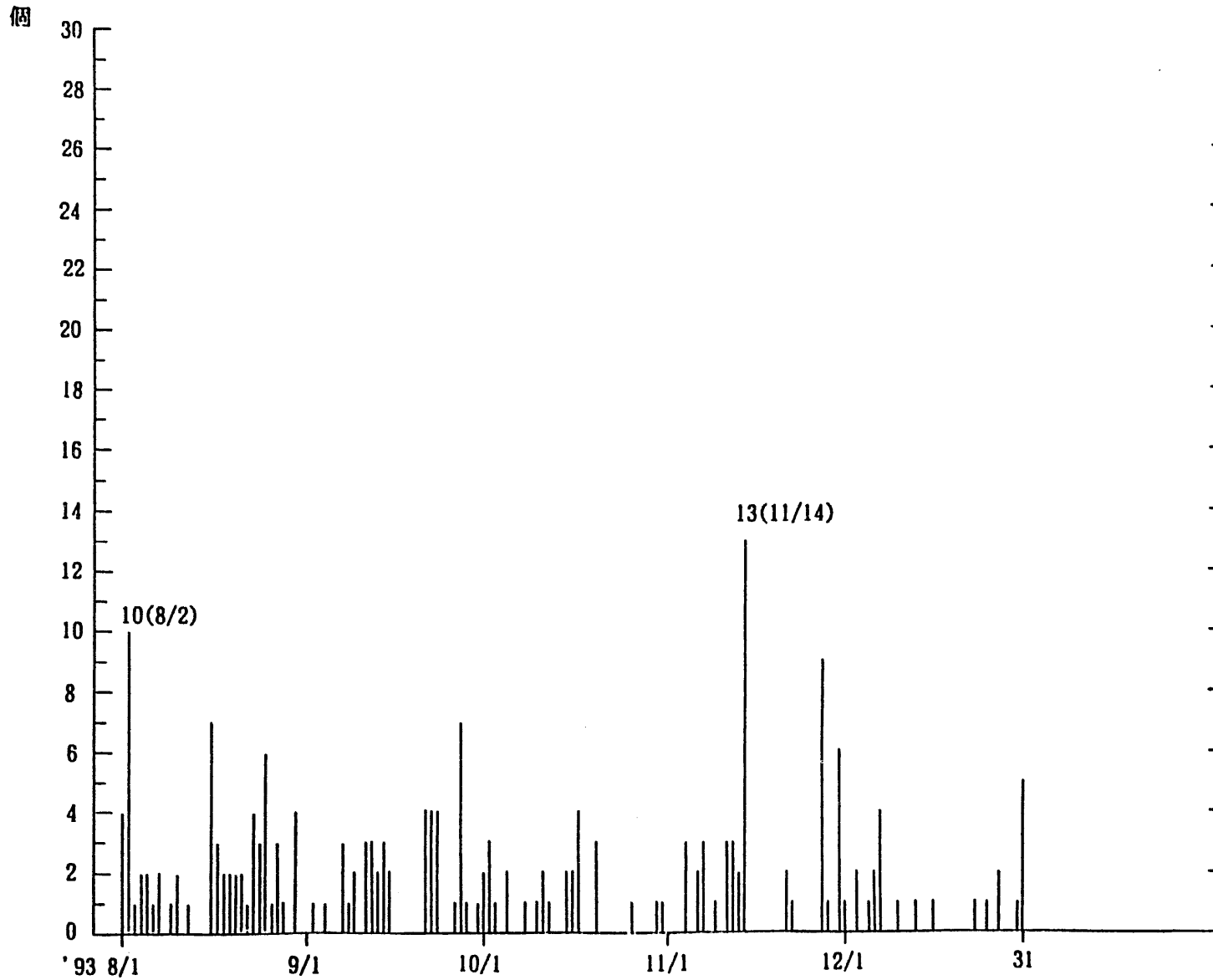
図 4・3・3 地震発生頻度 (動燃事業団 1 点地震観測記録の内、S-P タイムが 10 秒未満の地震について)
