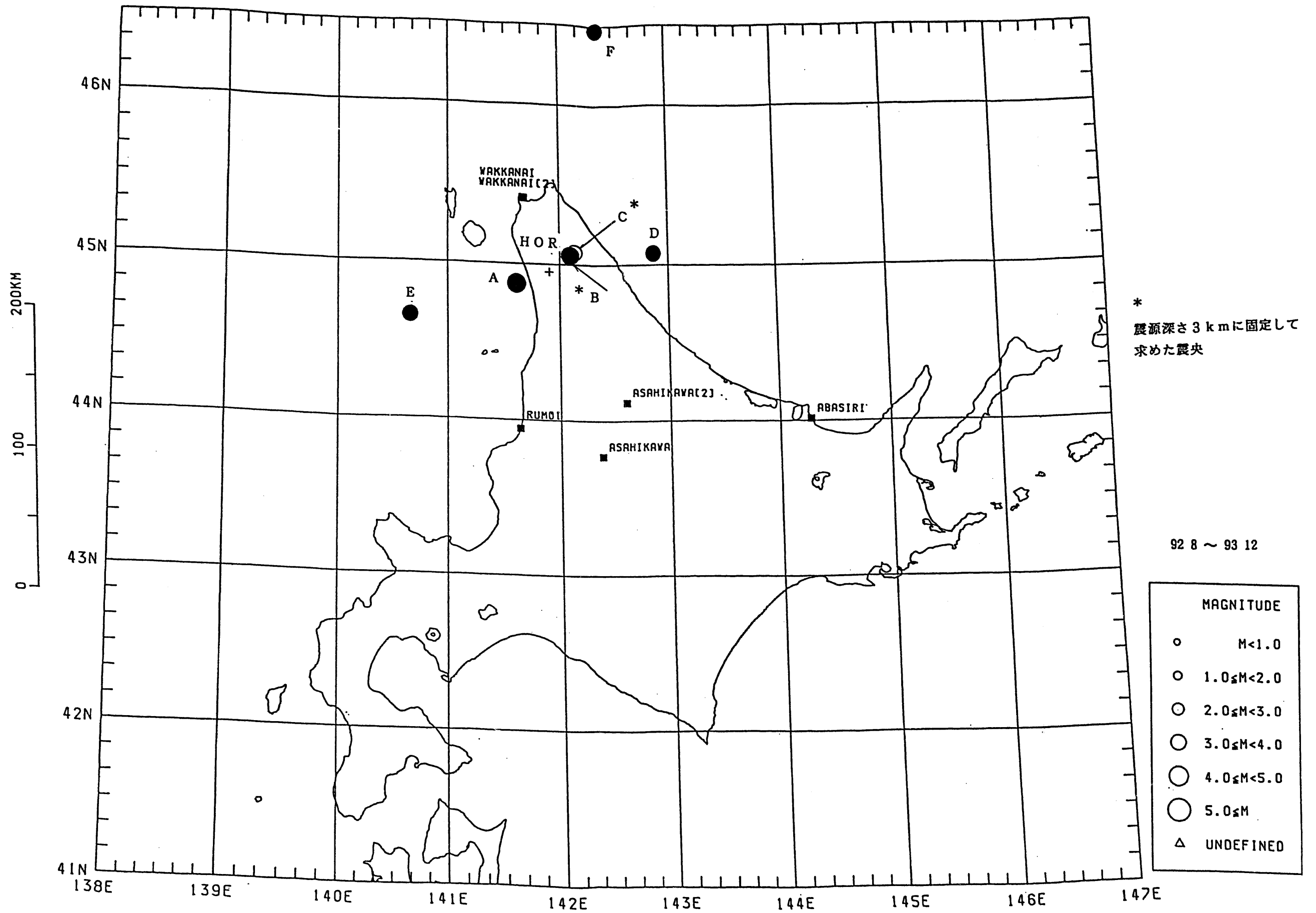
図 4・4・2 気象庁の観測点と観延観測点のデータの併合処理によって決定された地震の震央 (1992年8月~1993年12月: N=6)
