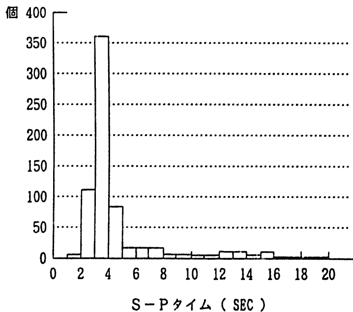
図 4-1 S-Pタイム頻度分布図 ( 20 秒以下について )
