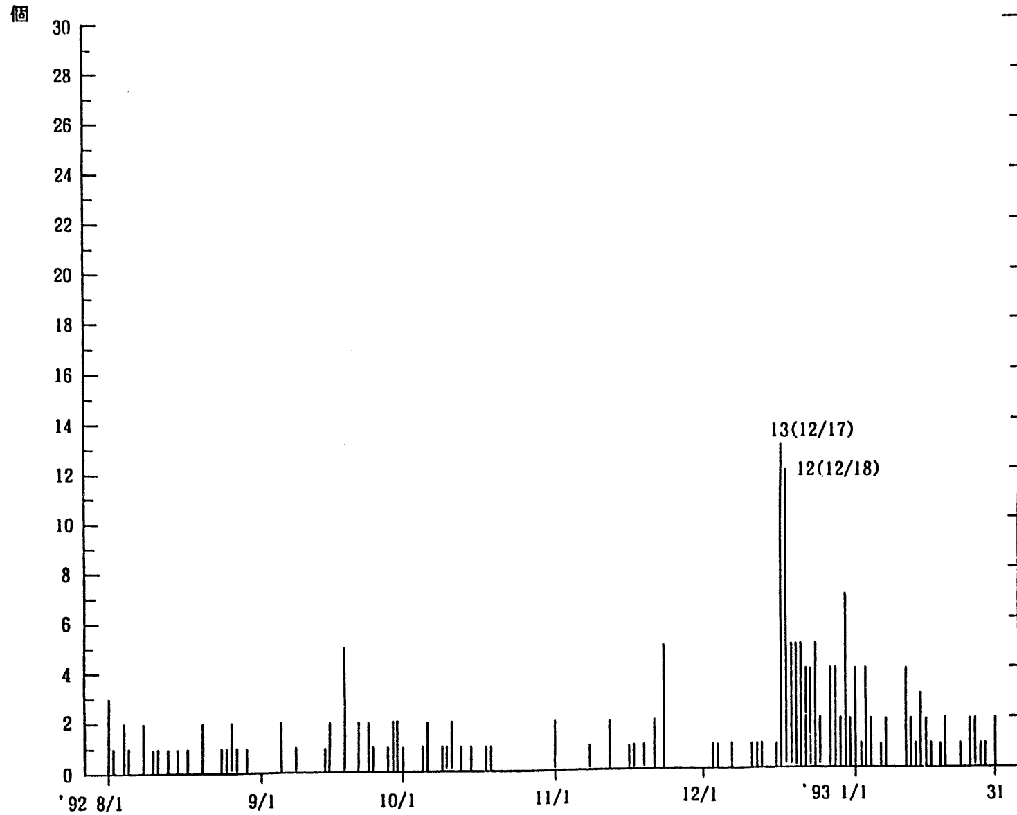
図 4・3・1 地震発生頻度 (動燃事業団1点地震観測記録の内、S-Pタイムが10秒未満の地震について)
