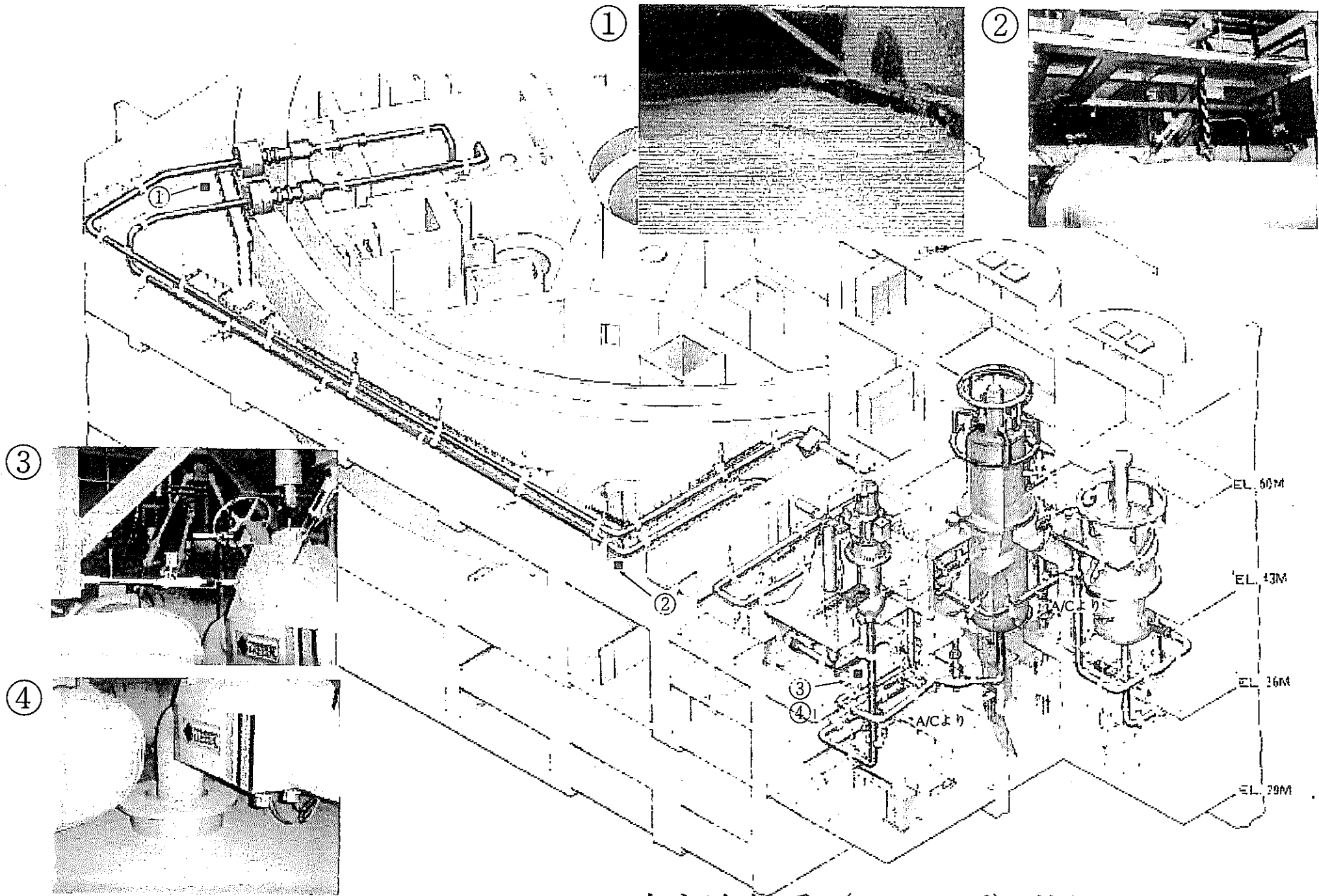
2次主冷却系 (Cループ) 状況 (1)
