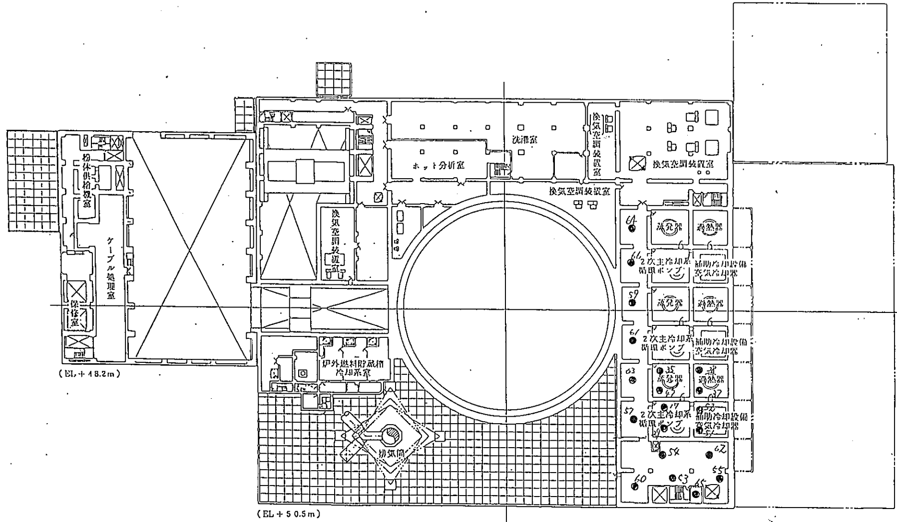
煙感知器発報位置図-1
