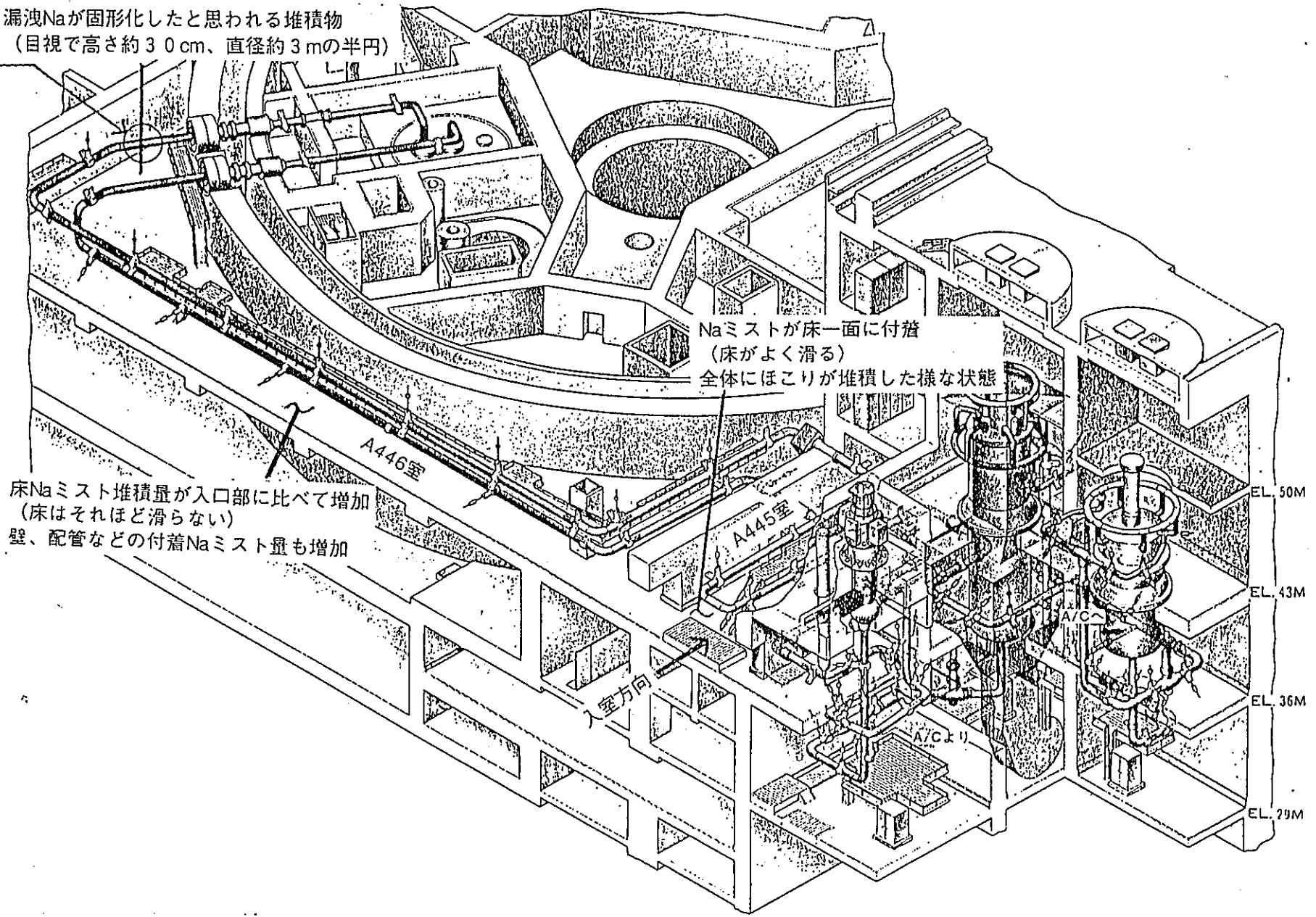
2次主冷却系 (Cループ) 鳥瞰図
