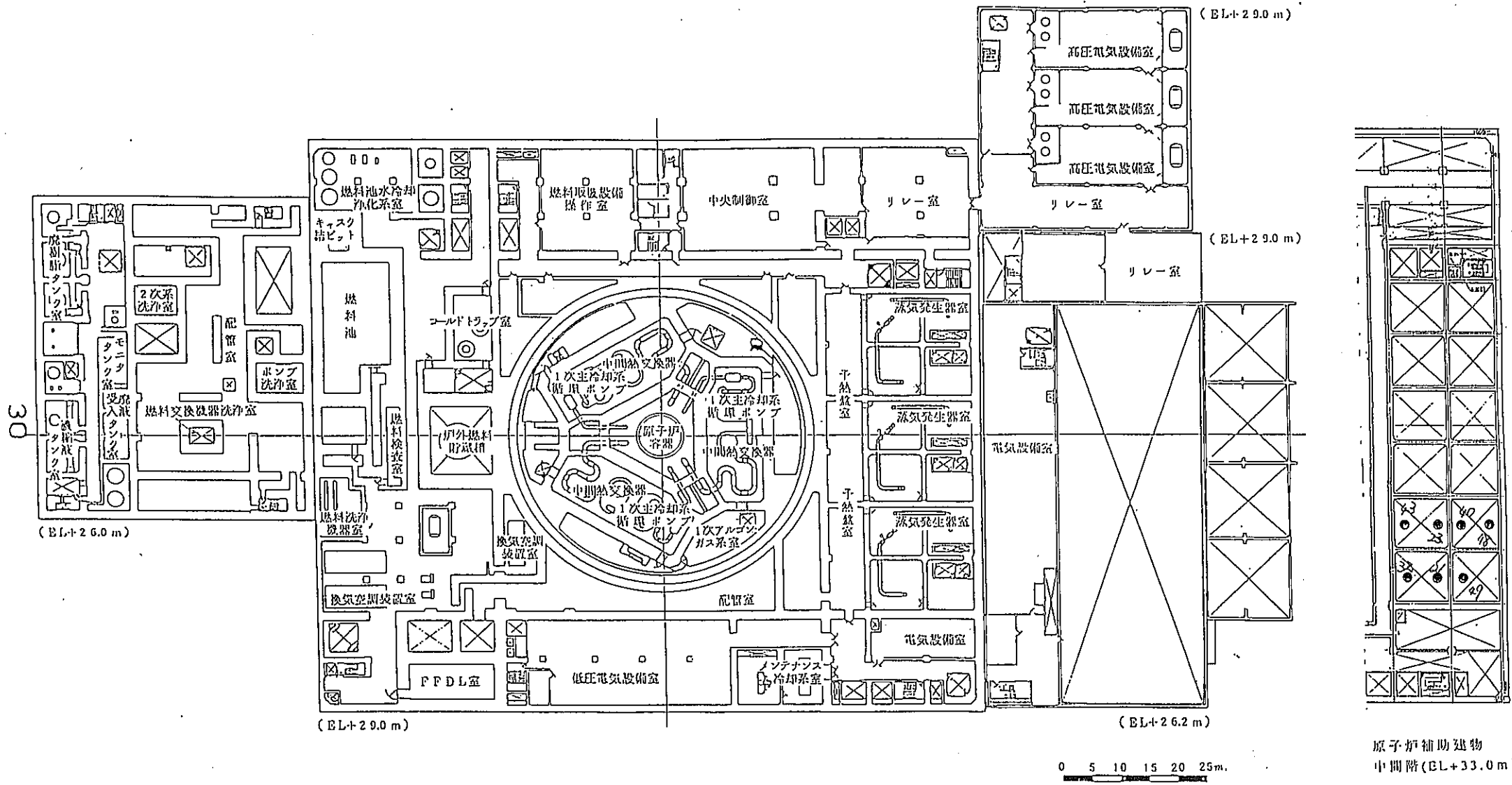
煙感知器発報位置図-4
