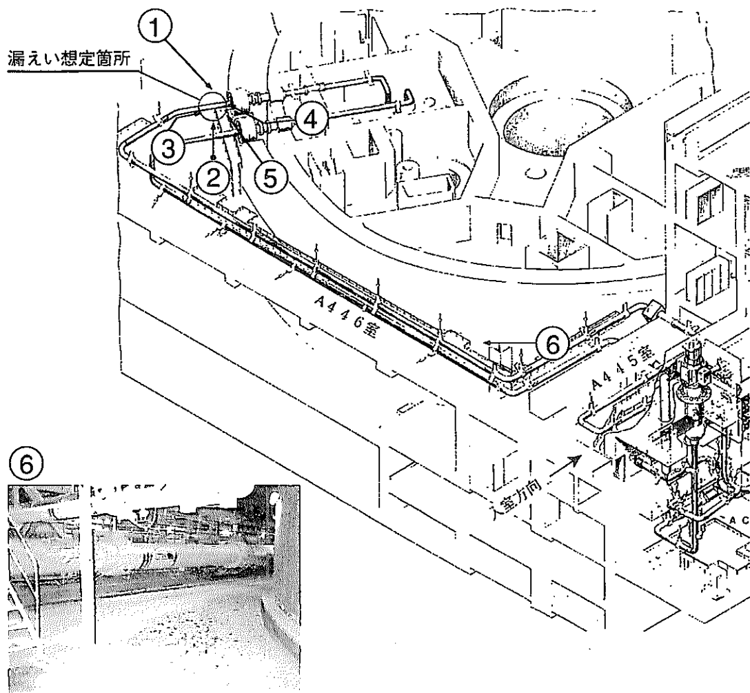
2次主冷却系 (Cループ) 状況 (2)
