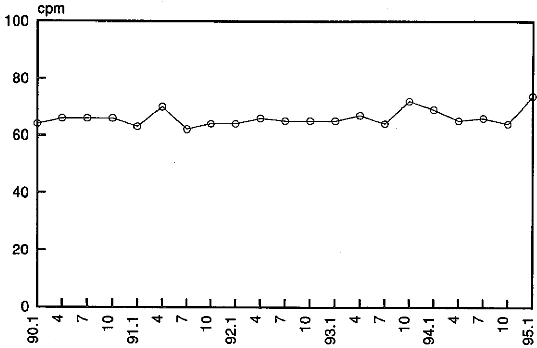
図D-19 船体表面線量 1. \beta 表面計数率
