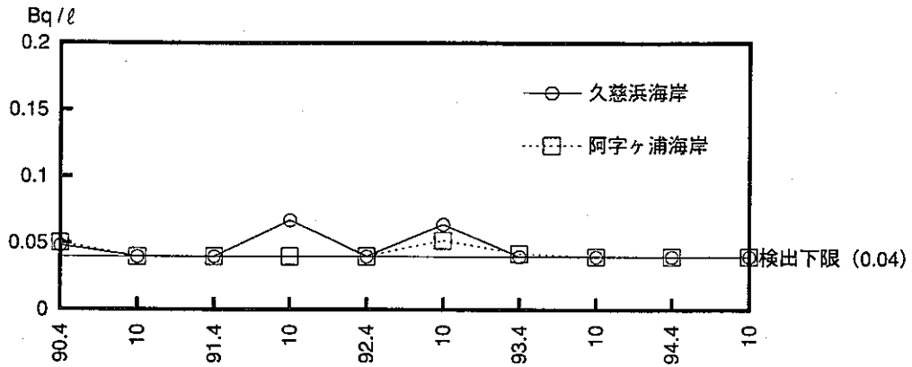
図D-15 海岸水中放射性物質濃度 イ.全β放射能
