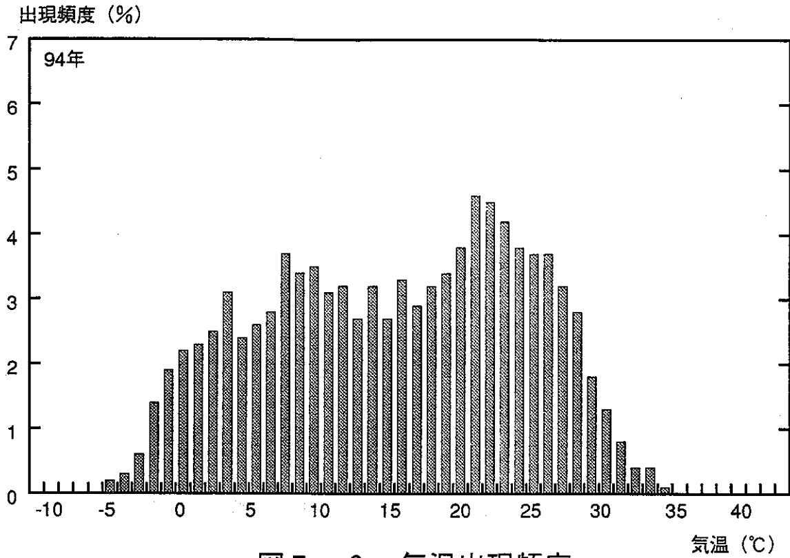
图 E - 8 气温出現頻度
