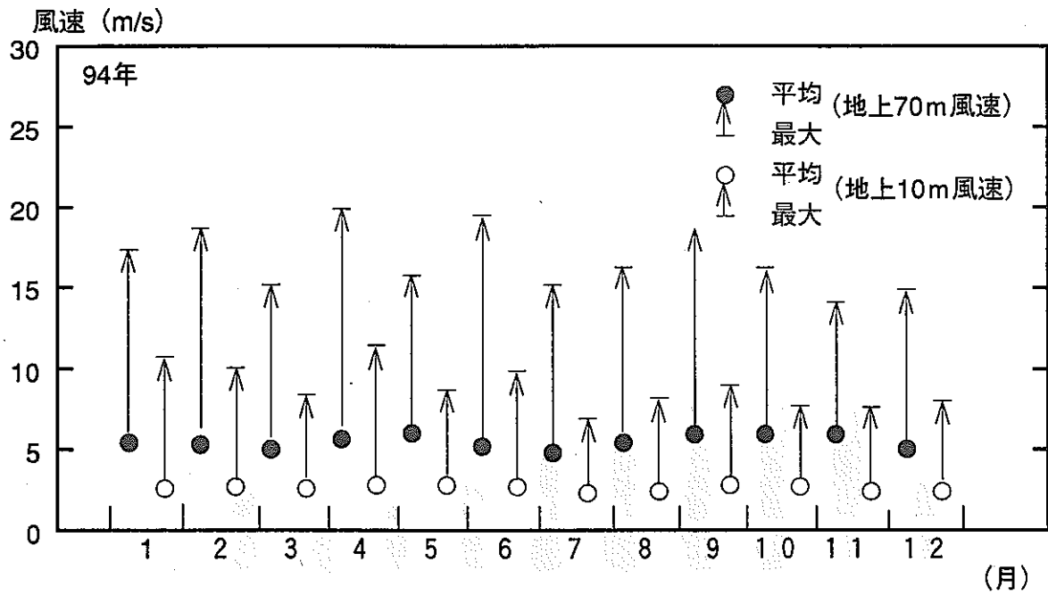
図 E - 5 月別平均風速及び最大風速
