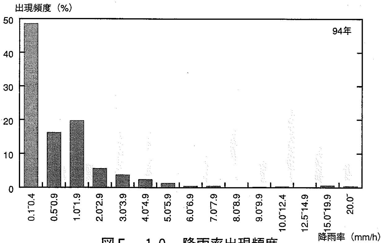
図 E - 1 0 降雨率出現頻度
