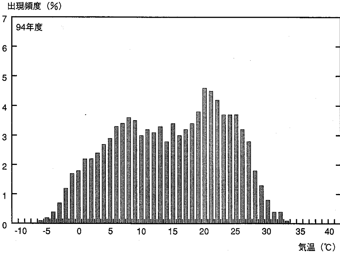
图 E - 8 气温出現頻度
