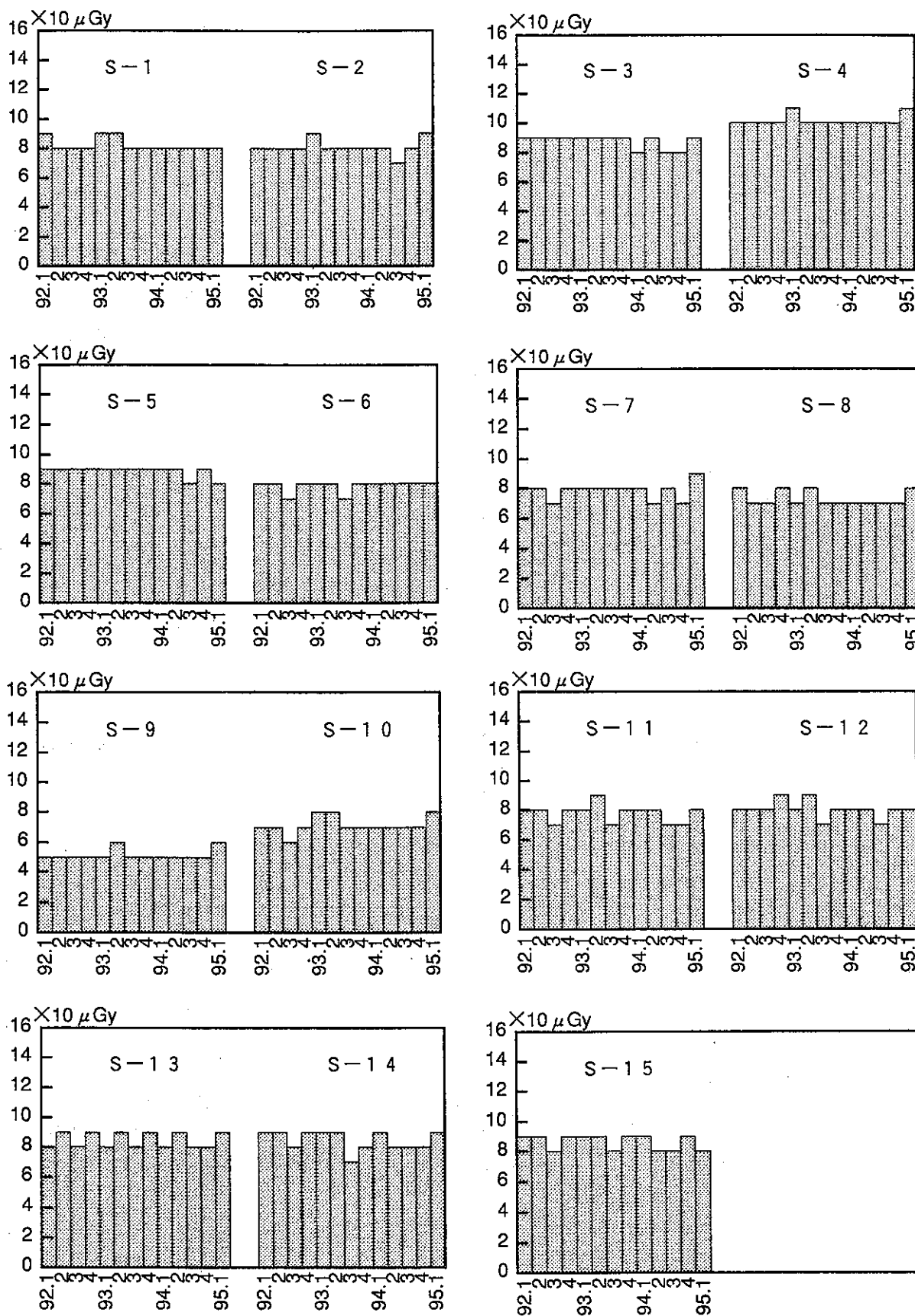
図D-2 空間γ線(積算線量) (続) □. 周辺監視区域内
