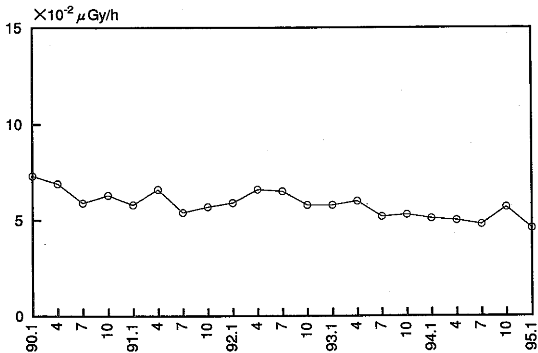
ロ. \gamma 表面線量率
