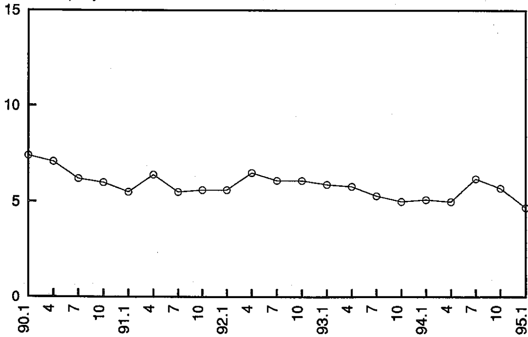
□. \gamma 表面線量率 \times 10^{-2} \mu\text{Gy/h}
