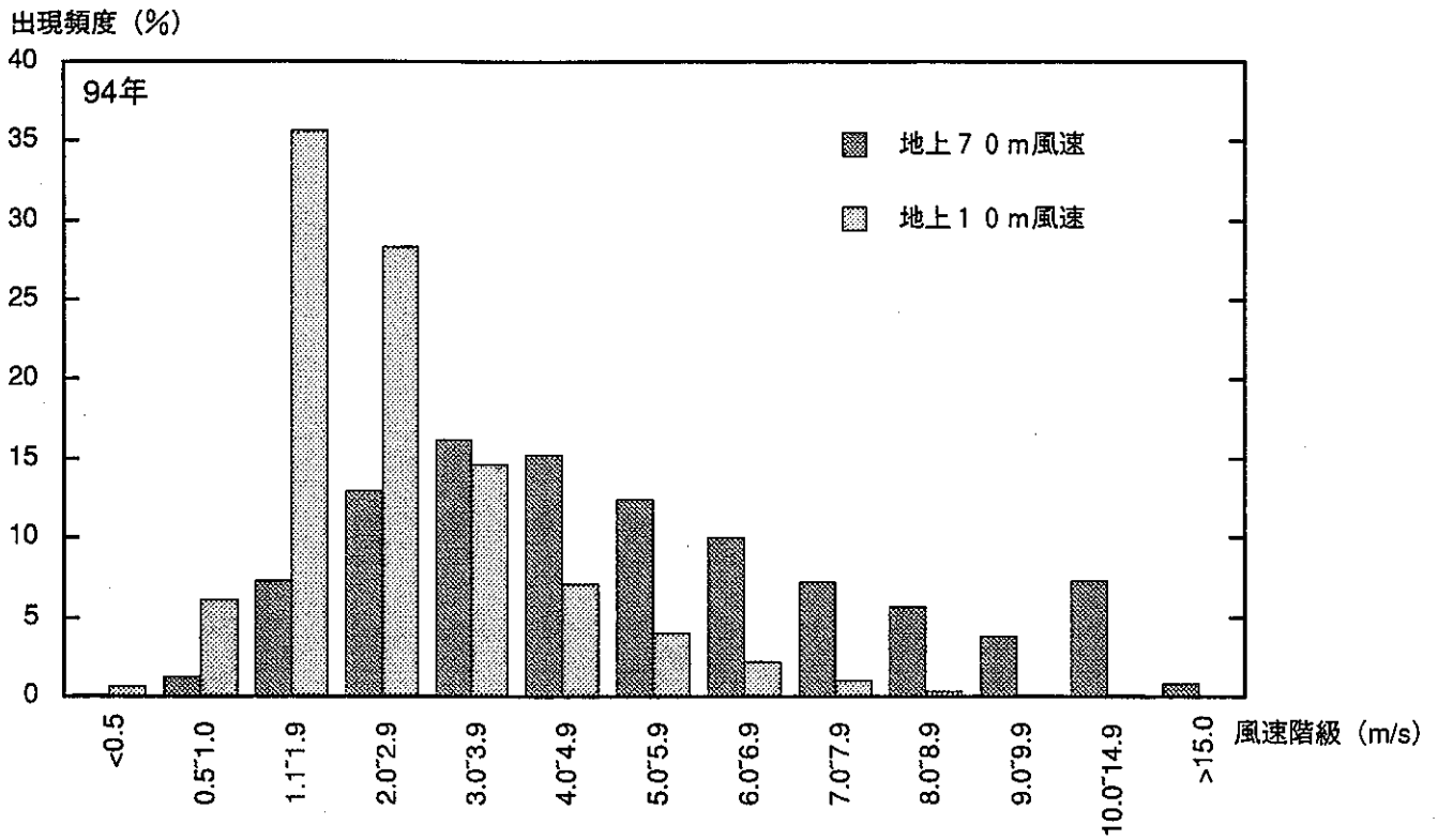
圖 E-6 風速階級出現頻度
