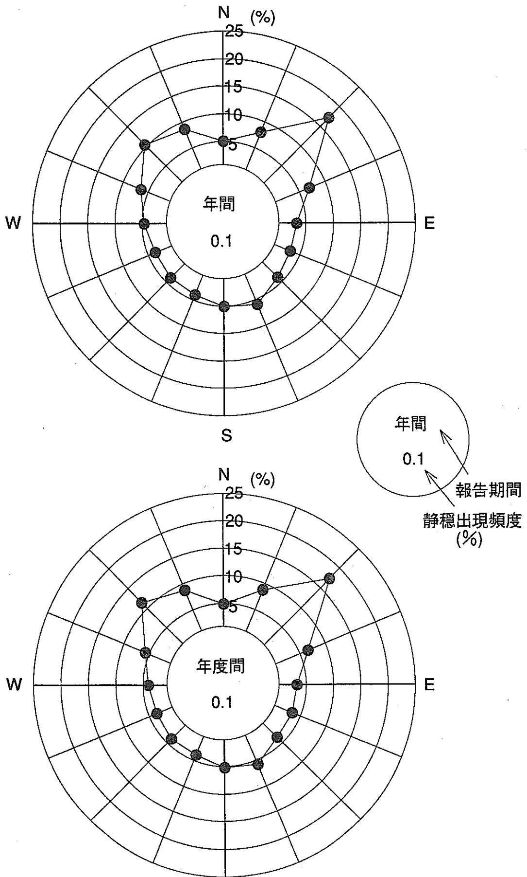
図E—1 地上70m風向出現頻度 (%)
