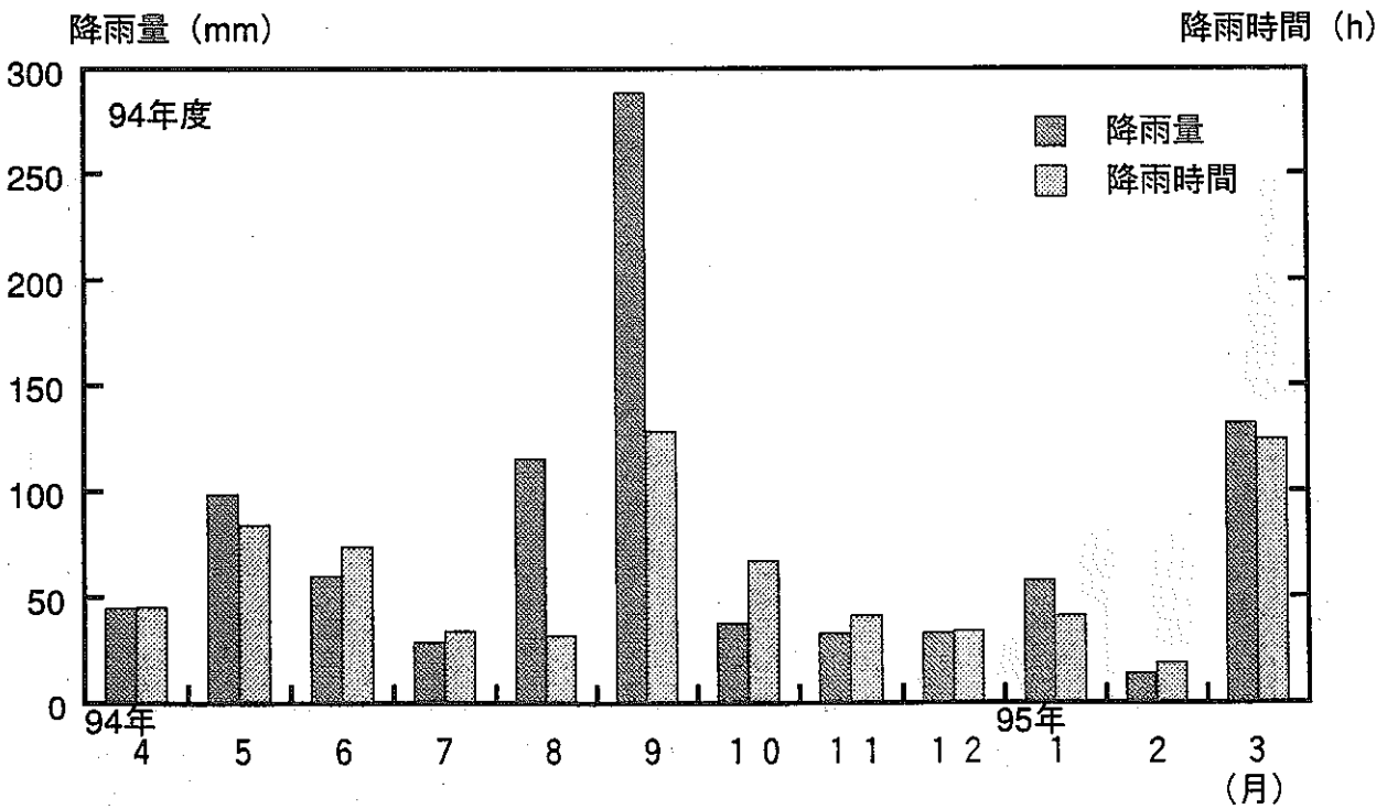
図 E-9 月間降雨量及び降雨時間
