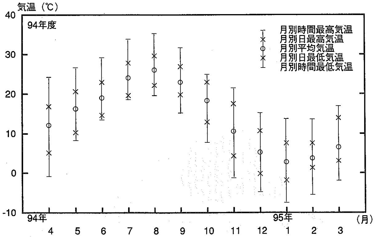
図 E - 7 月別平均・最高・最低気温
