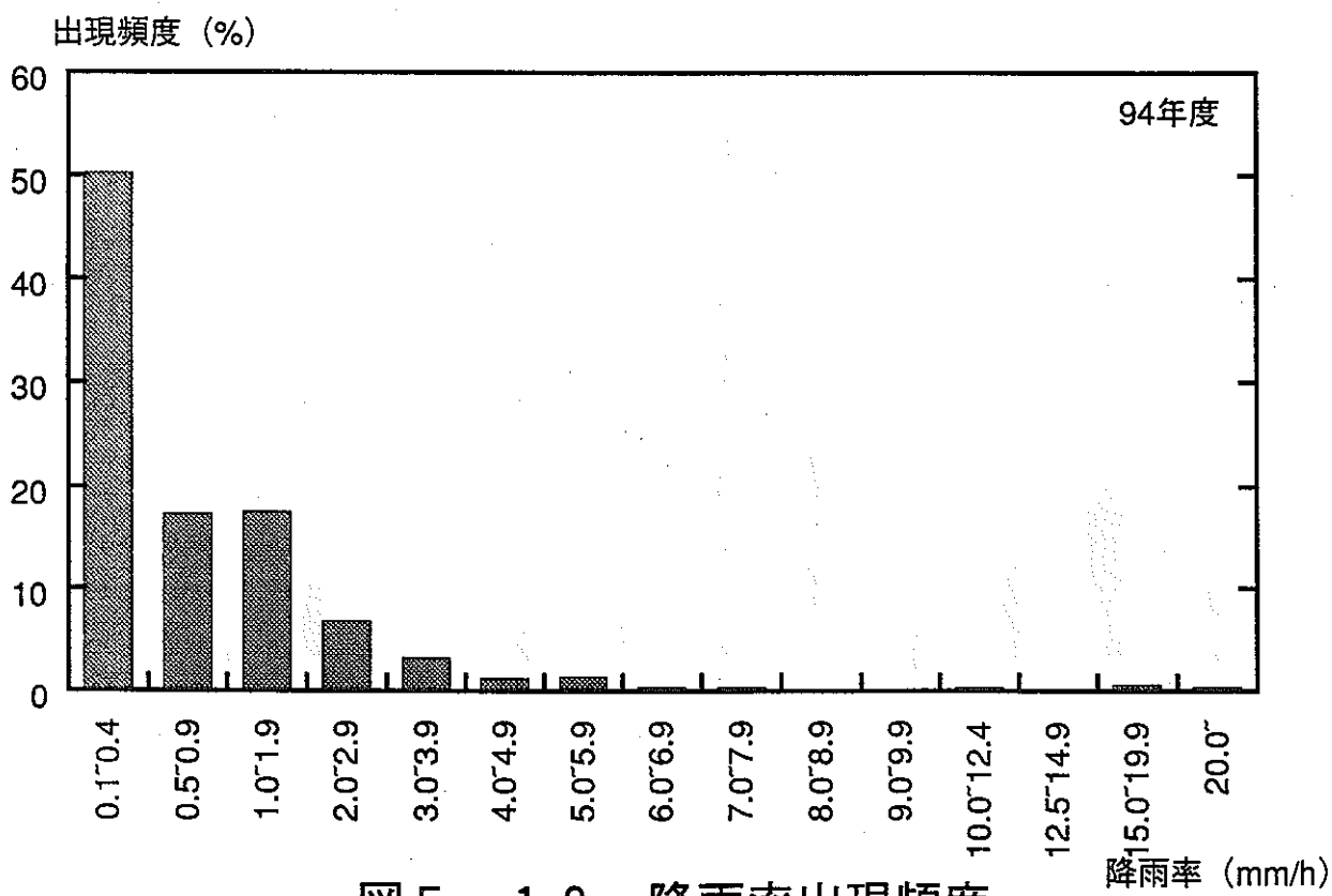
図 E - 1 0 降雨率出現頻度
