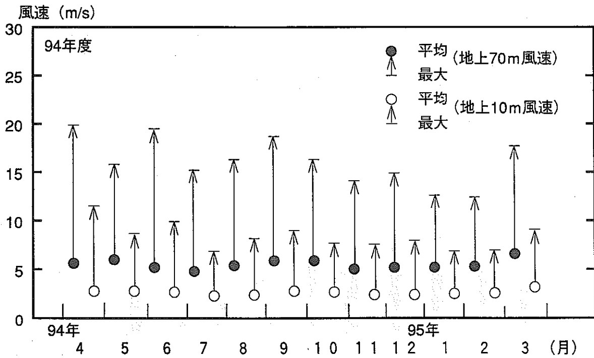
図 E - 5 月別平均風速及び最大風速
