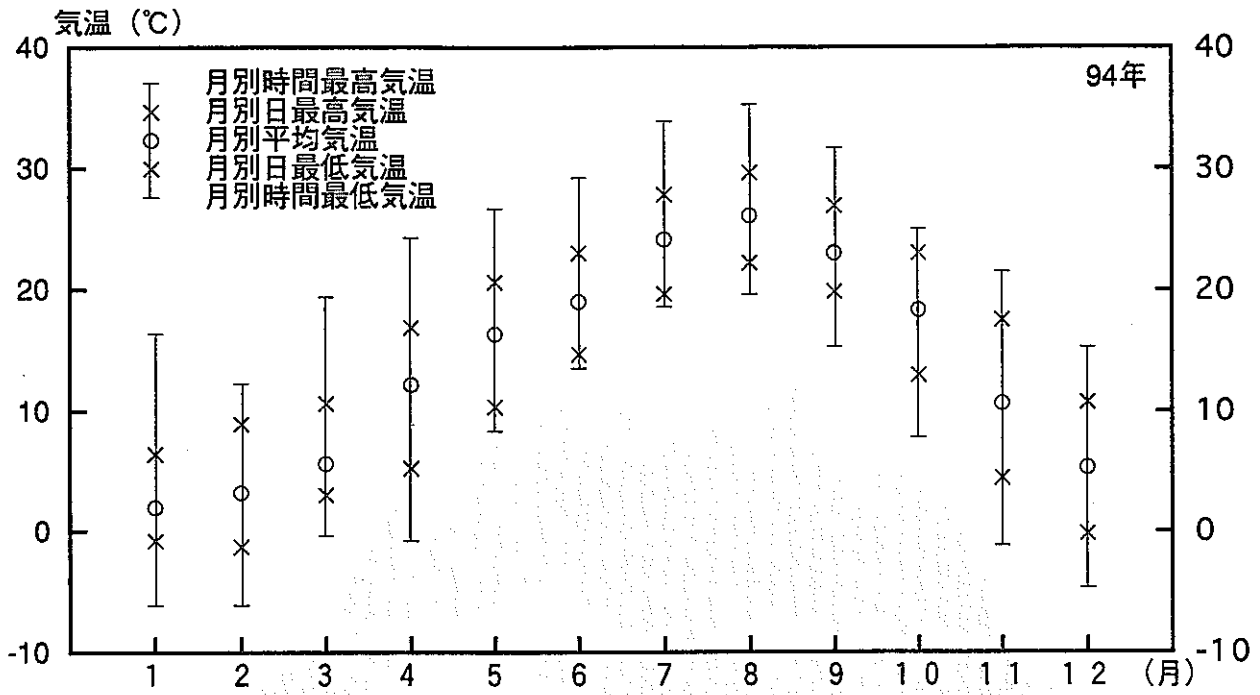
図 E - 7 月別平均・最高・最低気温
