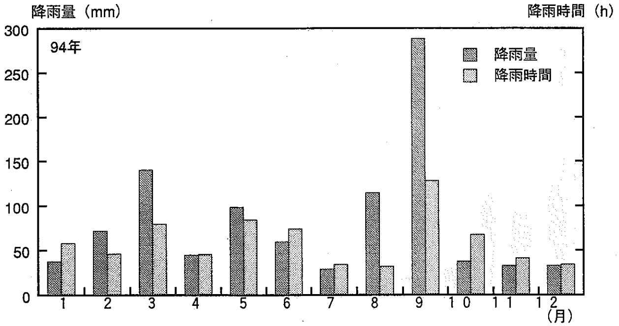
図 E-9 月間降雨量及び降雨時間
