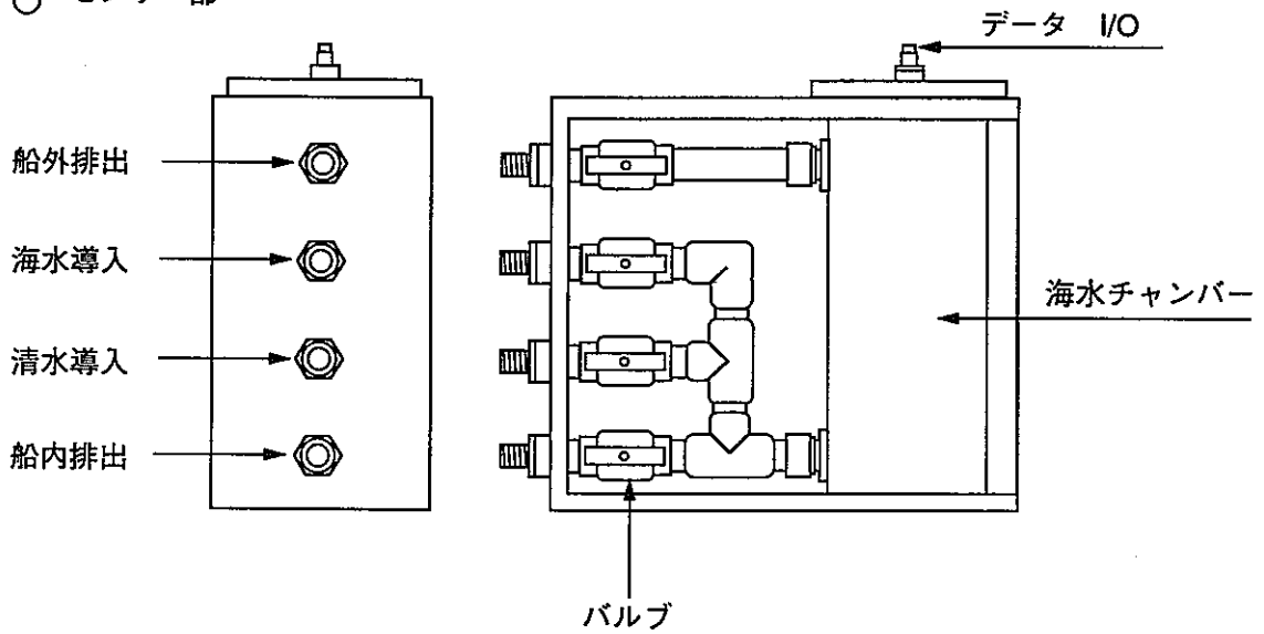
図2.1-2 水温・塩分計 系統図
