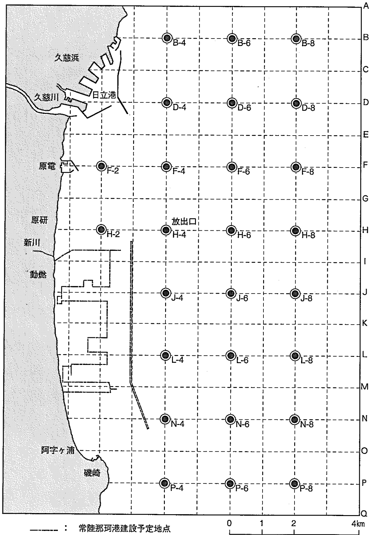
図2.1-1 水平観測地点図
