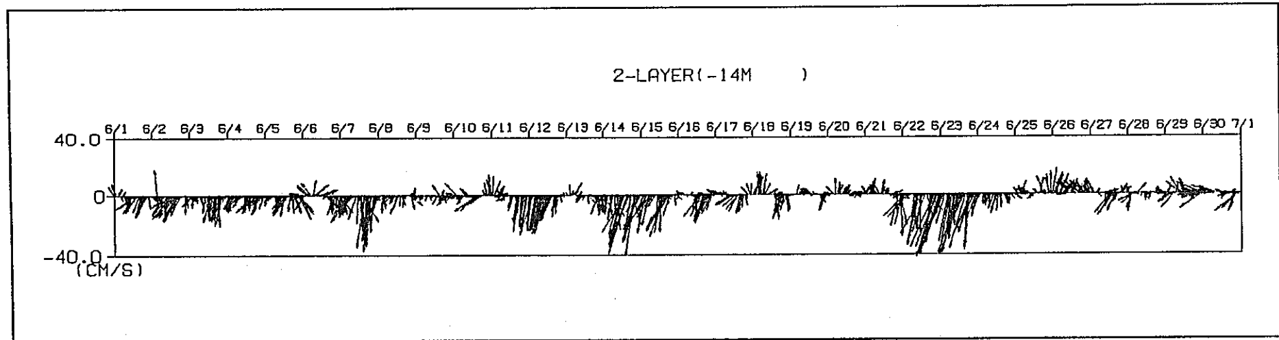
流向・流速ベクトル (海面下14m) 1995 / 6 / 1 0 : 00 ~ 6 / 30 23 : 55
