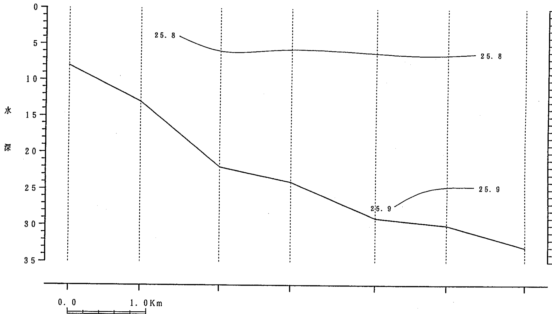
鉛直断面図
