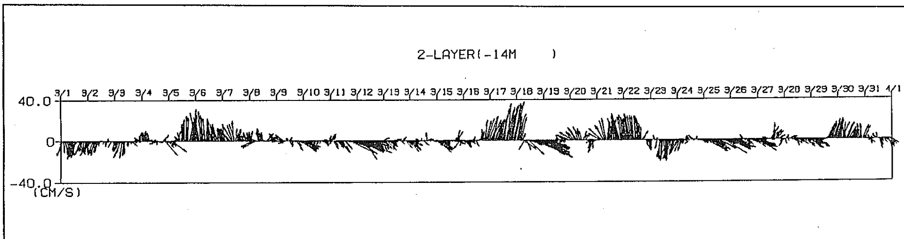
流向・流速ベクトル (海面下14m) 1995 / 3 / 1 0:00 ~ 3 / 31 23:55
