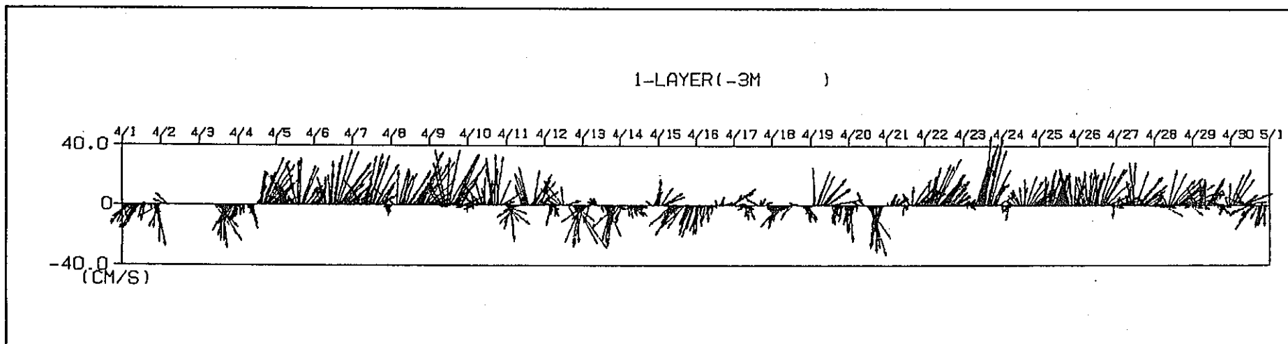
流向・流速ベクトル (海面下3m) 1995 / 4 / 1 0:00 ~ 4 / 30 23:55
