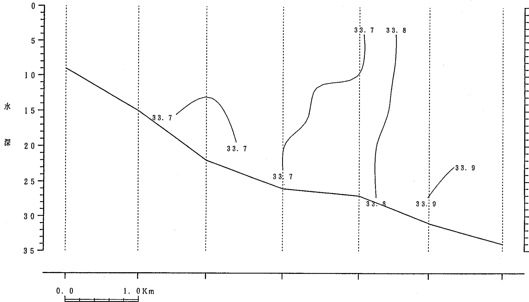
鉛直断面図
