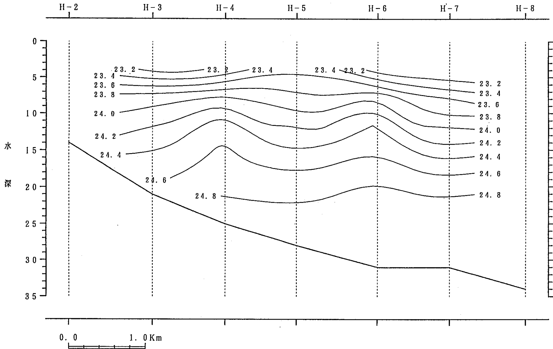
鉛直断面図
