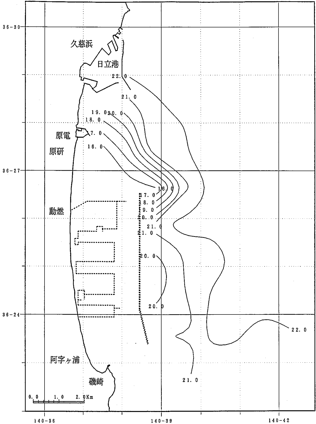
東海沖水温水平調査
