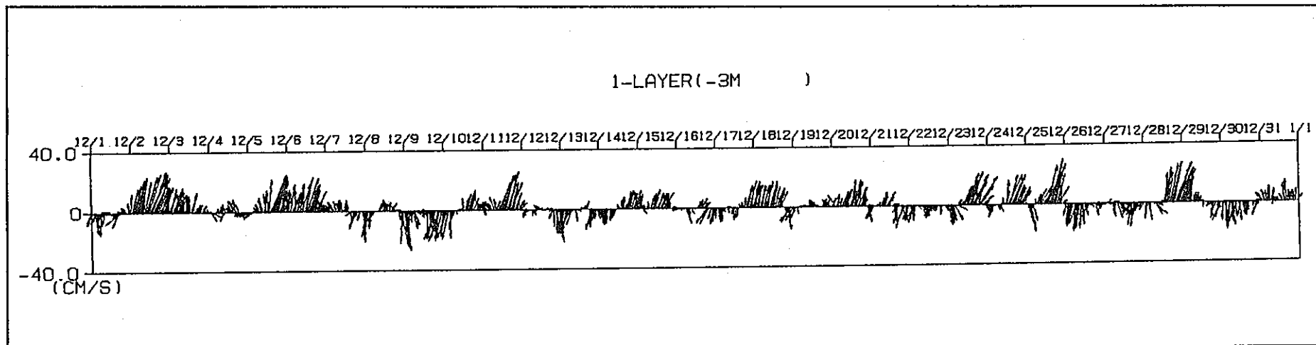
流向・流速ベクトル (海面下3m) 1995 / 12 / 1 0 : 00 ~ 12 / 31 23 : 55
