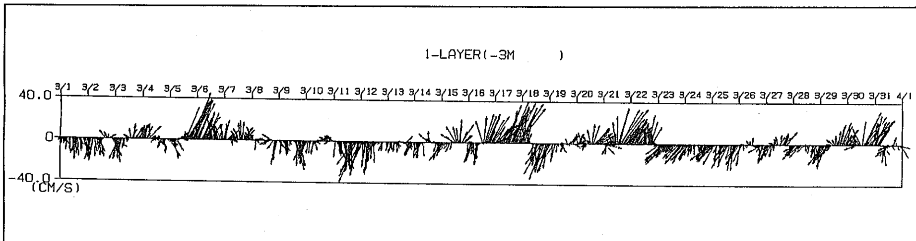
流向・流速ベクトル (海面下3m) 1995 / 3 / 1 0:00 ~ 3 / 31 23:55
