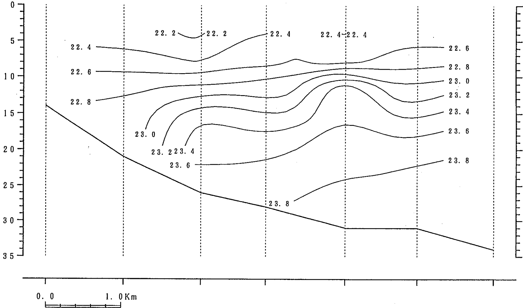
鉛直断面図
