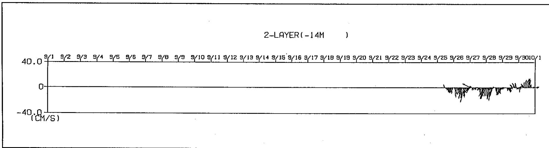
流向・流速ベクトル (海面下14m) 1995 / 9 / 1 0:00 ~ 9 / 30 23:55
