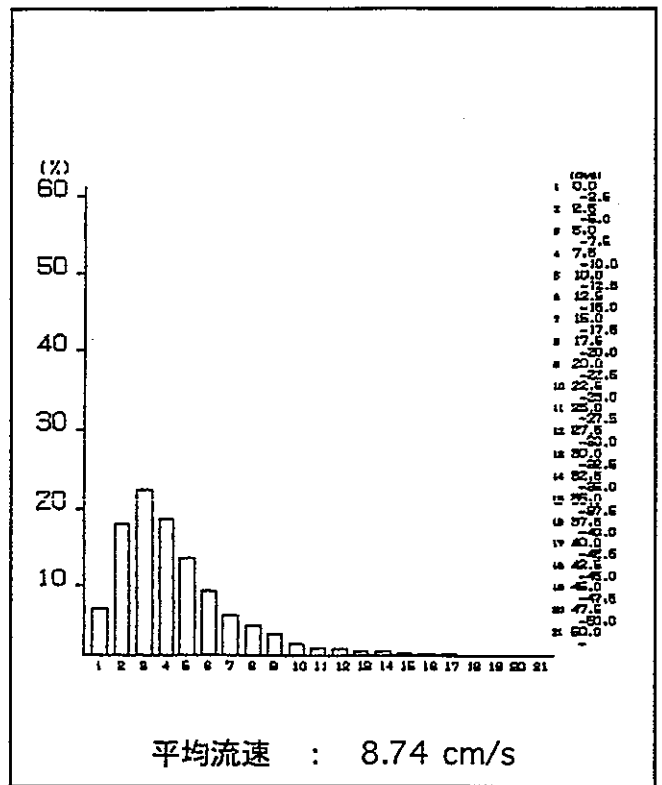
夏季流速分布 (海面下14m) 1995/6/1 0:00 ~ 8/31 23:55
