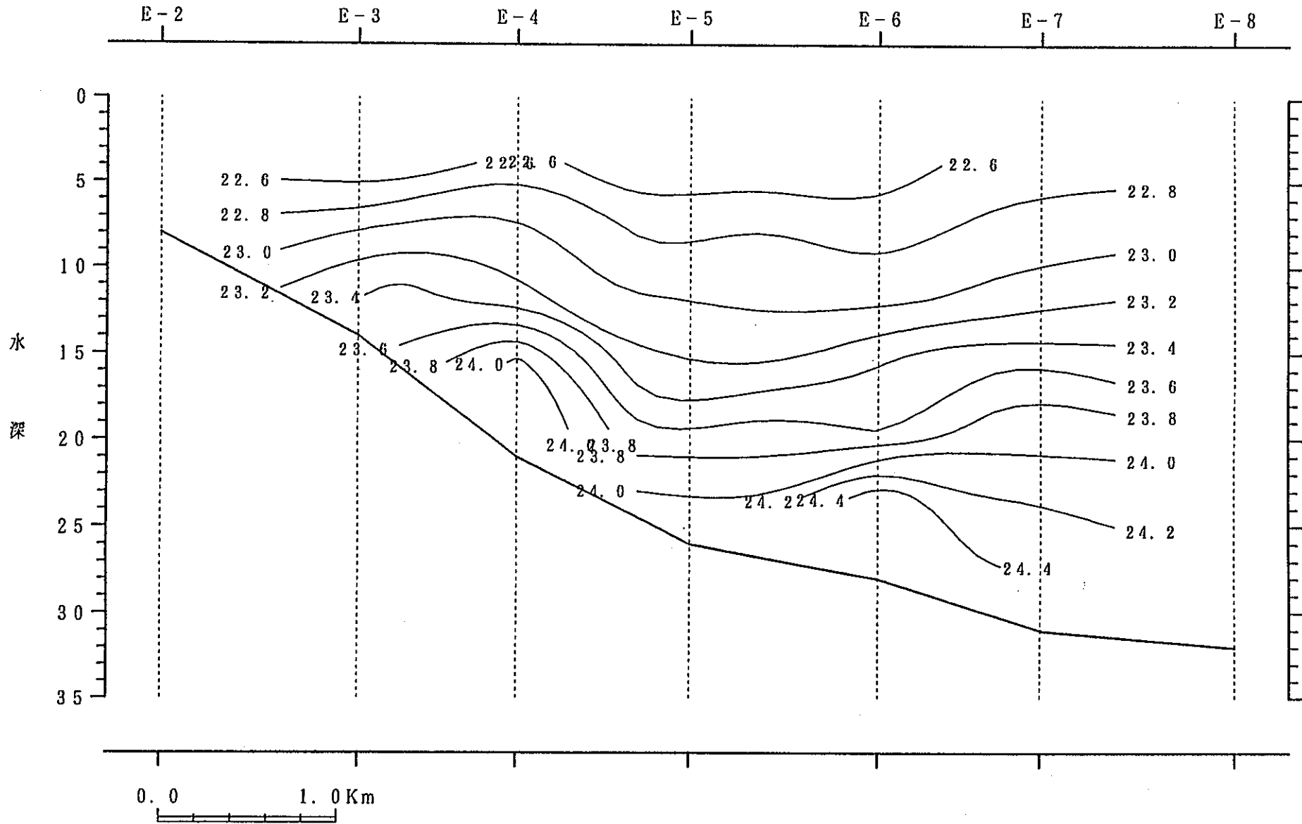
鉛直断面図
