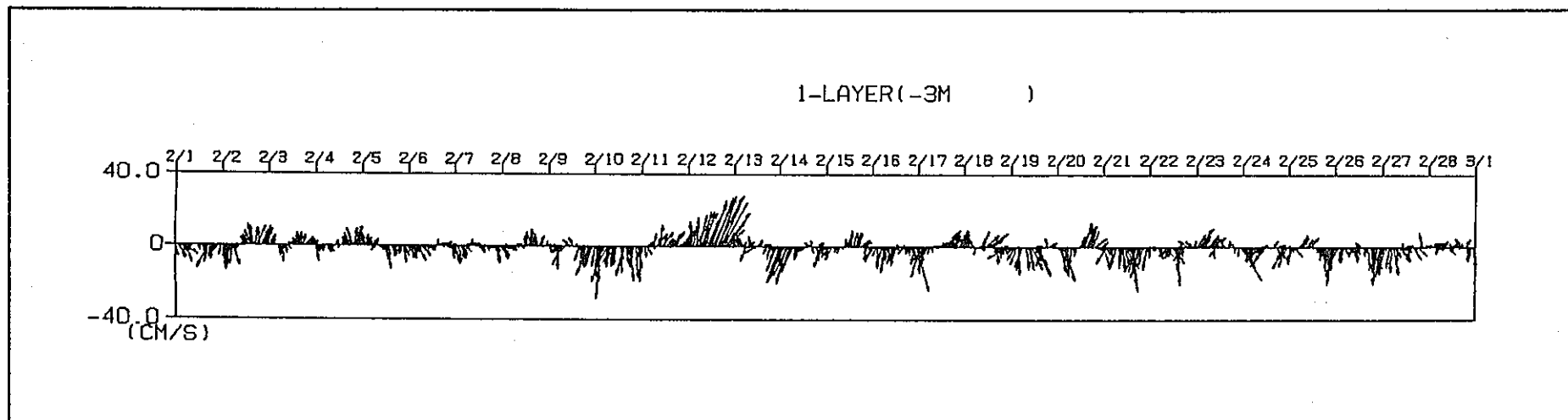
流向・流速ベクトル (海面下3m) 1995 / 2 / 1 0:00 ~ 2 / 28 23:55
