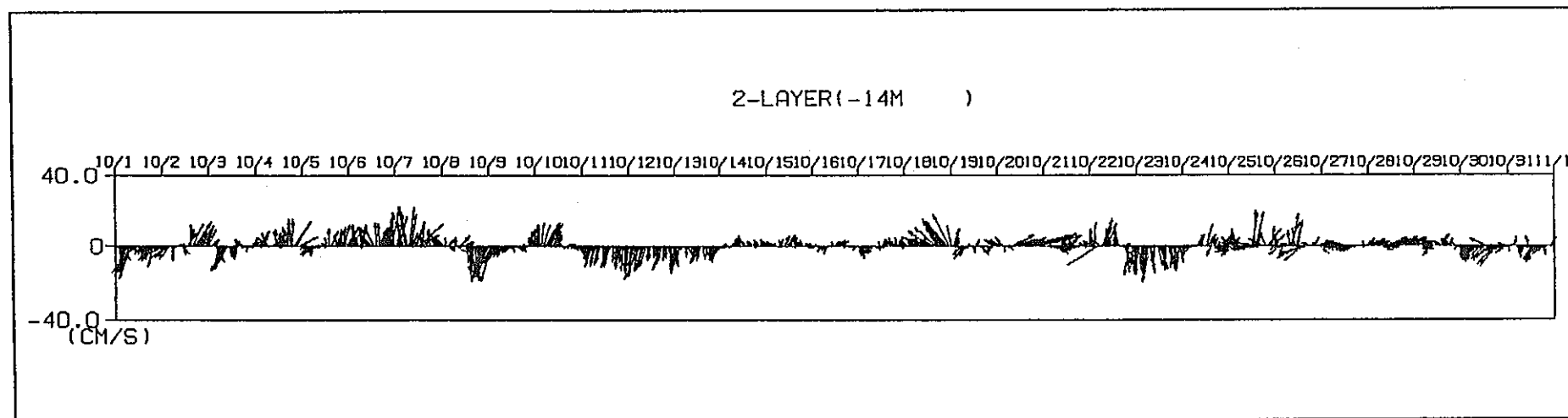
流向・流速ベクトル (海面下14m) 1995 / 10 / 1 0:00 ~ 10 / 31 23:55
