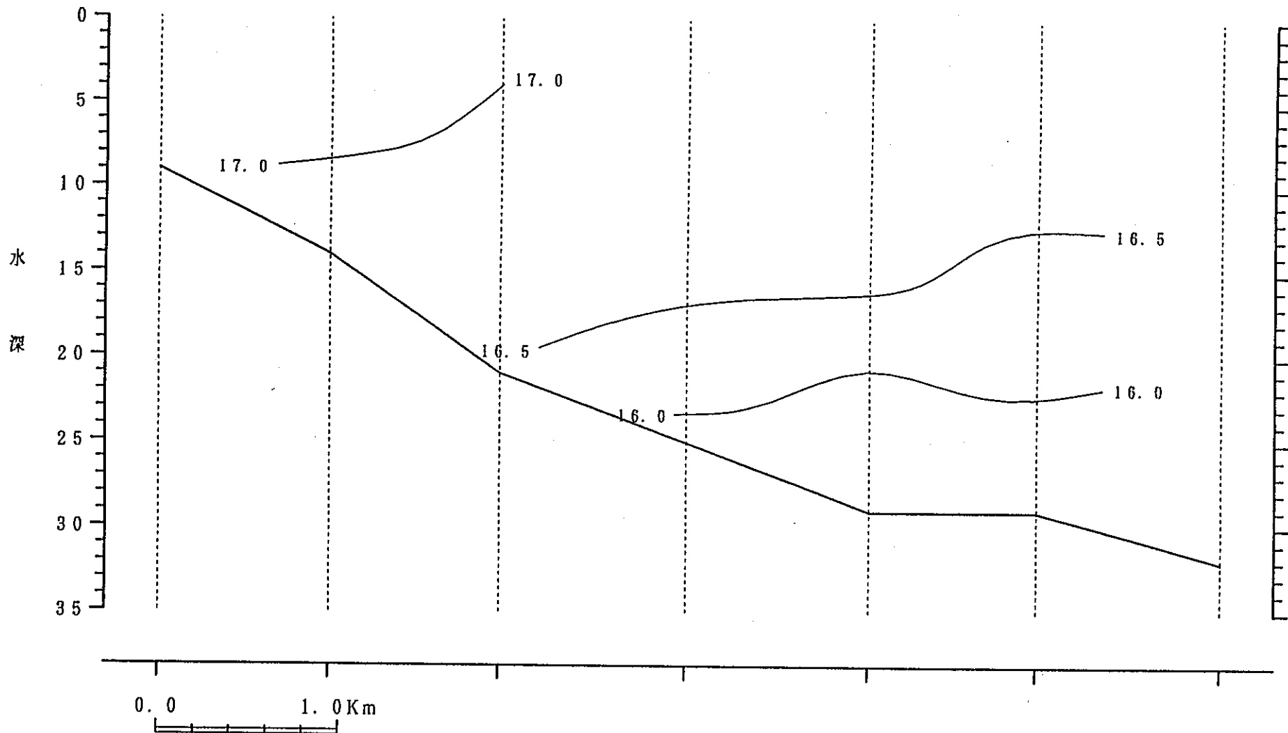
鉛直断面図
