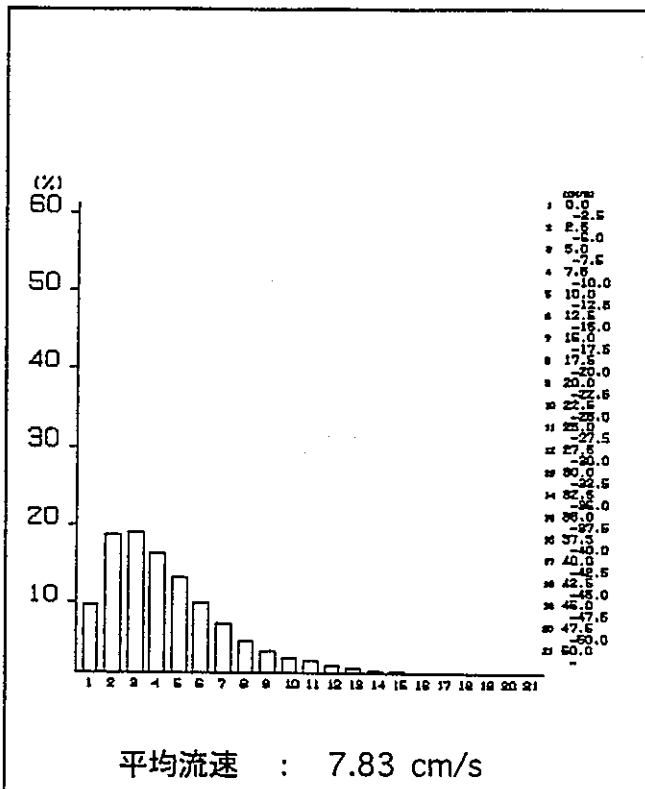
秋季流速分布 (海面下3m)
