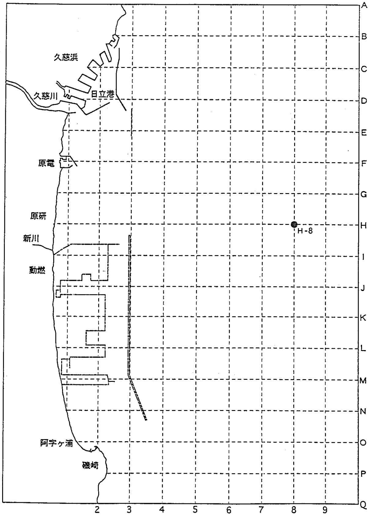
図 II-7.2-2 Tc-99 測定用の試料（海水）採取位置
