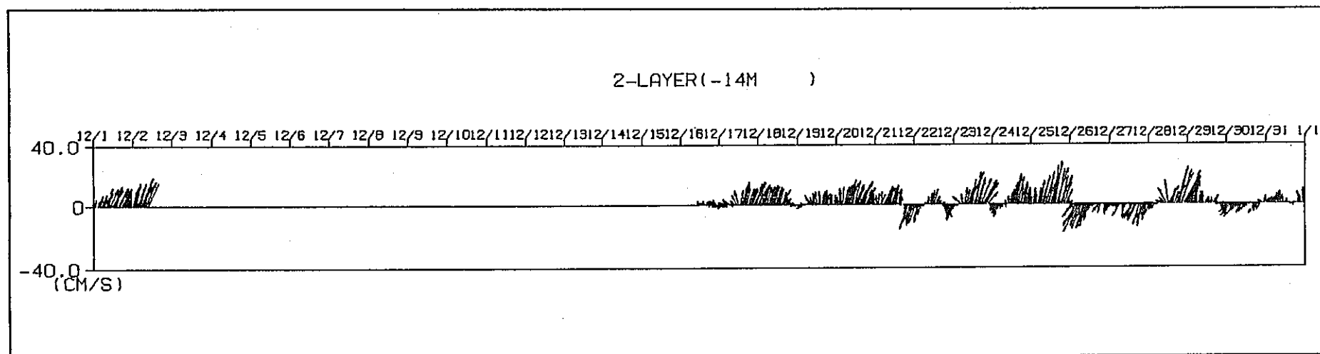
流向・流速ベクトル (海面下14m) 1995 / 12 / 1 0 : 00 ~ 12 / 31 23 : 55
