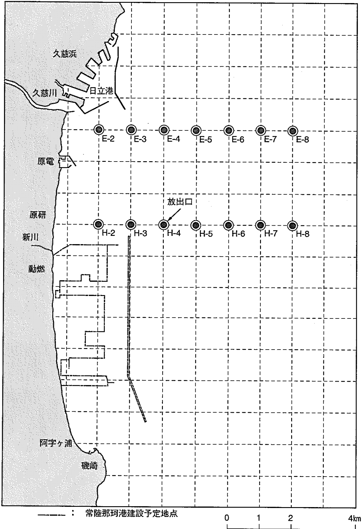
図3.1-1 鉛直観測地点図
