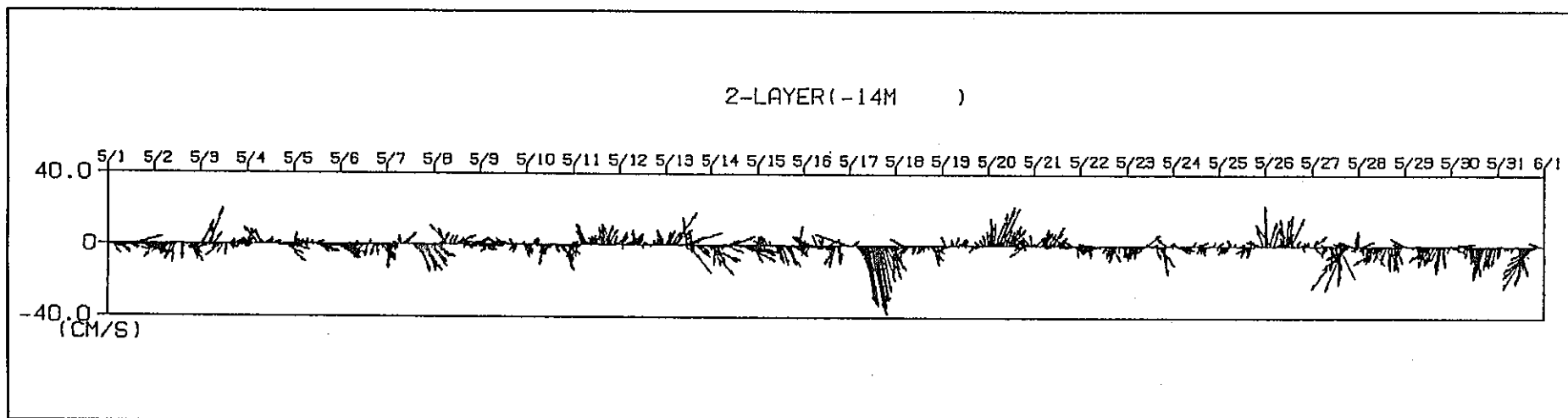
流向・流速ベクトル (海面下14m) 1995 / 5 / 1 0:00 ~ 5 / 31 23:55
