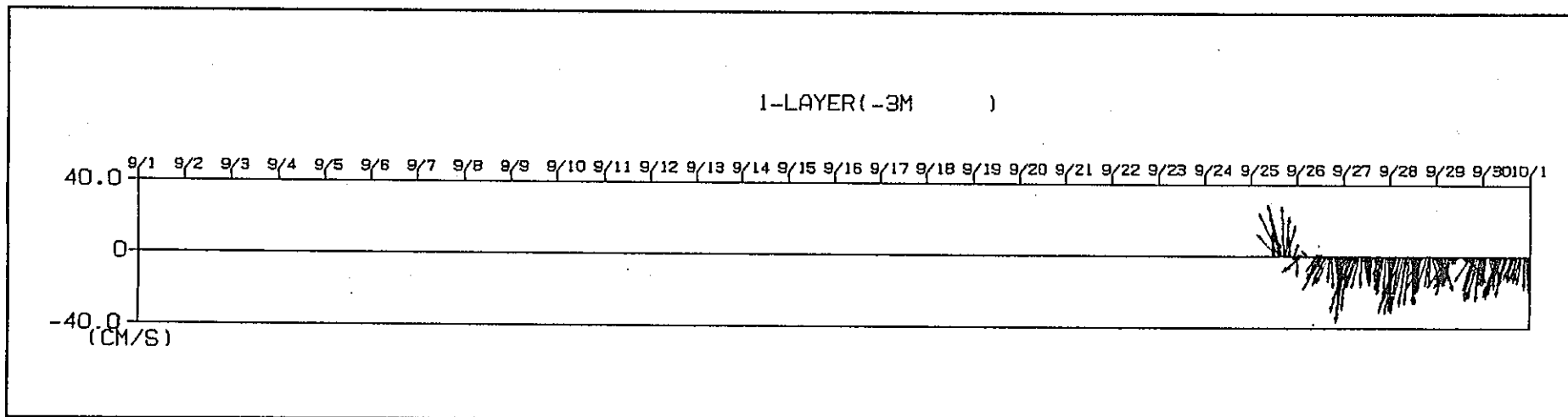
流向・流速ベクトル (海面下3m) 1995 / 9 / 1 0:00 ~ 9 / 30 23:55
