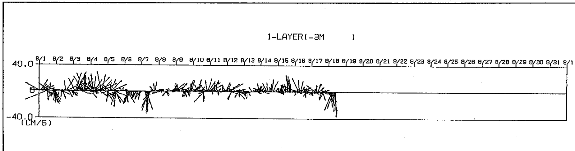
流向・流速ベクトル (海面下3m) 1995 / 8 / 1 0:00 ~ 8 / 31 23:55
