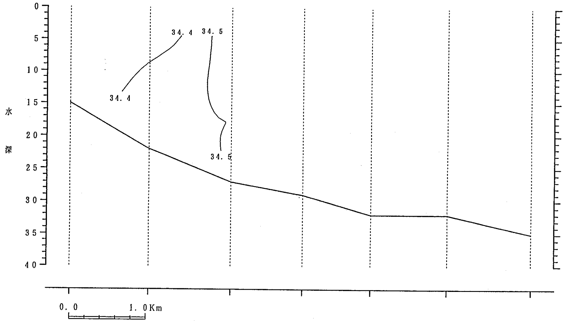
鉛直断面図
