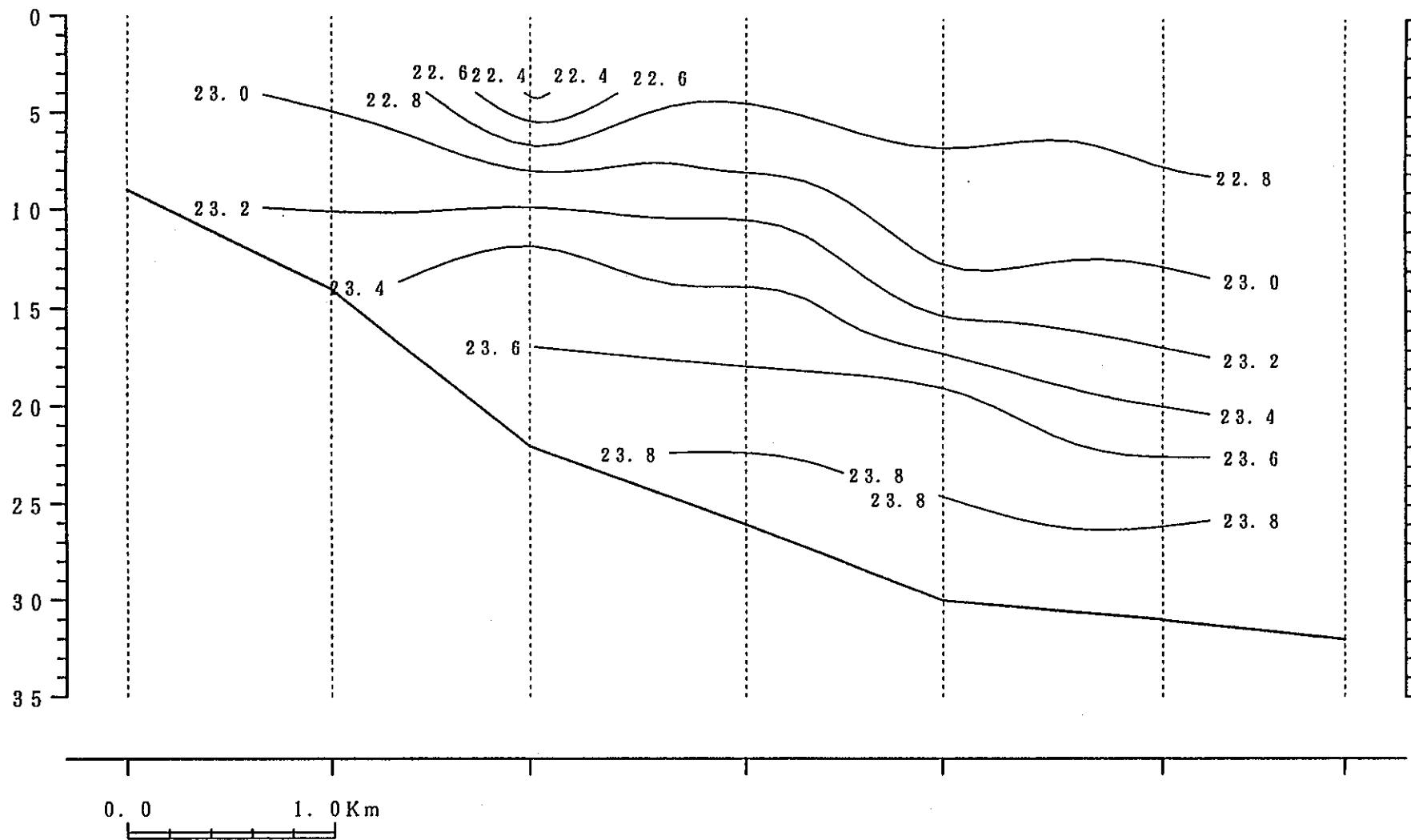
鉛直断面図
