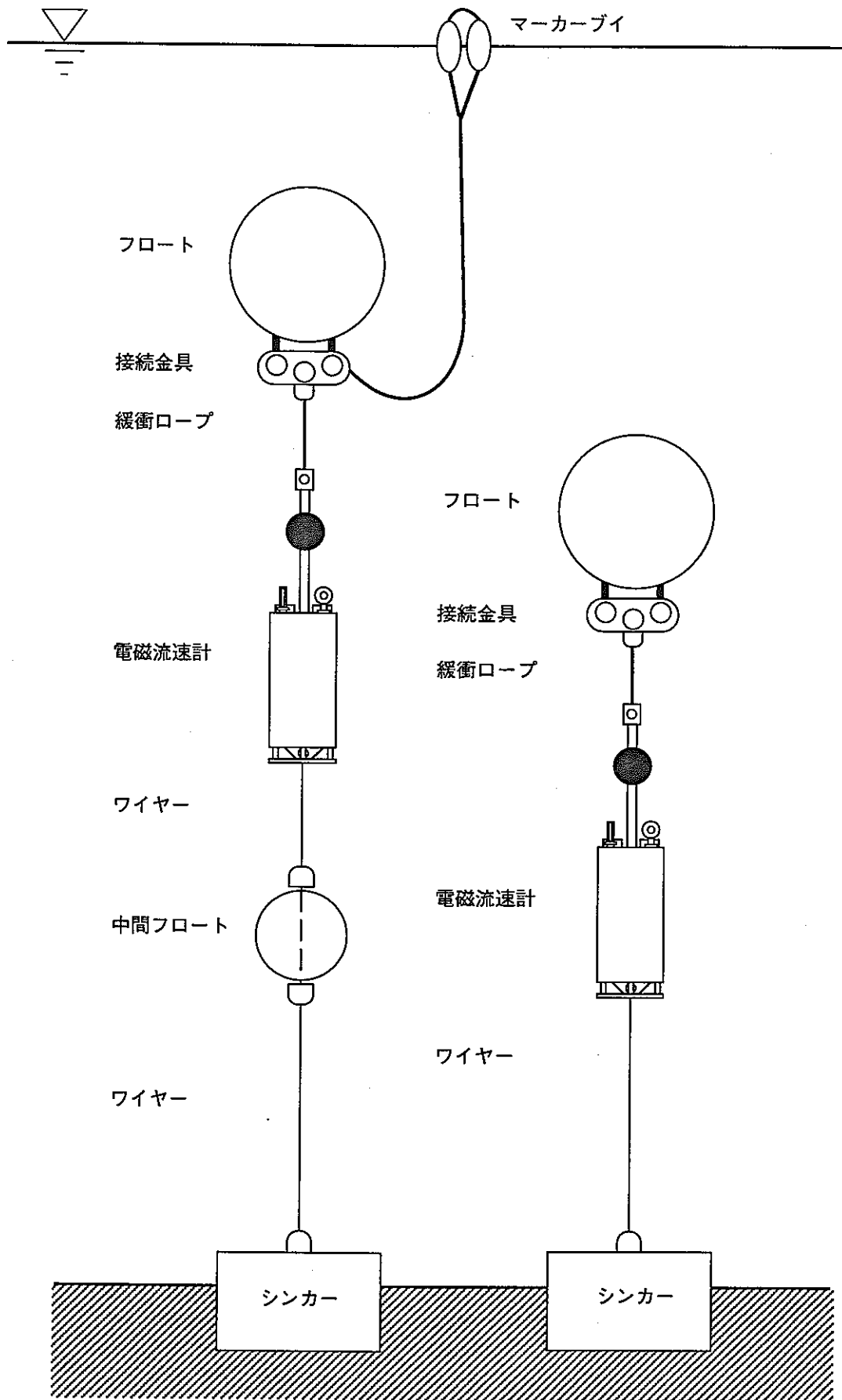
流速計設置図
