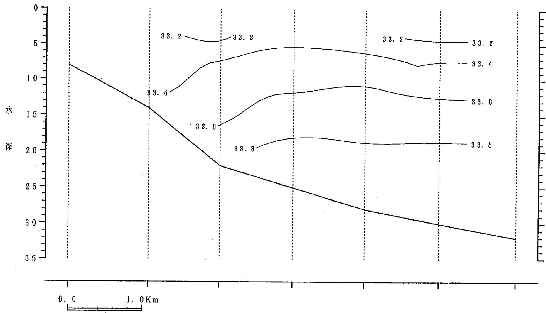
鉛直断面図
