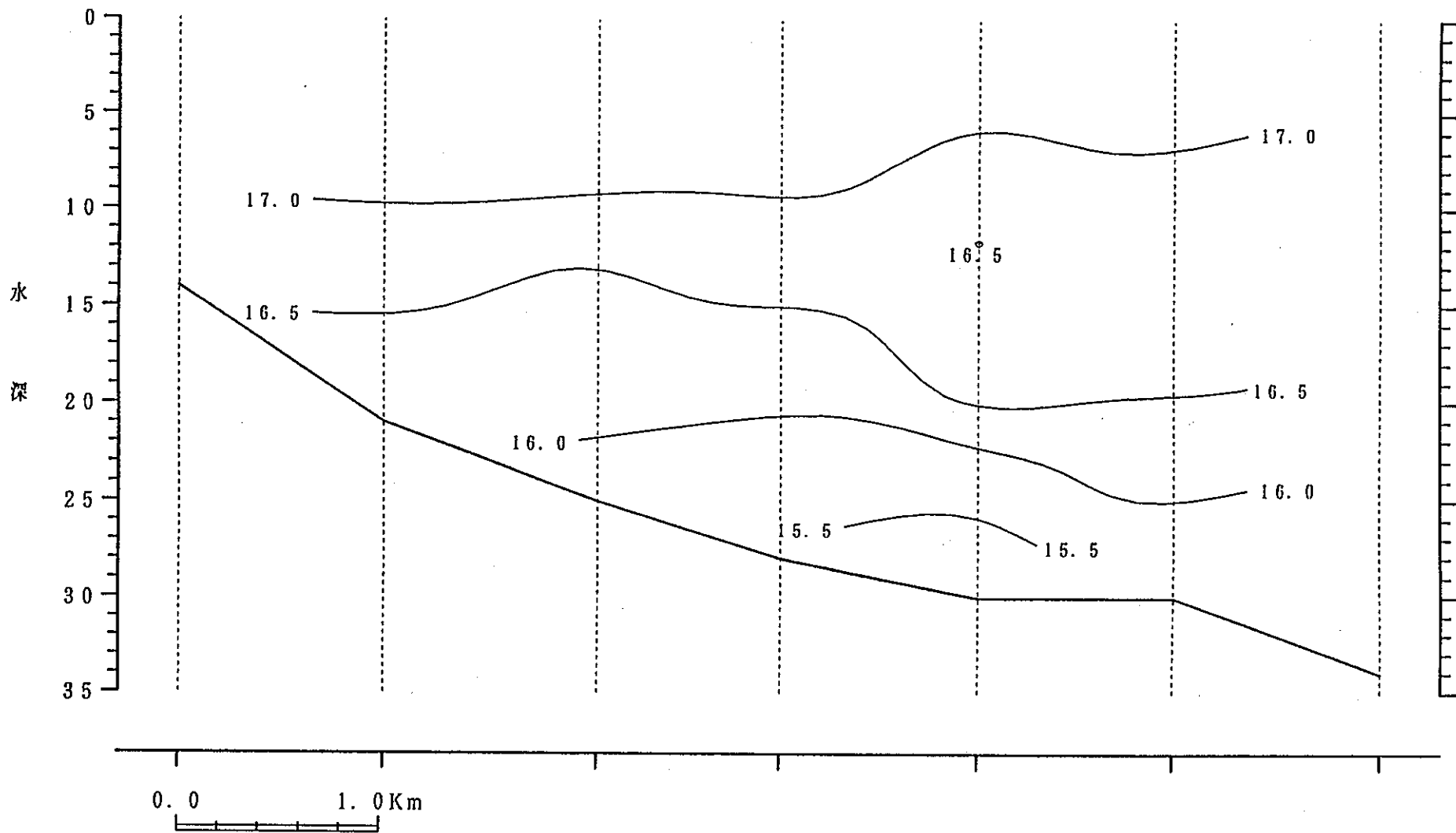
鉛直断面図
