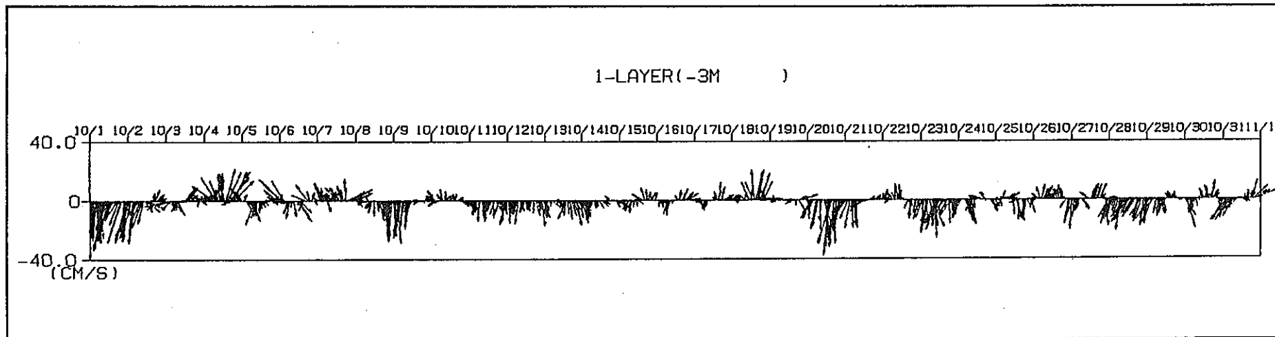
流向・流速ベクトル (海面下3m) 1995 / 10 / 1 0:00 ~ 10 / 31 23:55
