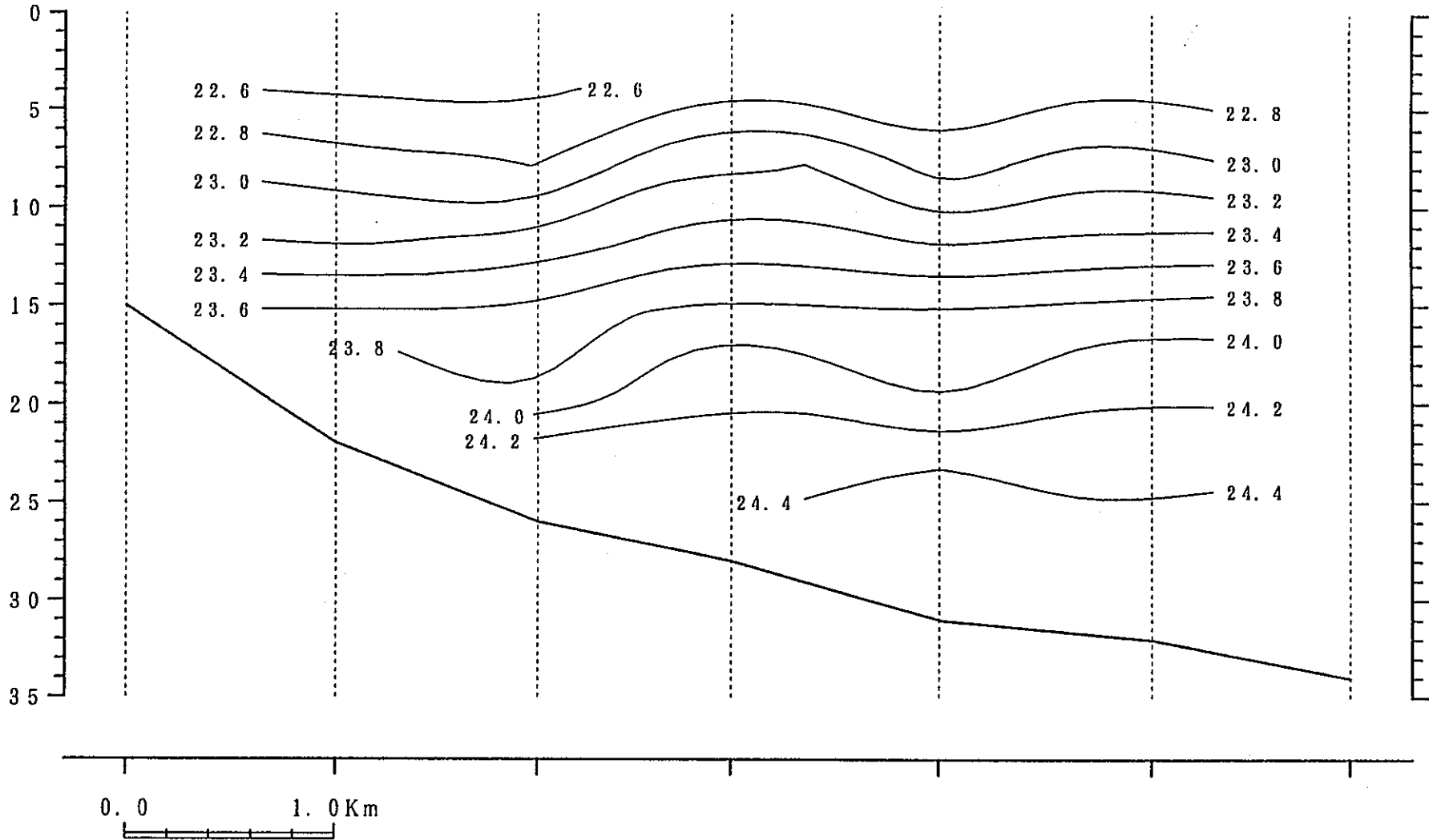
鉛直断面図
