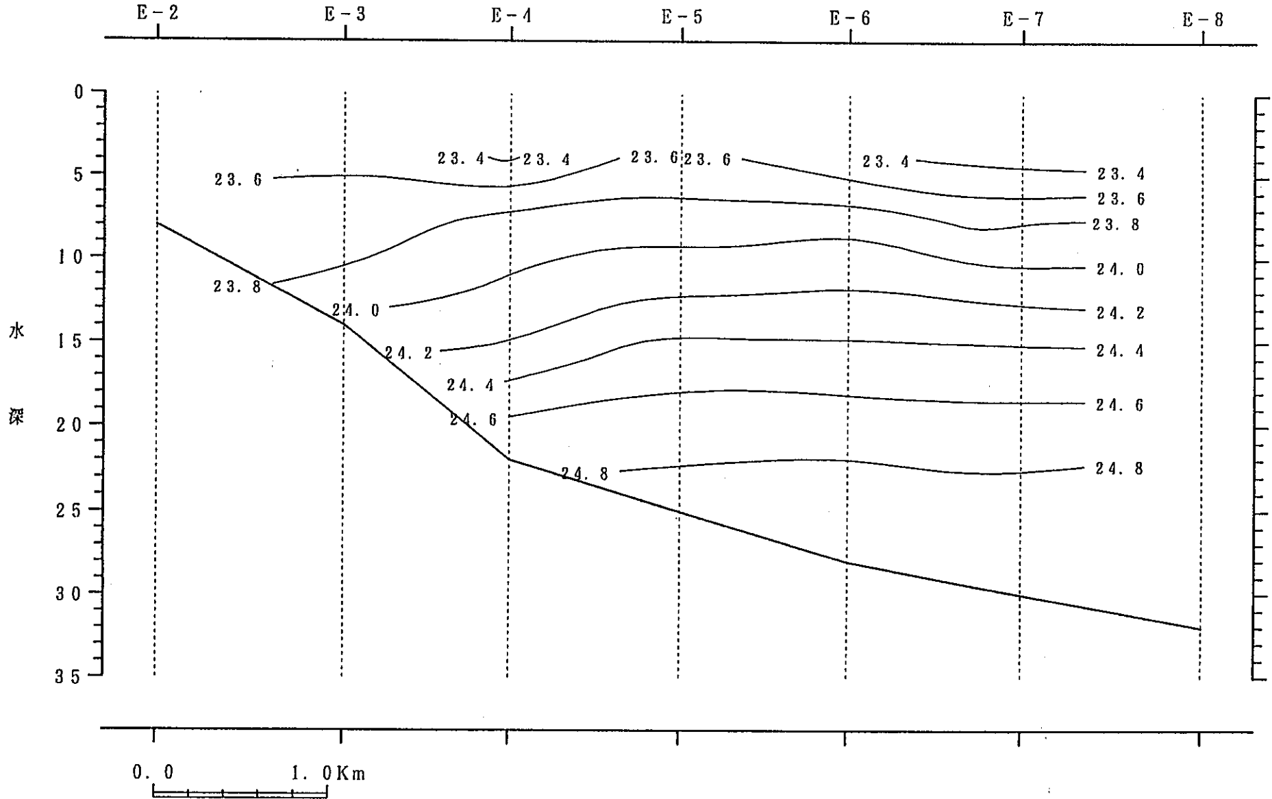
鉛直断面図
