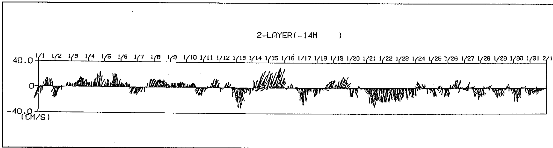
流向・流速ベクトル (海面下14m) 1995 / 1 / 1 0:00 ~ 1 / 31 23:55
