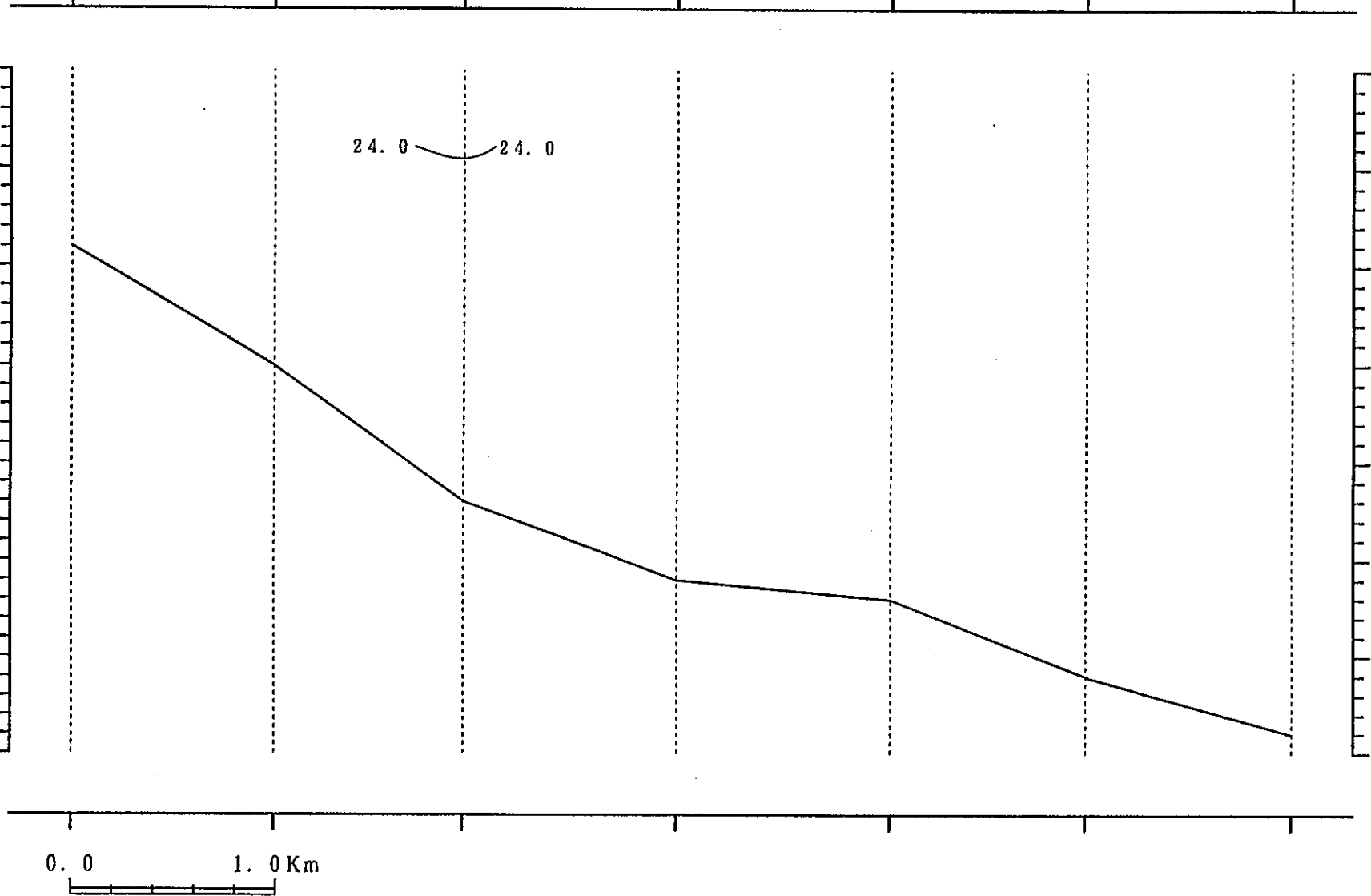
鉛直断面図
