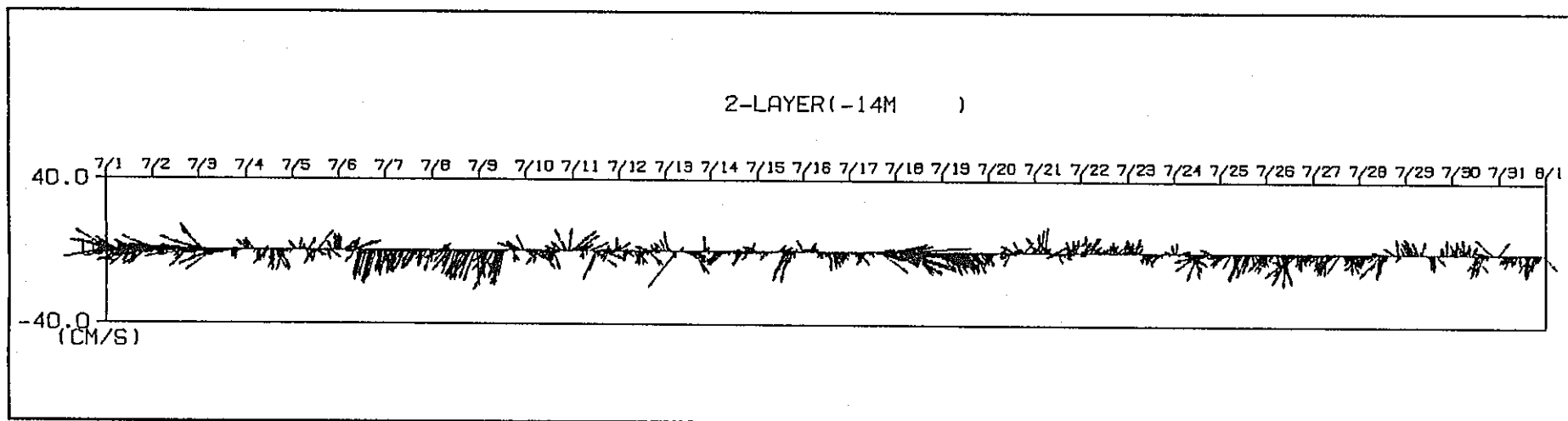
流向・流速ベクトル (海面下14m) 1995 / 7 / 1 0:00 ~ 7 / 31 23:55
