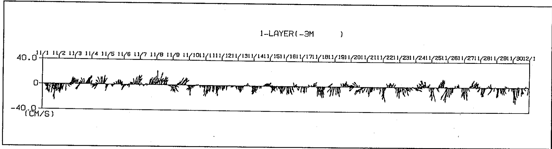
流向・流速ベクトル (海面下3m) 1995 / 11 / 1 0:00 ~ 11 / 31 23:55
