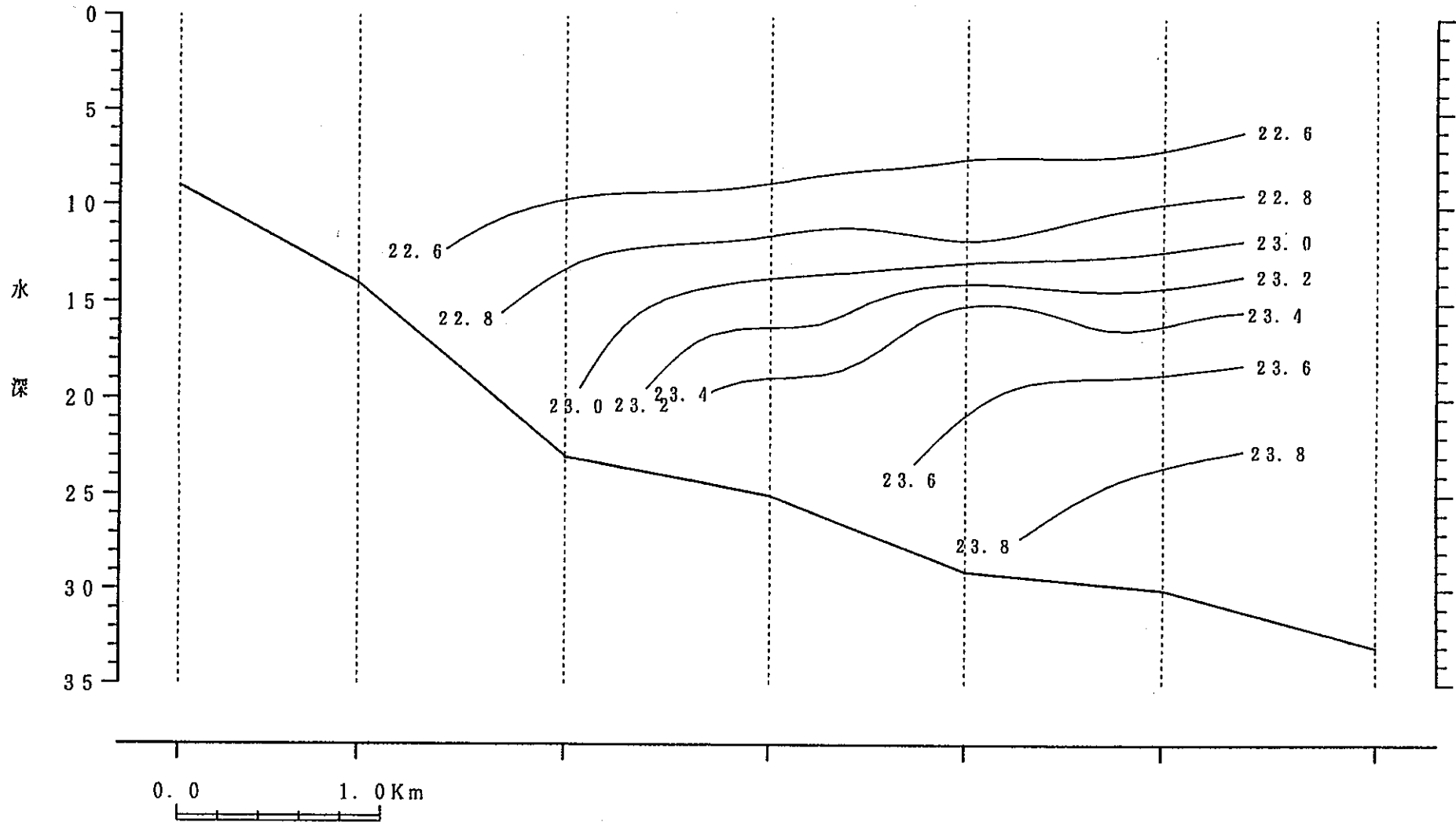
鉛直断面図
