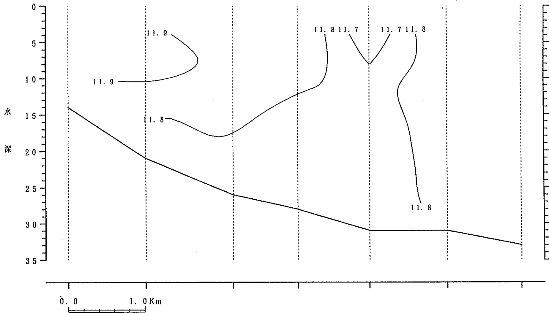
鉛直断面図
