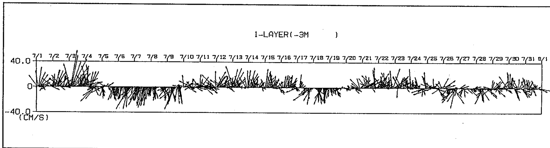
流向・流速ベクトル (海面下3m) 1995 / 7 / 1 0:00 ~ 7 / 31 23:55
