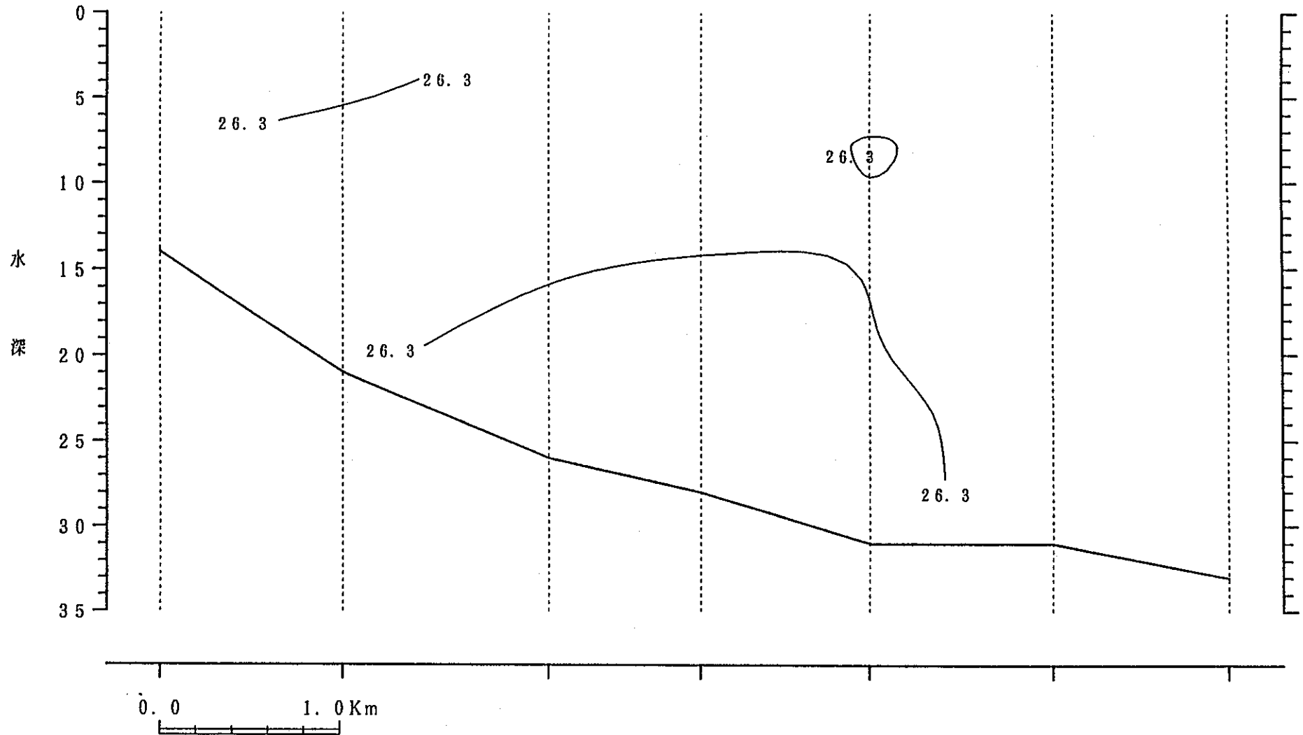
鉛直断面図
