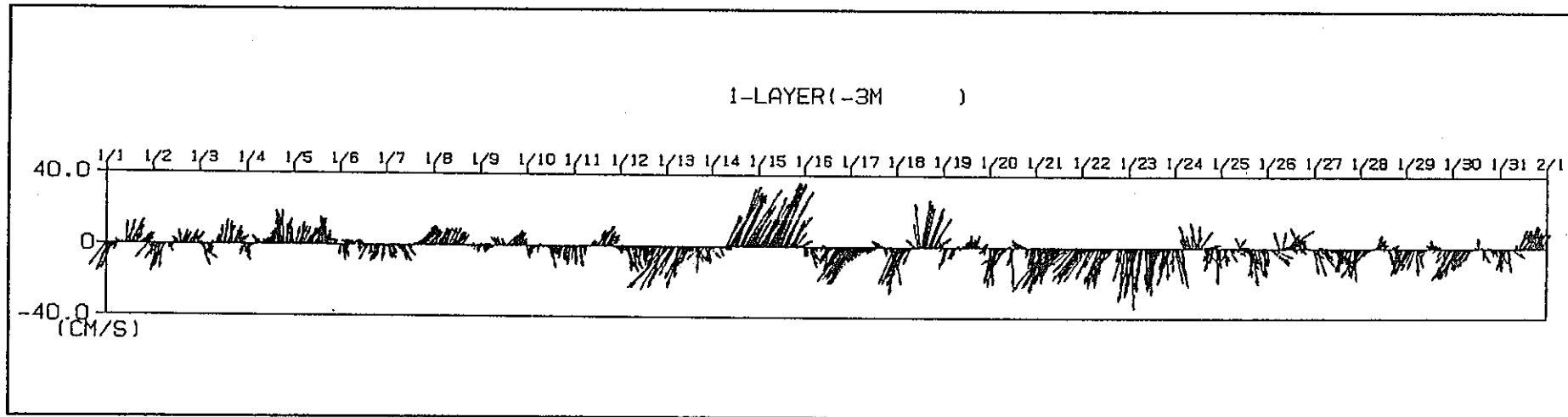
流向・流速ベクトル (海面下3m) 1995 / 1 / 1 0:00 ~ 1 / 31 23:55
