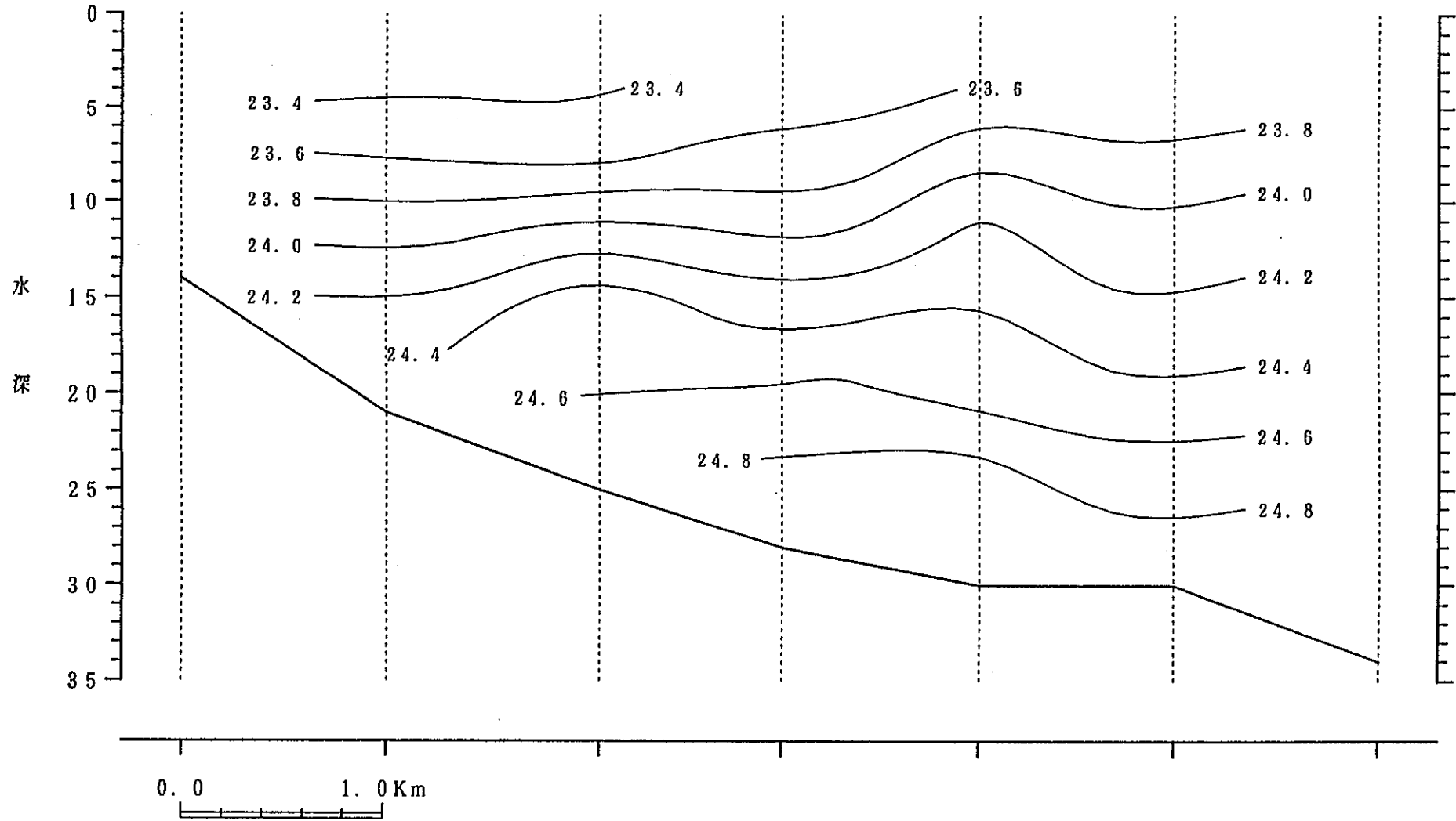
鉛直断面図
