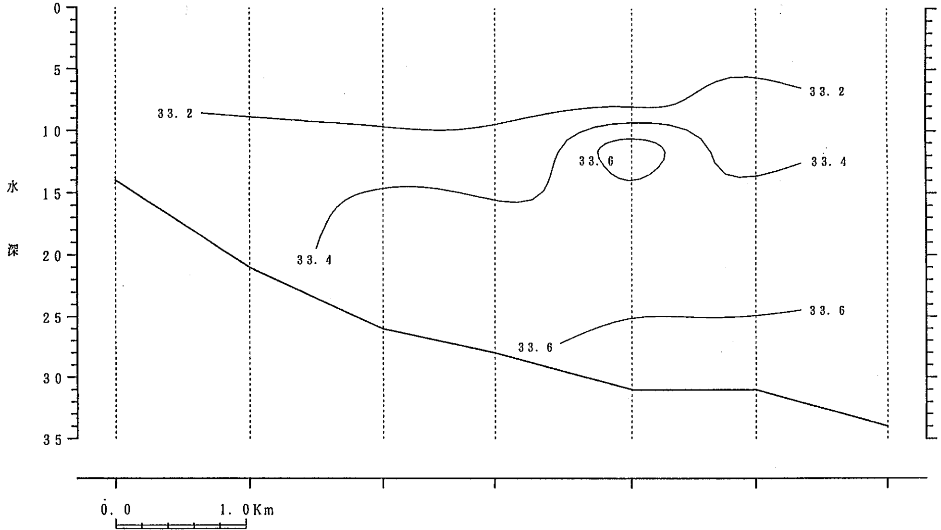
鉛直断面図
