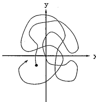
不規則変量 x, y の相関
