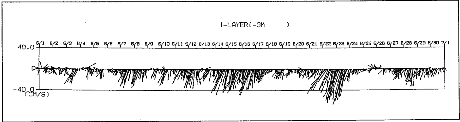
流向・流速ベクトル (海面下3m) 1995 / 6 / 1 0 : 00 ~ 6 / 30 23 : 55
