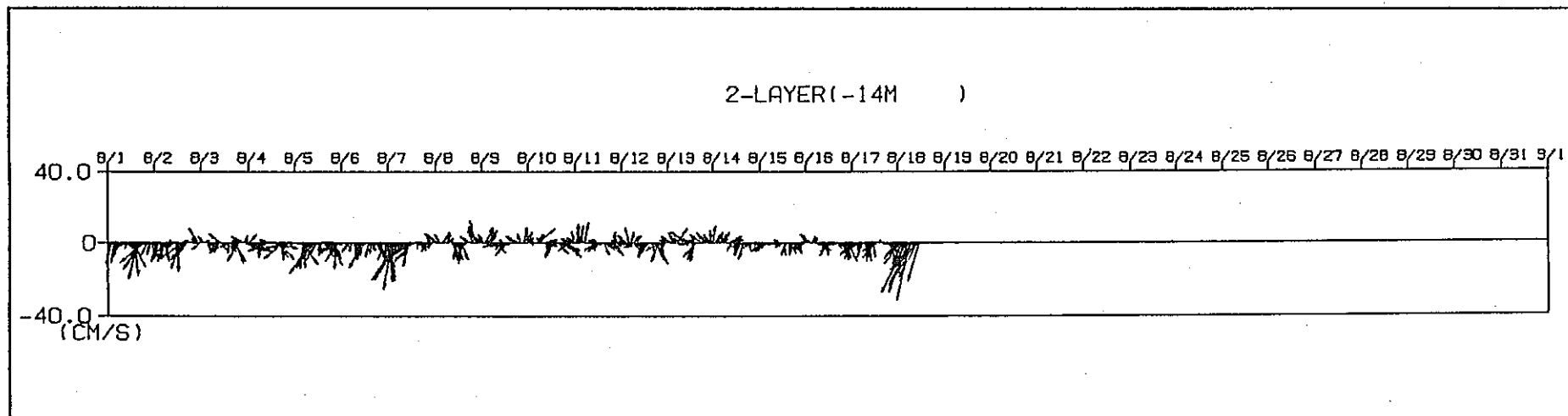
流向・流速ベクトル (海面下14m) 1995 / 8 / 1 0:00 ~ 8 / 31 23:55
