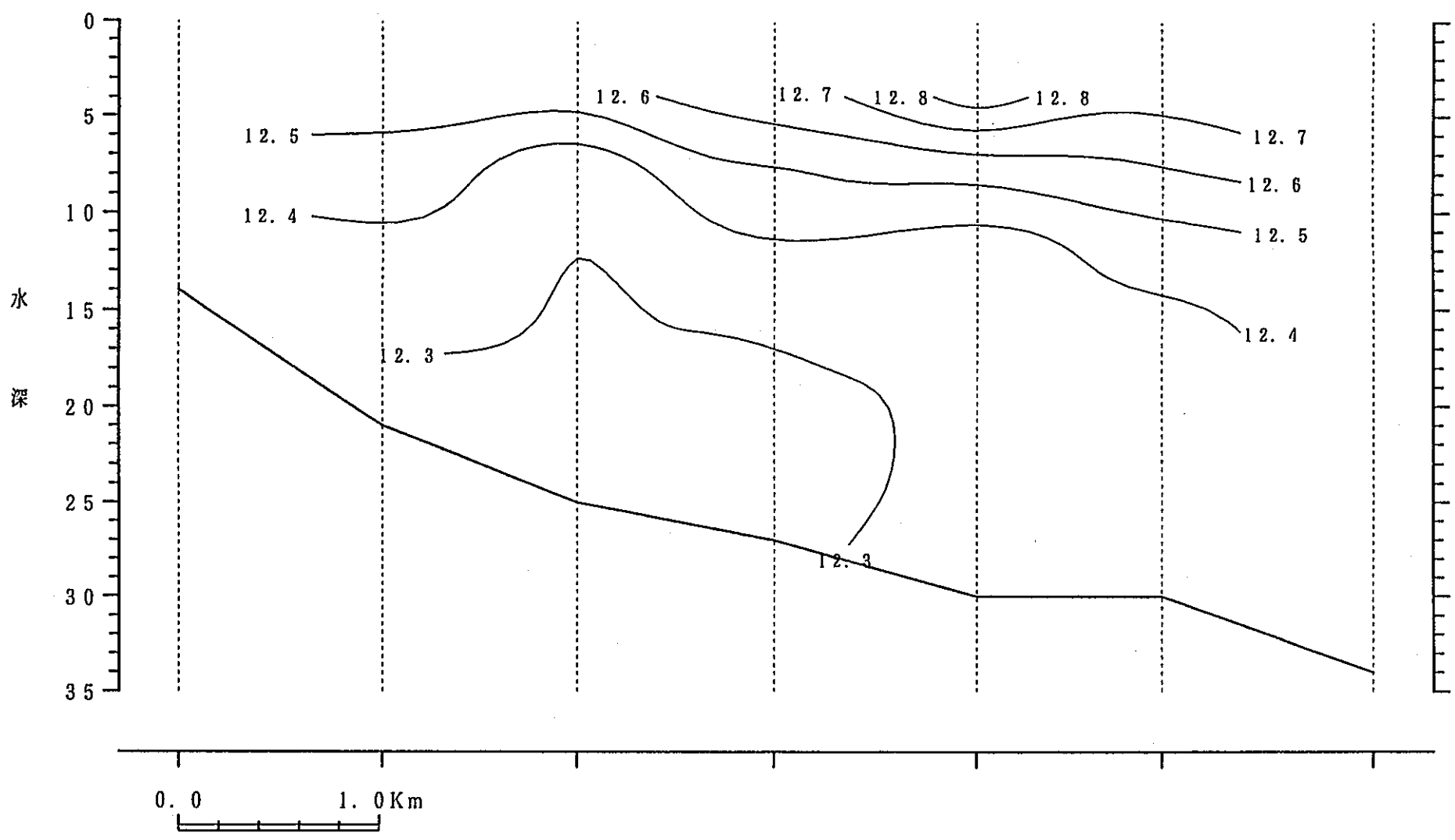
鉛直断面図
