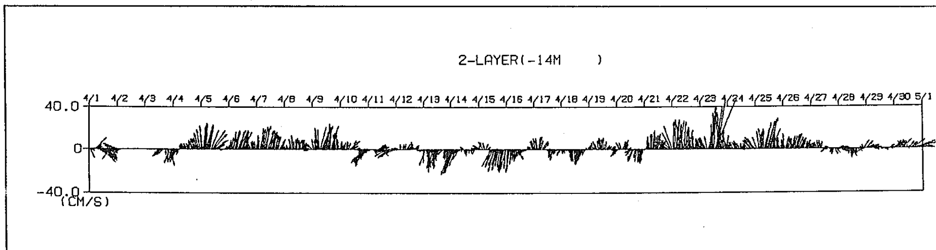
流向・流速ベクトル (海面下14m) 1995 / 4 / 1 0:00 ~ 4 / 30 23:55
