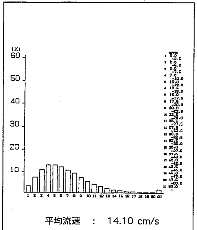
夏季流速分布 (海面下3m)
