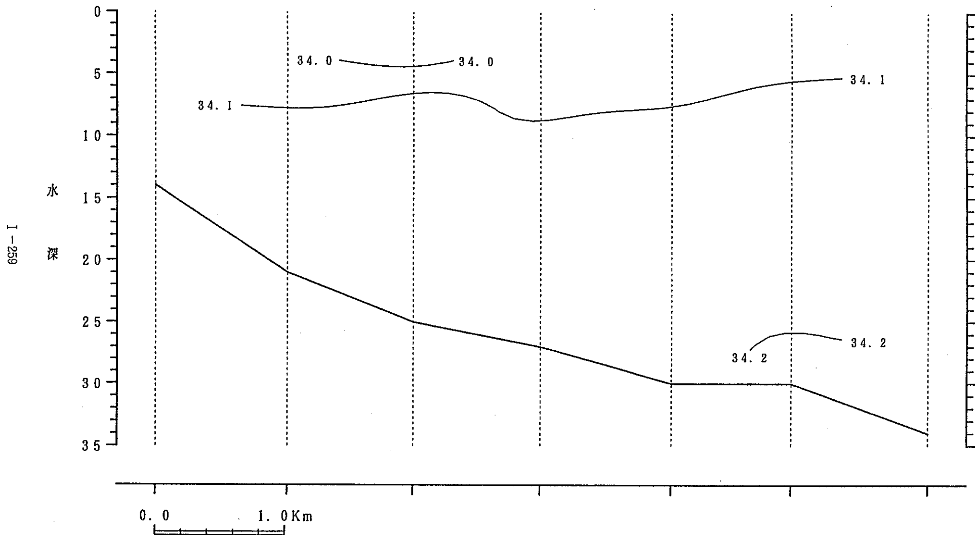
鉛直断面図
