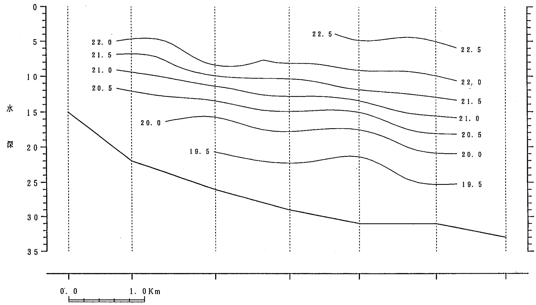
鉛直断面図
