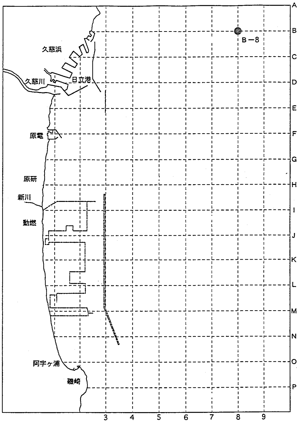
図 II-7.1-2 海水中Pu、Amの物理形態調査に係る試料（海水）採取位置
