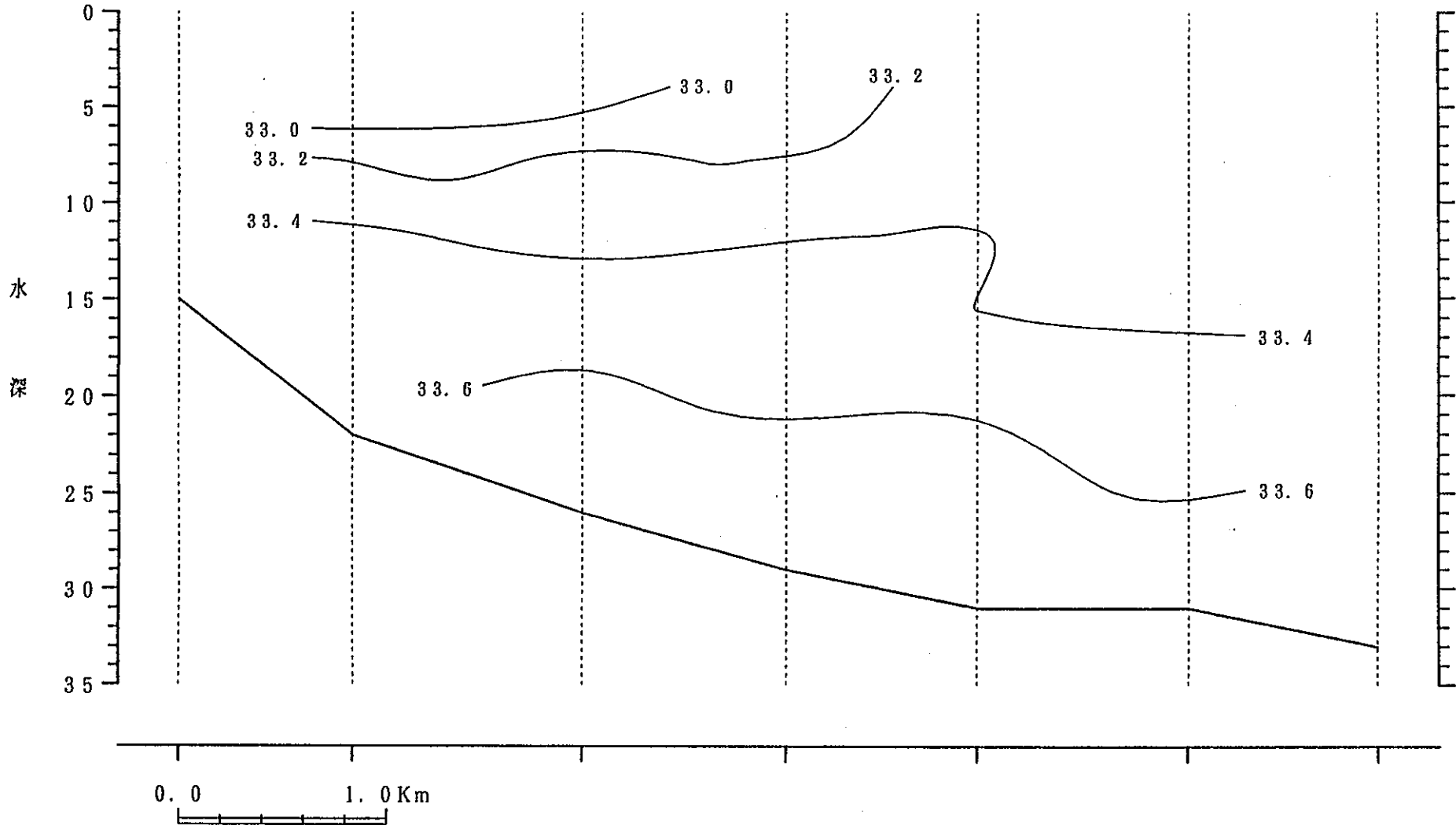
鉛直断面図
