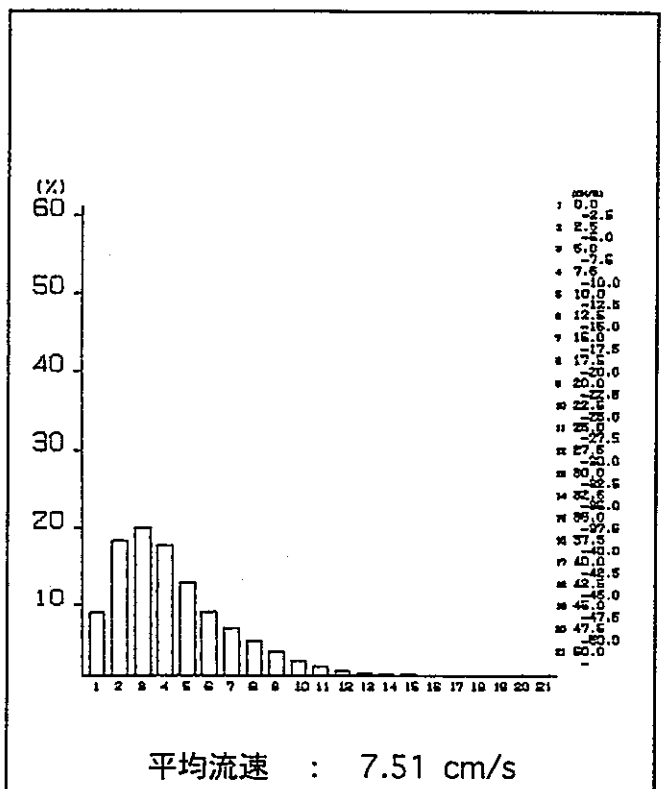
冬季流速分布 (海面下3m)
