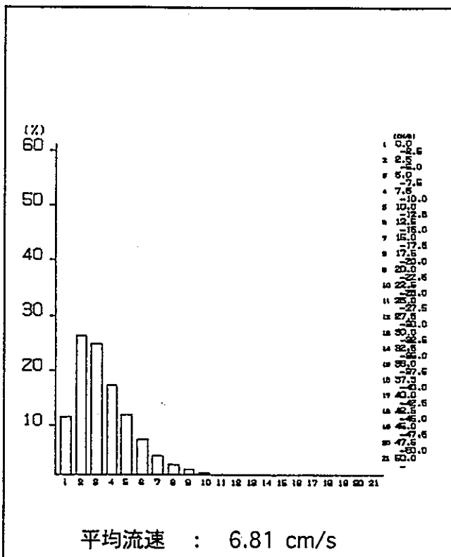
春季流速分布 (海面下14m) 1995/3/1 0:00 ~ 5/31 23:55
