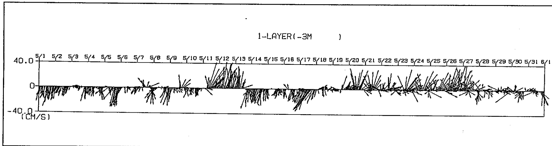
流向・流速ベクトル (海面下3m) 1995 / 5 / 1 0:00 ~ 5 / 31 23:55
