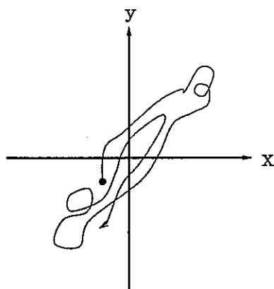
不規則変量 x, y の相関
