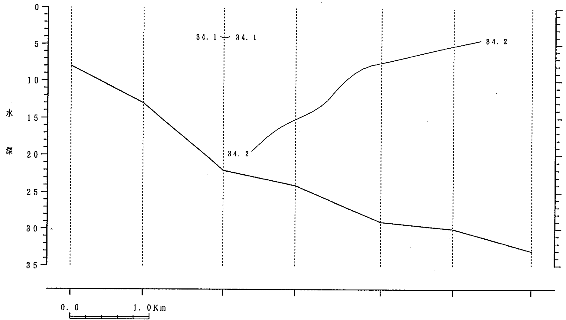
鉛直断面図
