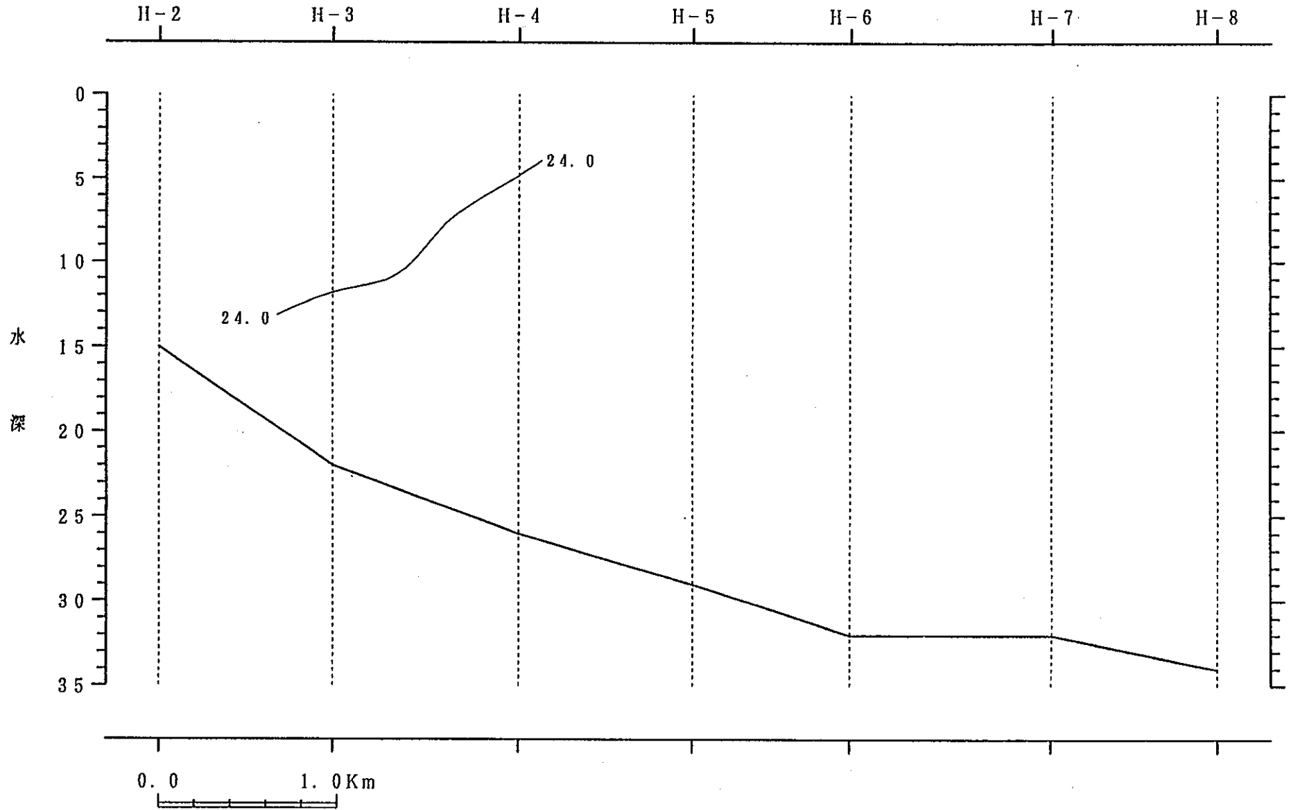
鉛直断面図
