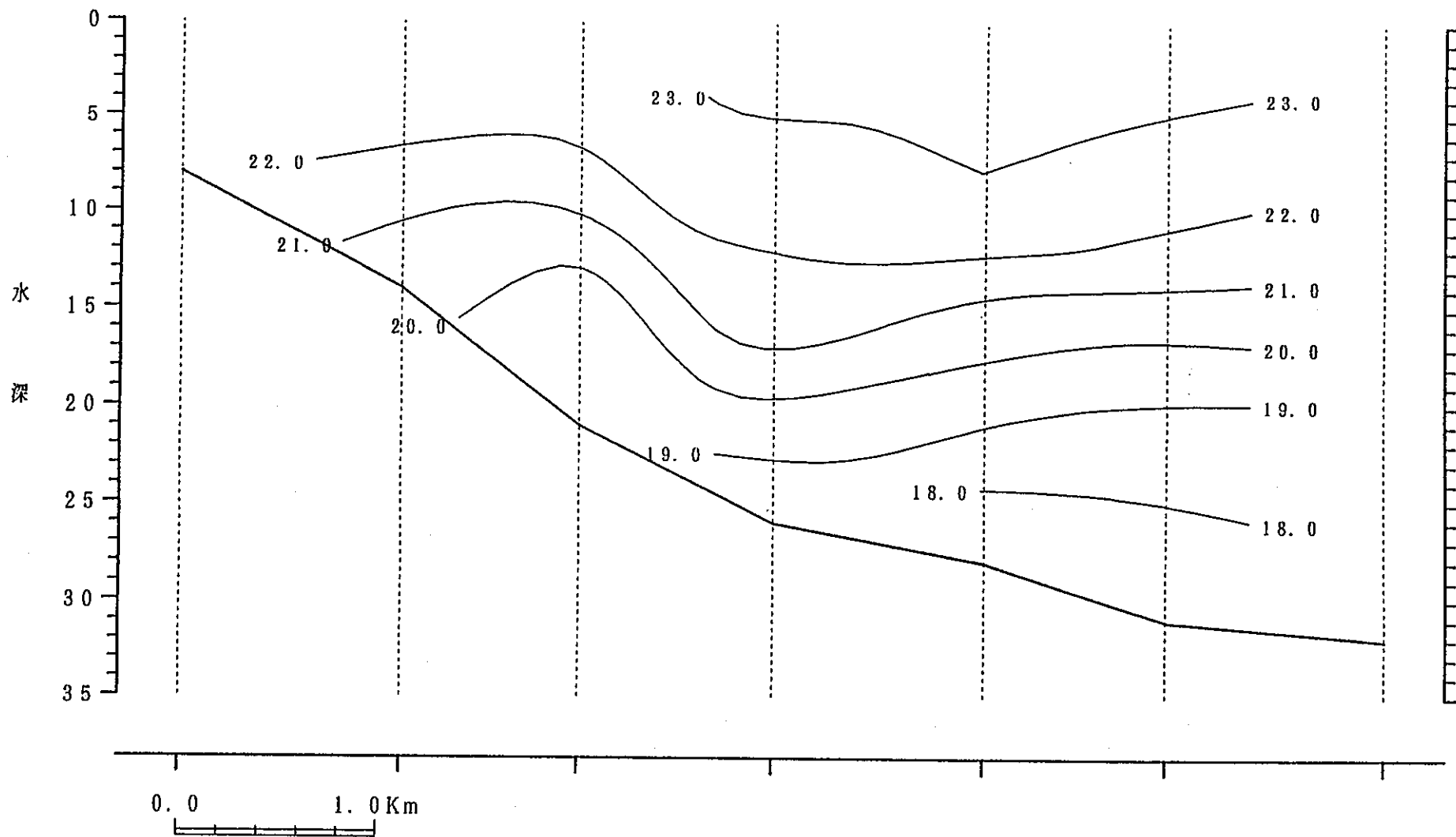
鉛直断面図
