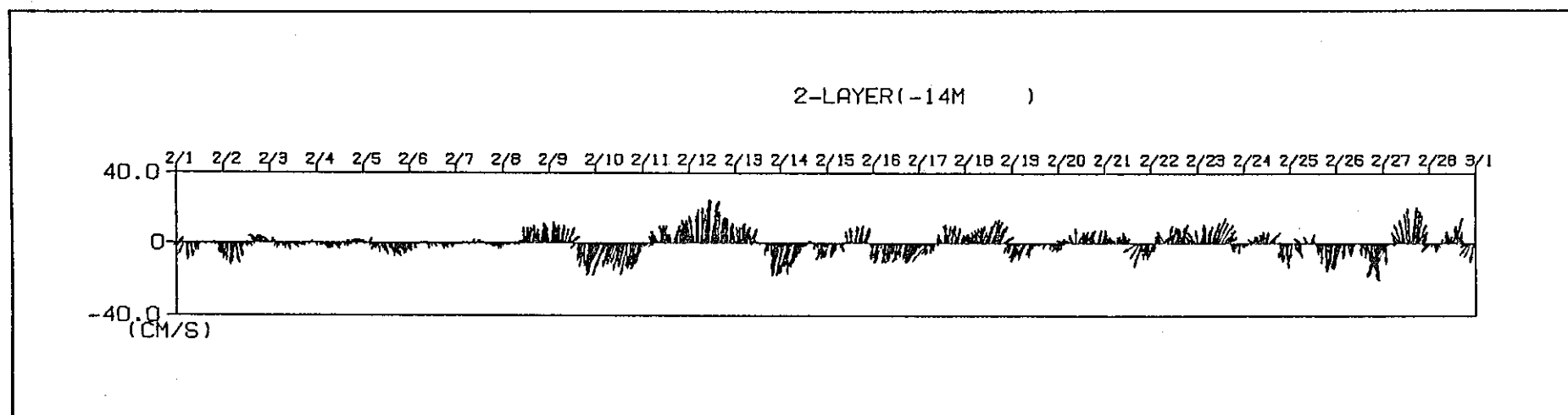
流向・流速ベクトル (海面下14m) 1995 / 2 / 1 0:00 ~ 2 / 28 23:55
