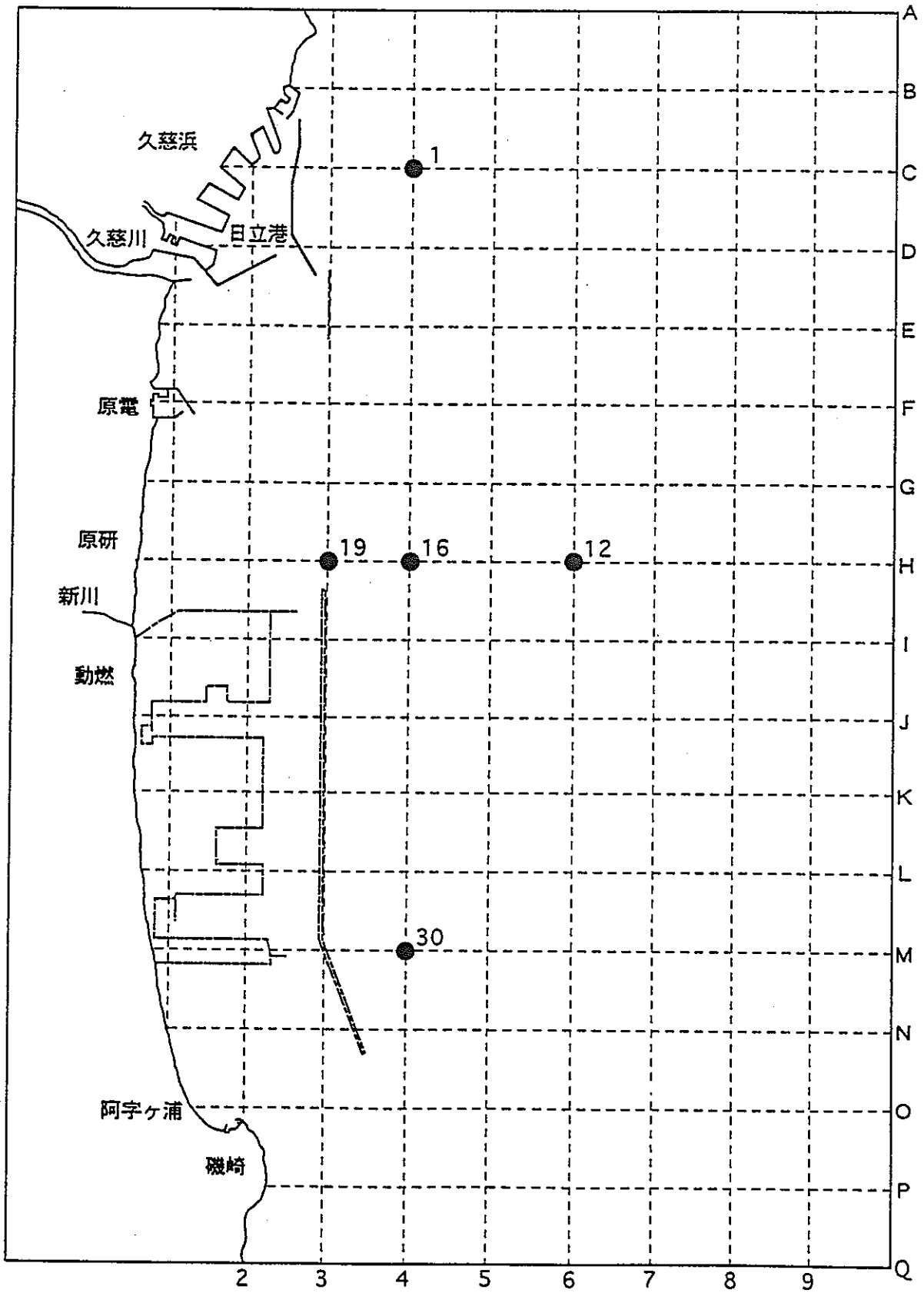
図 II-7.3-2 炭素 (C-14) 測定用の試料 (海水) 採取位置
