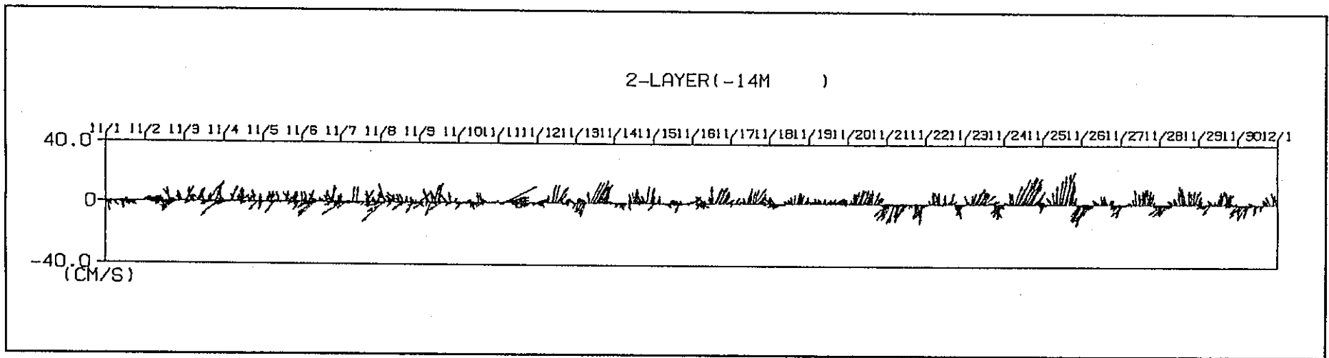
流向・流速ベクトル (海面下14m) 1995 / 11 / 1 0:00 ~ 11 / 31 23:55
