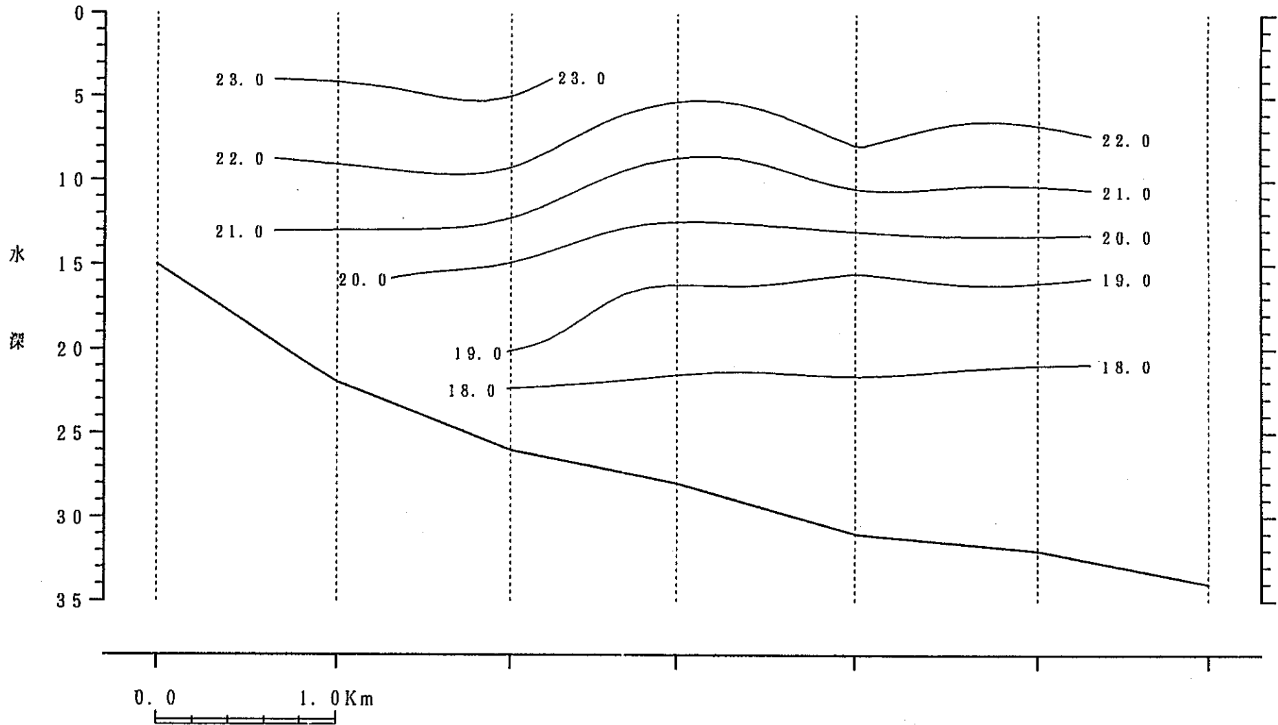
鉛直断面図
